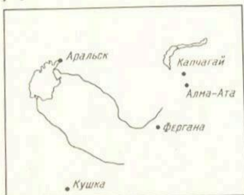
Рис. 14. Территория, данные о минерализации осадков на которой использовались при анализе
