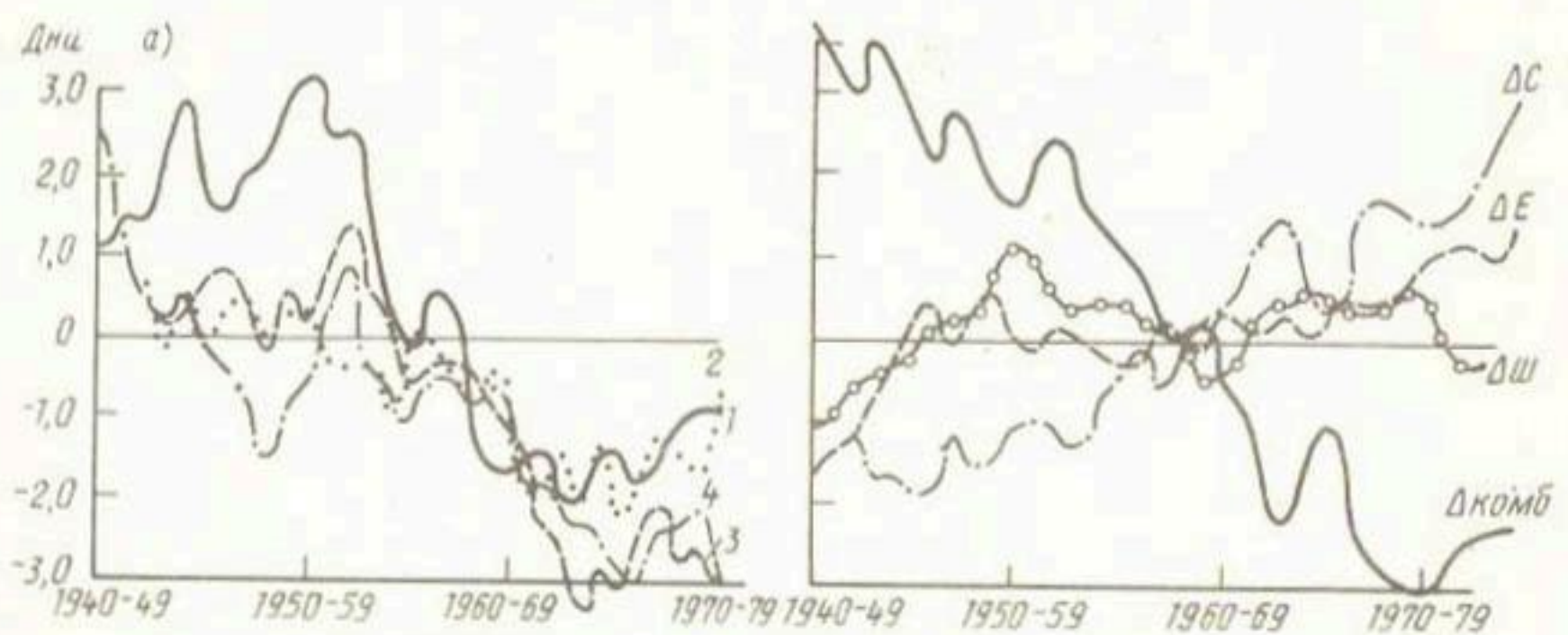
Рис. 28. 10-летние скользящие средние отклонений от нормы числа годовой ход циркуля I - Тамды, 2 - Уялы,
