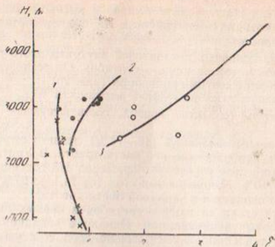
Рис. 27. Зависимость величины \delta от средневзвешенной высоты: 1 — западная часть; 2 — Уратыубинская котловина; 3 — восточная часть.
