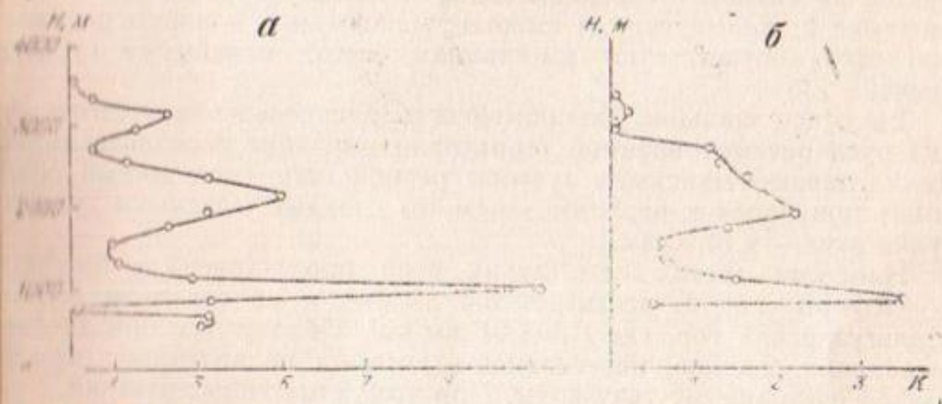
Рис. 14. Распределение показателя полноты родниковой сети по высоте. Бассейны рек Исфары (а) и Ходжабакиргана (б).
