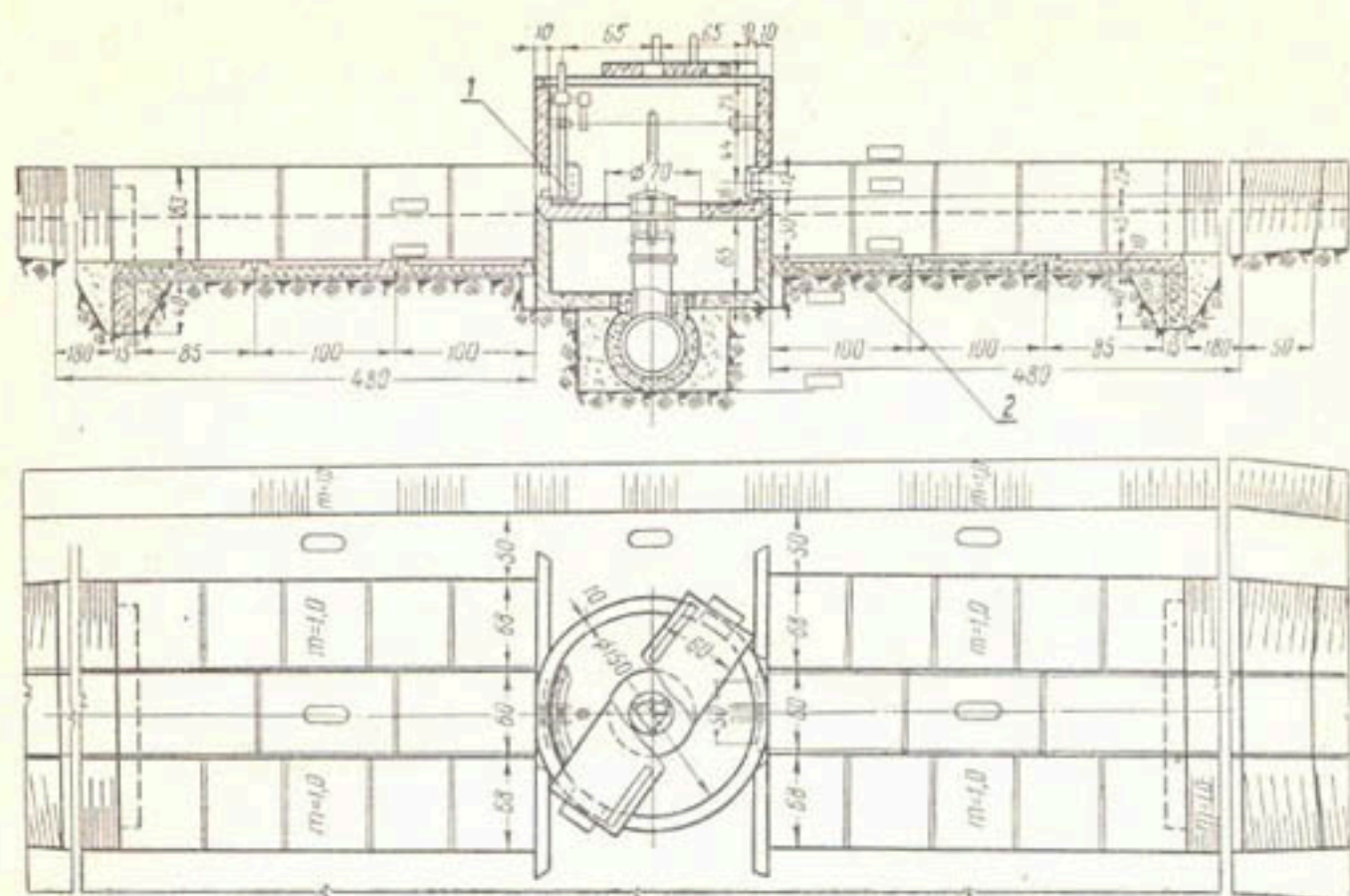
Рис 45. Двухсторонний водовыпуск с тарельчатым клапаном из трубопровода в открытые оросители:
