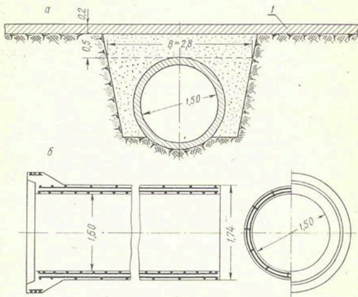
Рис. 105. Расчетная схема проезда (а) и конструктивная схема трубы (б):
