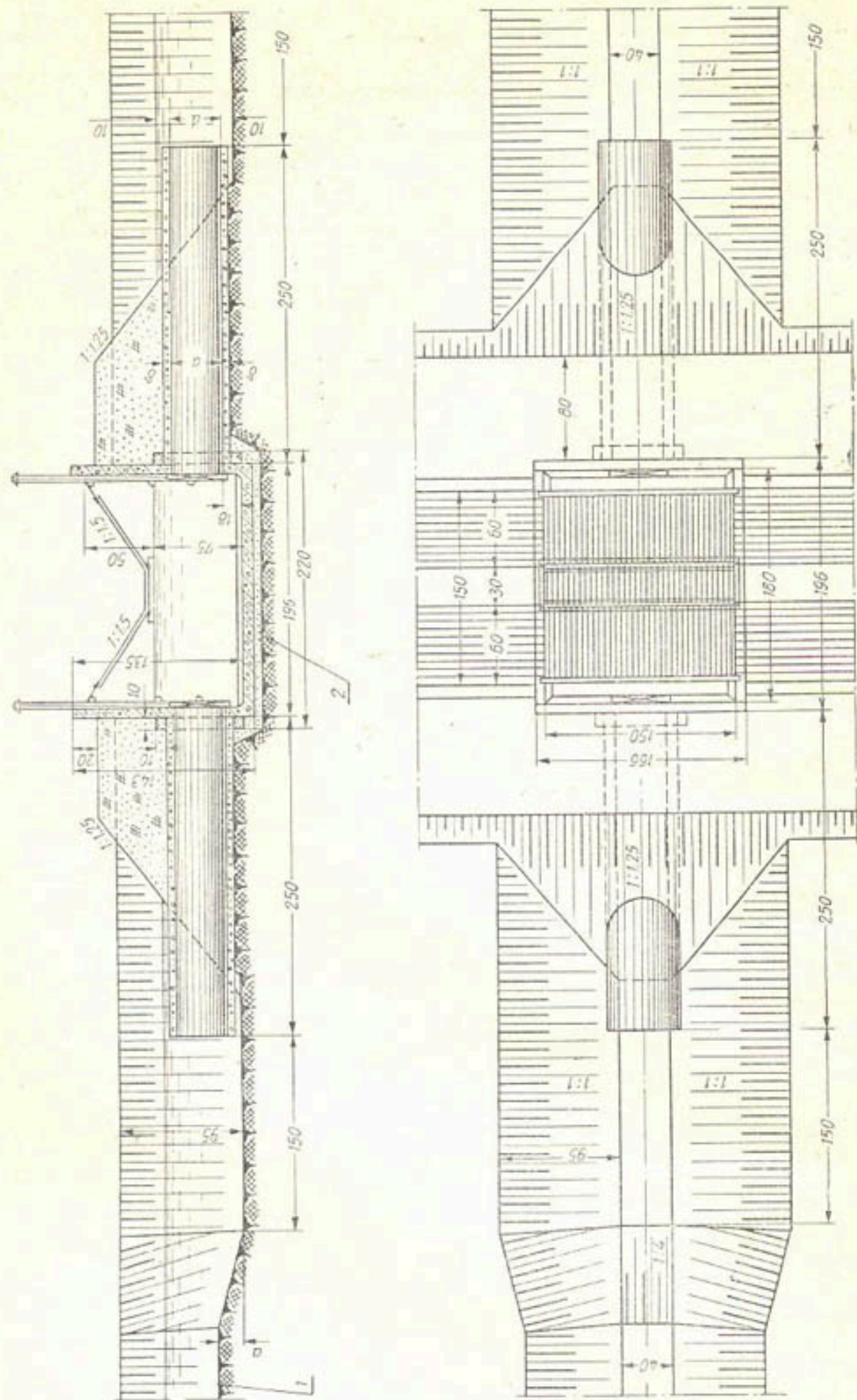
Рис. 5. Водовыпуск во временный ороситель: 1 — временный ороситель; 2 — гравийная подготовка.
