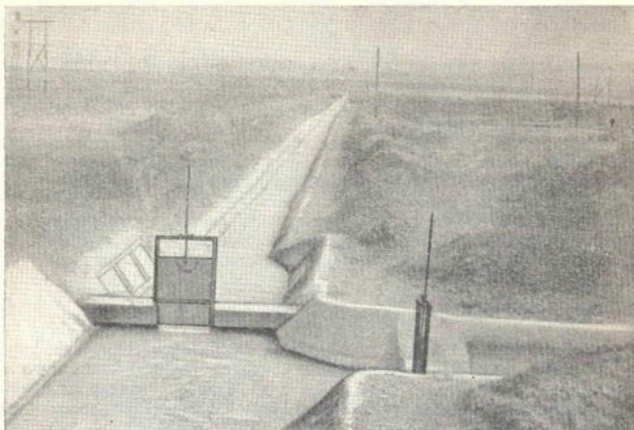
Рис. 32. Узел сооружений — двойник, состоящий из открытого регулятора и перегородаживающего сооружения.
