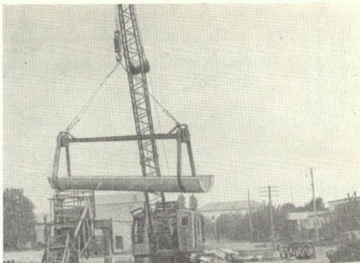
Рис. 125. Захватная траверса для загрузки лотков.
