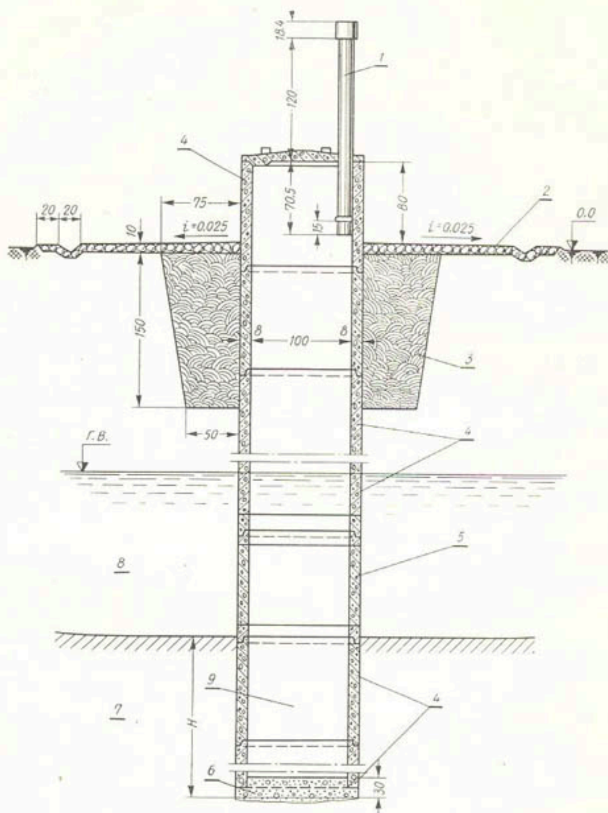
Рис. 83. Шахтный колодец из сборного железобетона:
