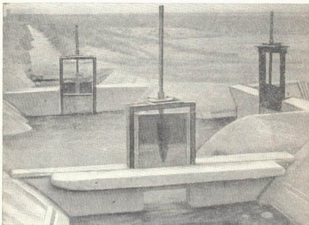
Рис. 33. Узел сооружений — тройник, состоящий из двух открытых регуляторов и перегородаживающего сооружения.
