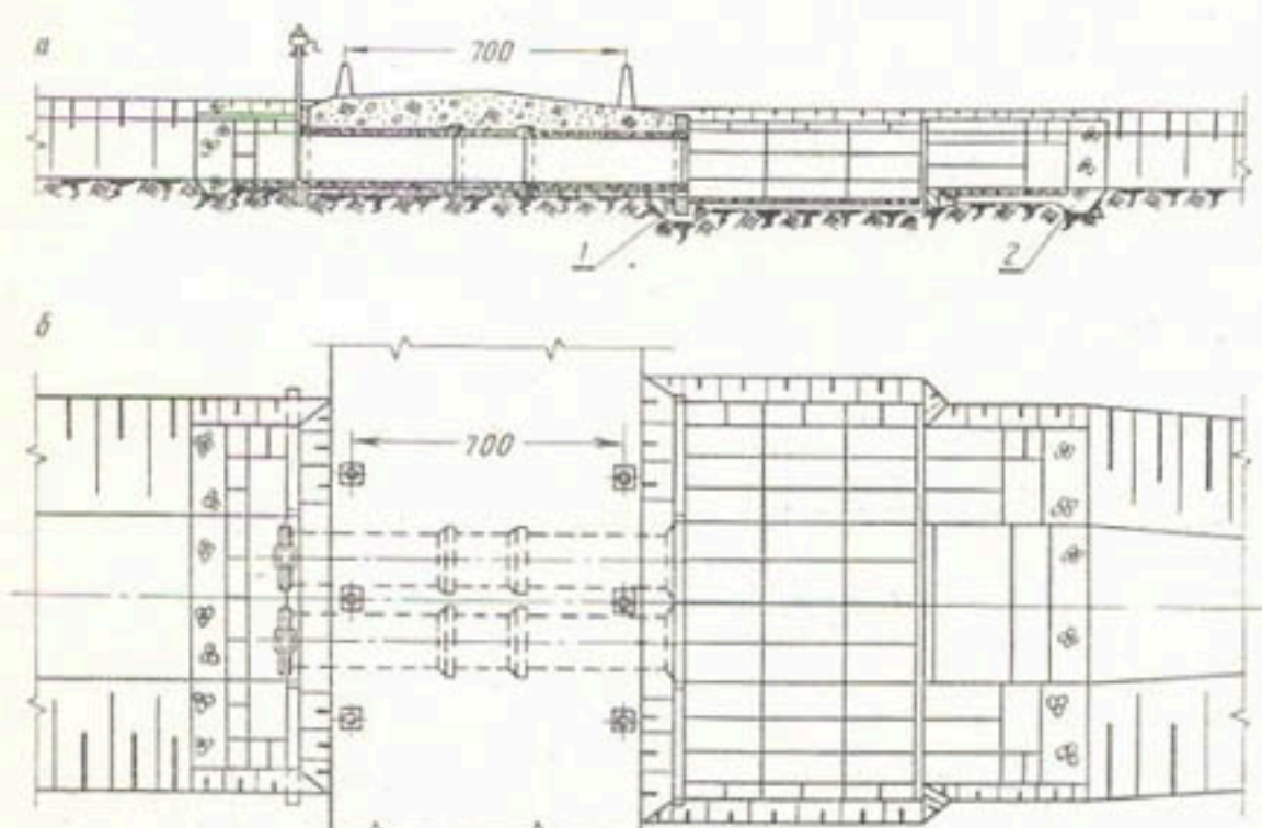
Рис. 77. Трубчатый шлюз-регулятор:
