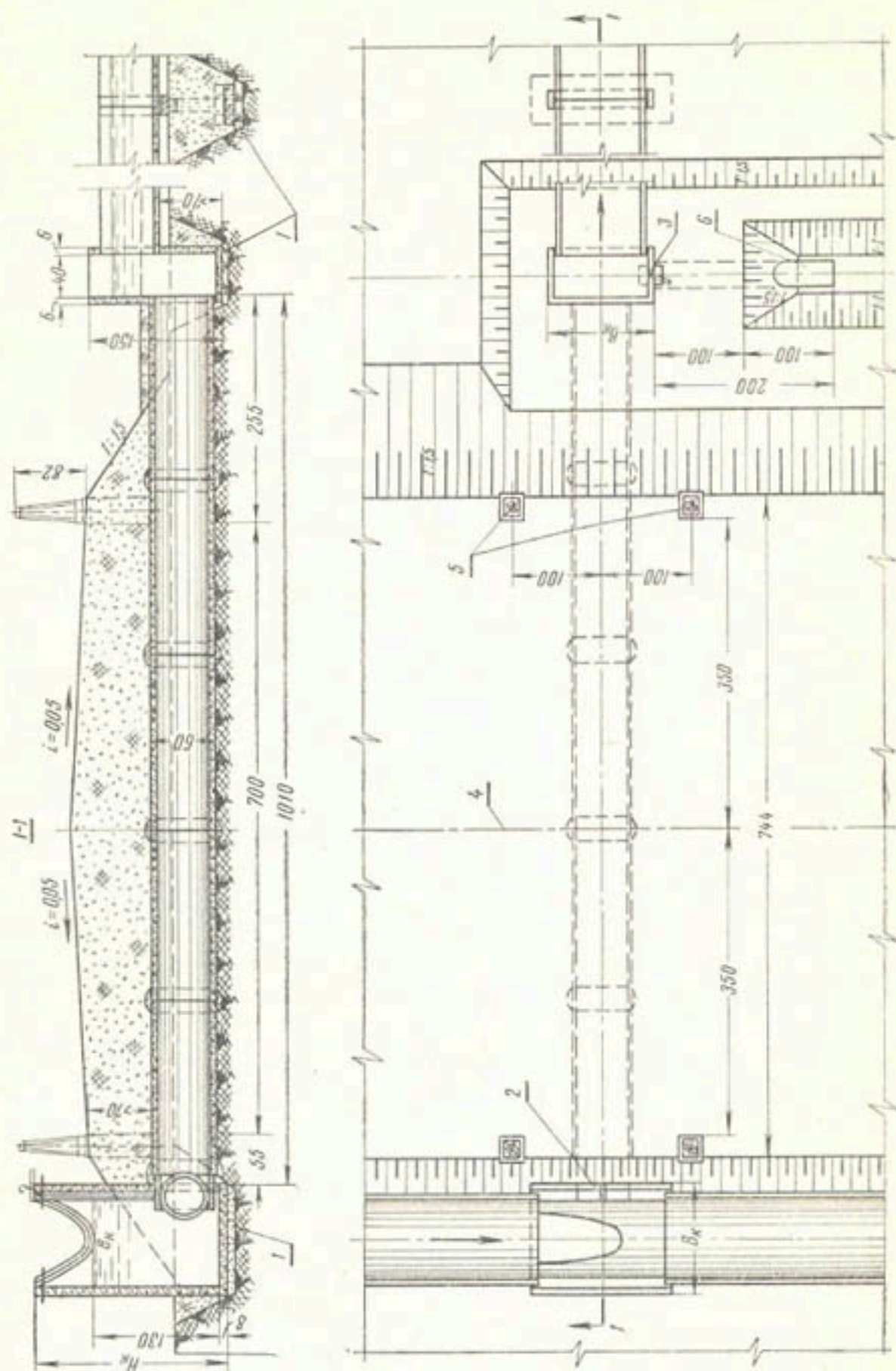
Рис. 60. Вододелитель с перепадом и водовыпуском для скоростей больше критических:
