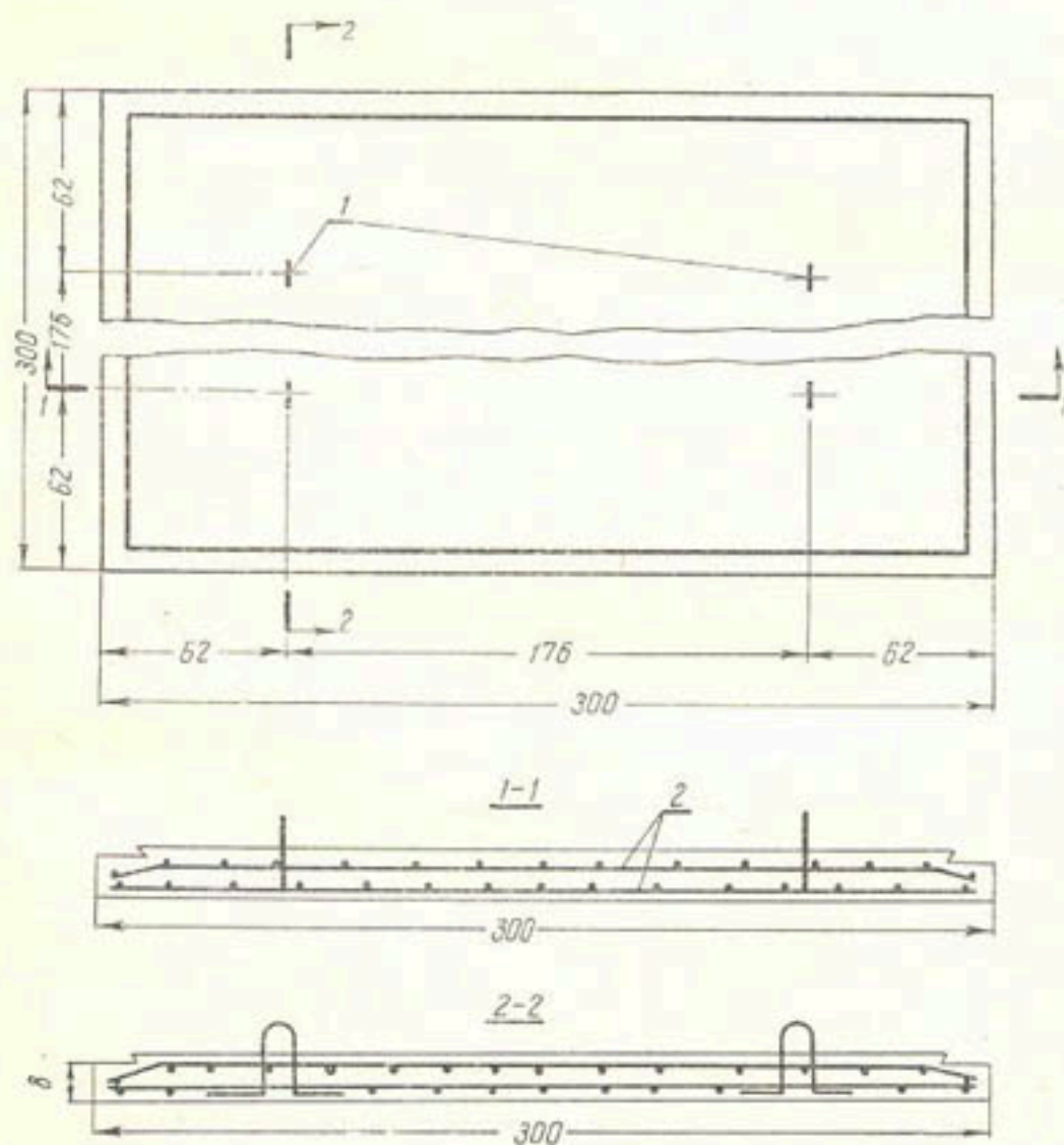
Рис. 36. Железобетонная плита для облицовки канала Северский Донец — Донбасс:
