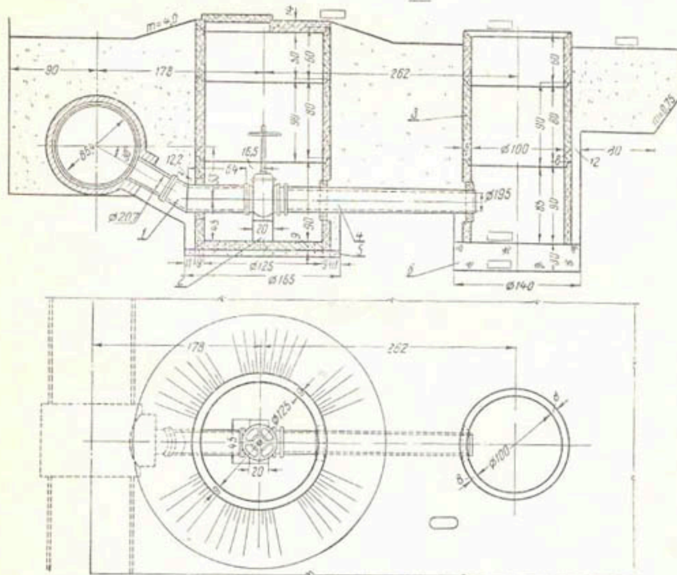
Рис. 46. Смотровой колодец и колодец промежуточного сброса воды из трубопровода:
