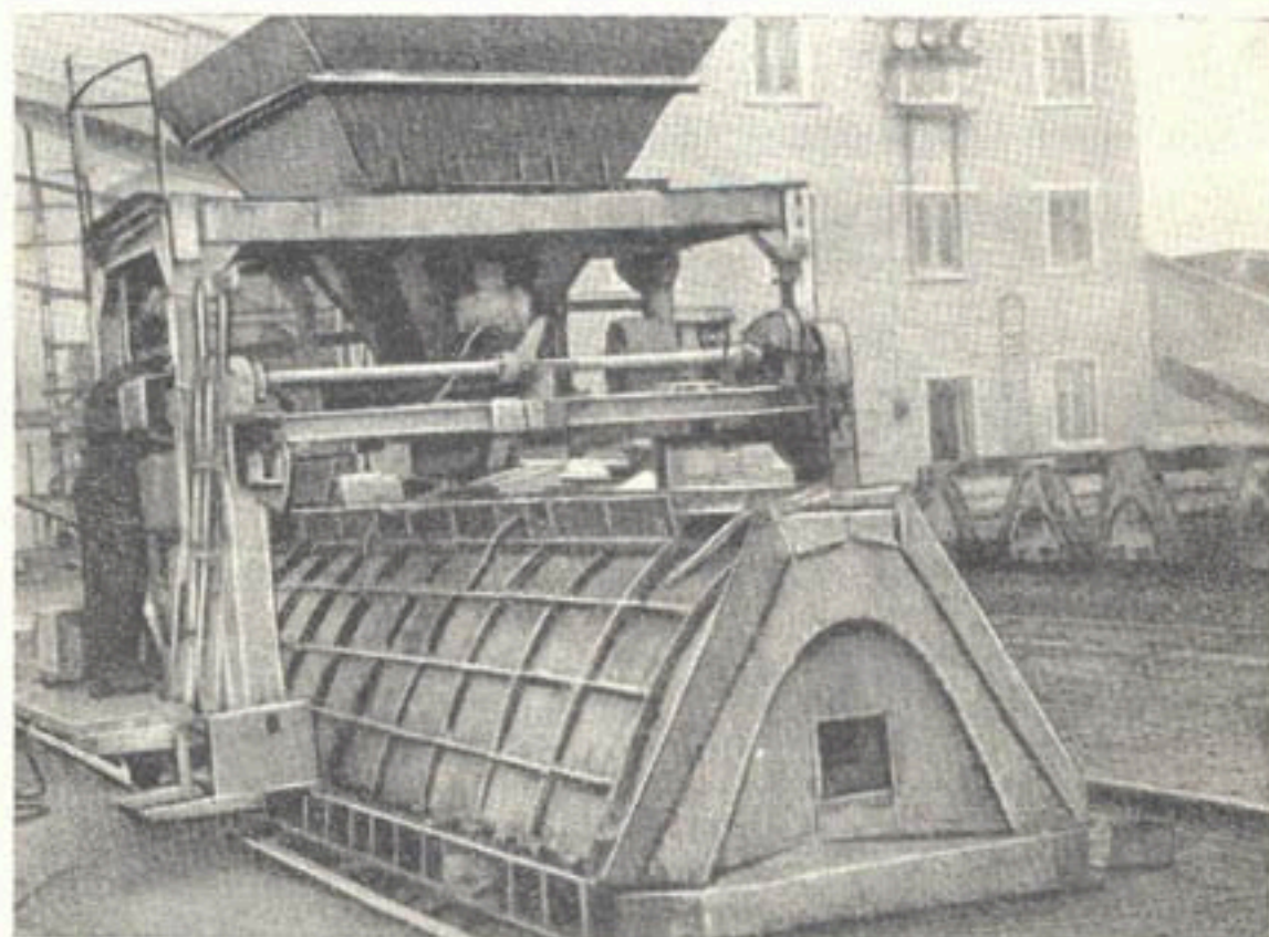
Рис. 116. Формовка лотков глубиной 1 м на виброплощадке.
