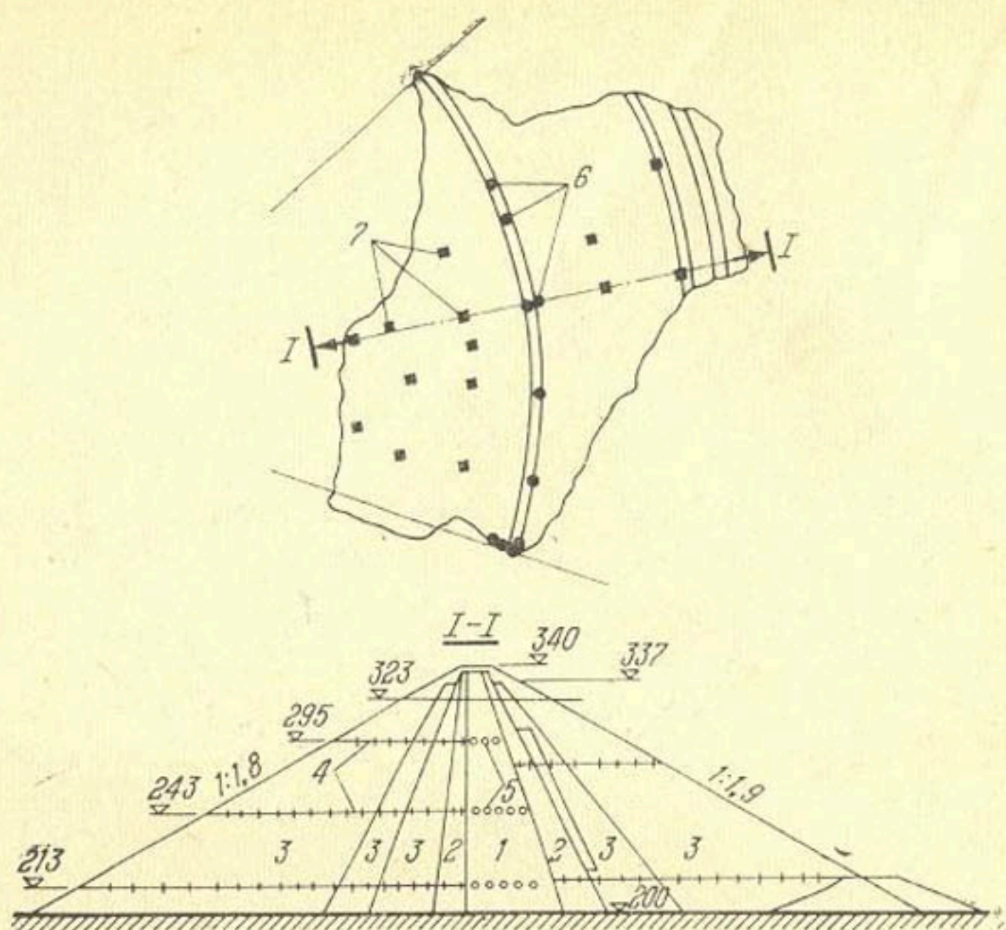
Рис. VI.6. Схемы расположения контрольно-измерительной аппаратуры в поперечном сечении и плане плотины Картерс
