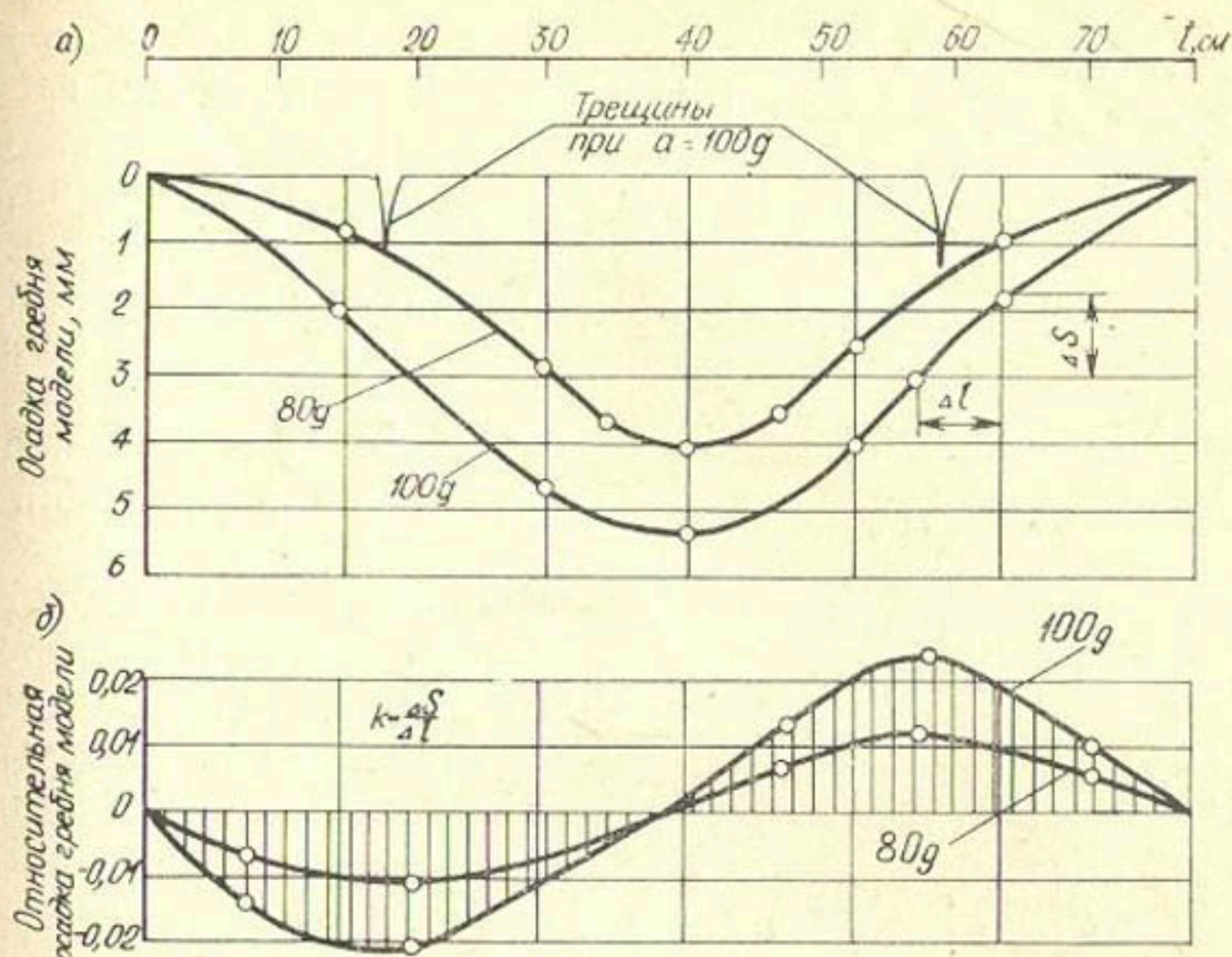
Рис. IV.1. Эпюры вертикальных перемещений (а) и относительных осадок (б) гребня модели при уклоне бортов каньона \alpha = 40^\circ
