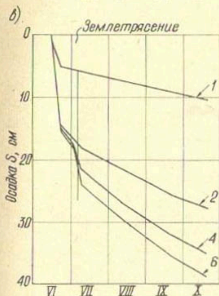
Рис. I.13. График наполнения водохранилища (а), осадки точек ядра (б), верхней (в) и нижней (г) призм плотины Инфернильо
