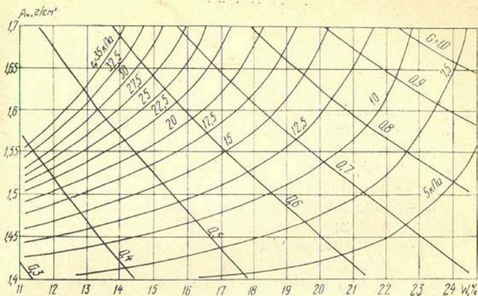
Рис. V.9. Линии равных сцеплений на разрыв c_p в зависимости от \rho_{sk} , W , G для гиссаракского суглинка
