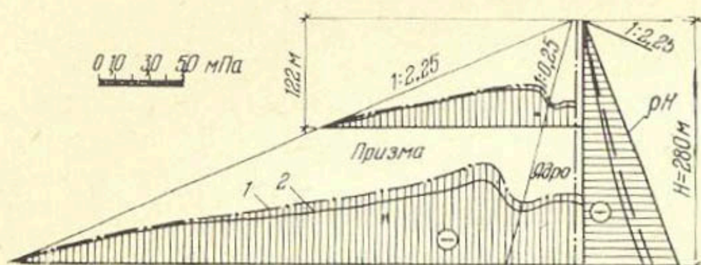
Рис. III.12. Распределение вертикальных напряжений \sigma_y в поперечном сечении плотины с ядром при E_{\text{пр}} > E_{\text{я}} для условий плоской задачи 1 и пространственной задачи 2
