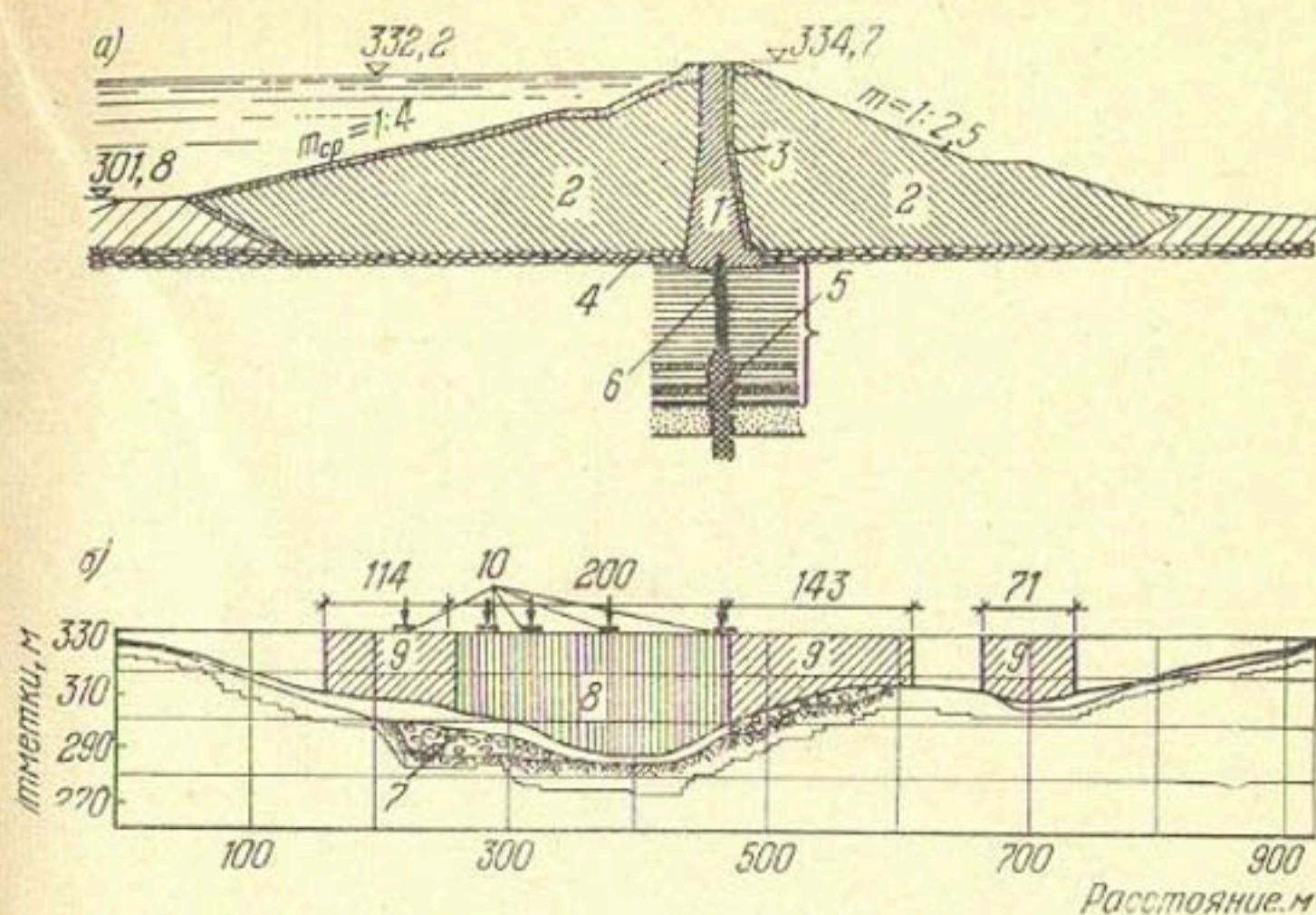
Рис. I.7. Плотина Болдерхед
