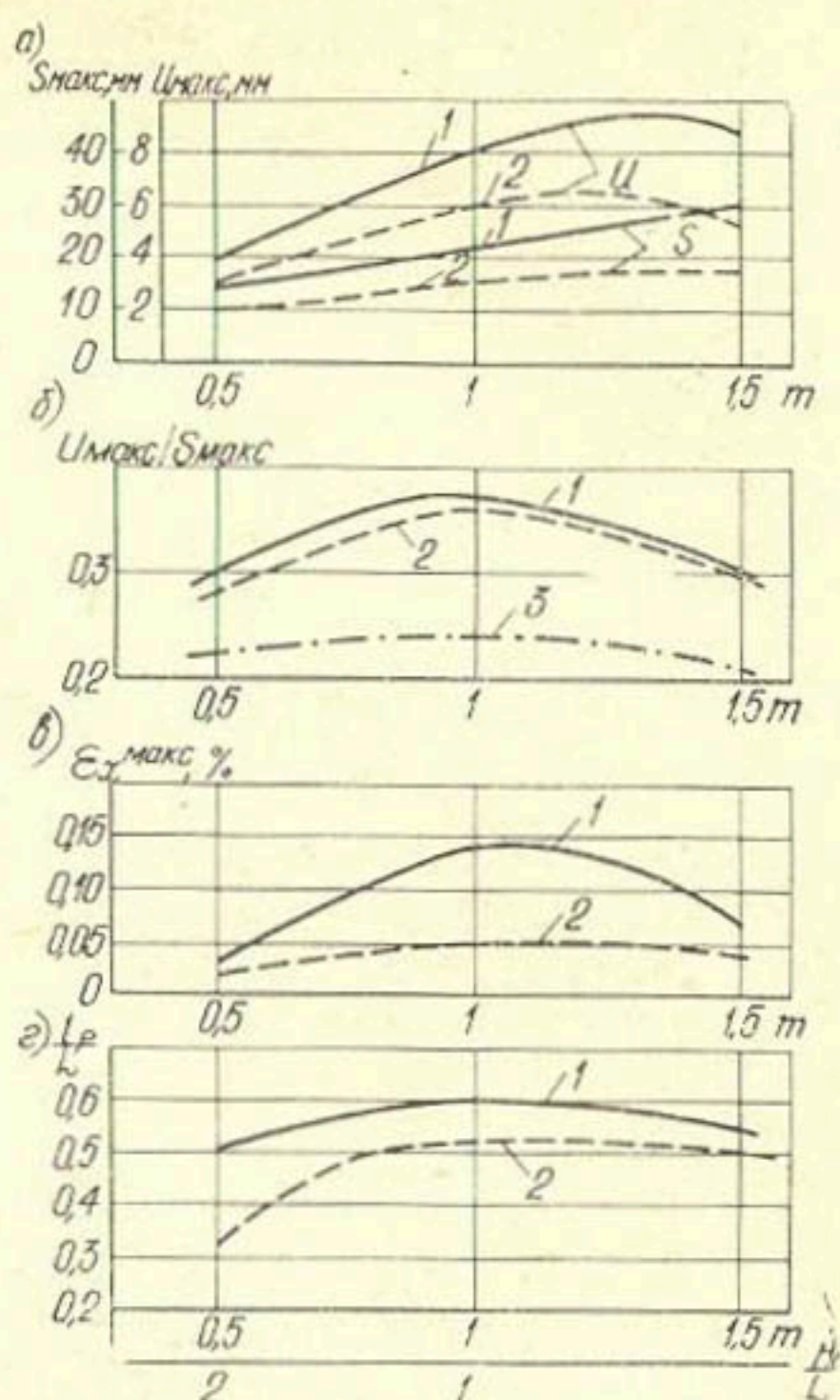
Рис. IV.6. Графики изменения максимальных значений вертикальных и горизонтальных перемещений (а), их отношения \frac{u_{\max}}{S_{\max}} (б), относительных деформаций (в) и относительных размеров зон растяжения на гребне (г) в зависимости от заложения бортов m 1 — \rho_{\text{ск}} = 1,55 \text{ г/см}^3 ; 2 — \rho_{\text{к}} = 1,7 \text{ г/см}^3 ; 3 — расчетная кривая при E = 15 \text{ МПа} , \mu = 0,3
