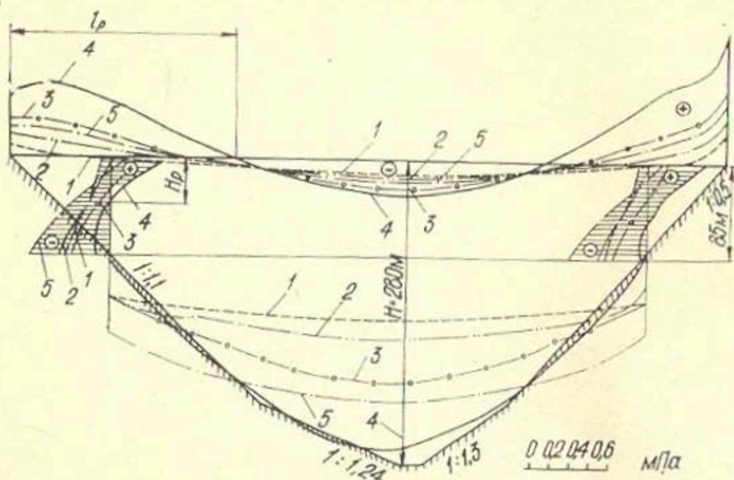
Рис. III.11. Распределение горизонтальных напряжений \sigma_x в продольном сечении ядра плотины при решении пространственной задачи
