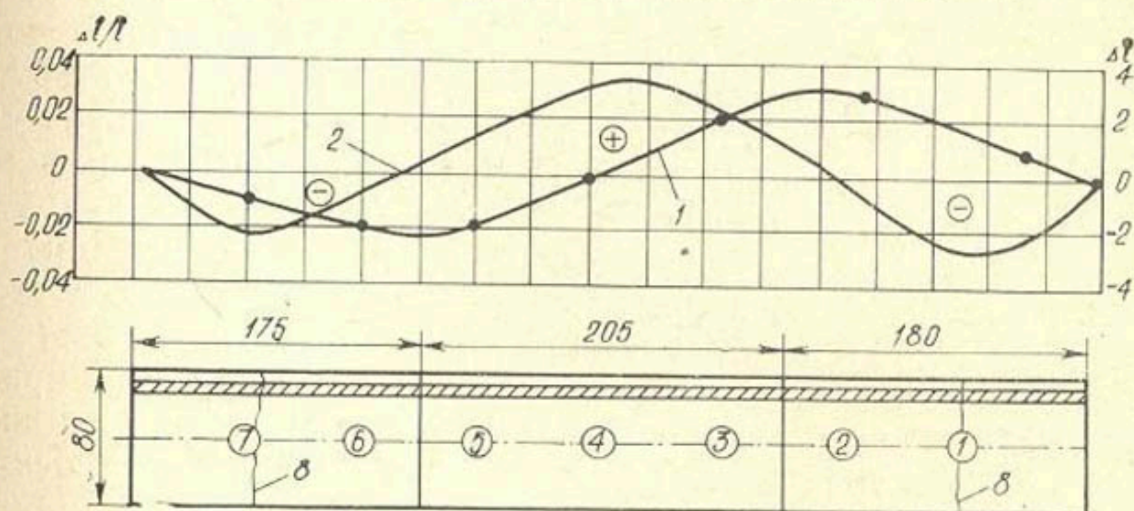
Рис. IV.1. Эпюры вертикальных перемещений (а) и относительных осадок (б) гребня модели при уклоне бортов каньона \alpha = 40^\circ
