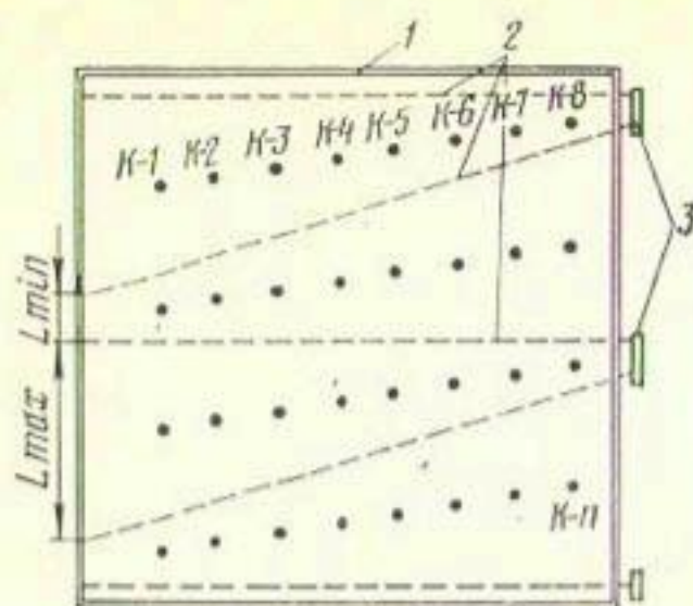
Рис. 5. Схема расположения пробных дрен на участке:
