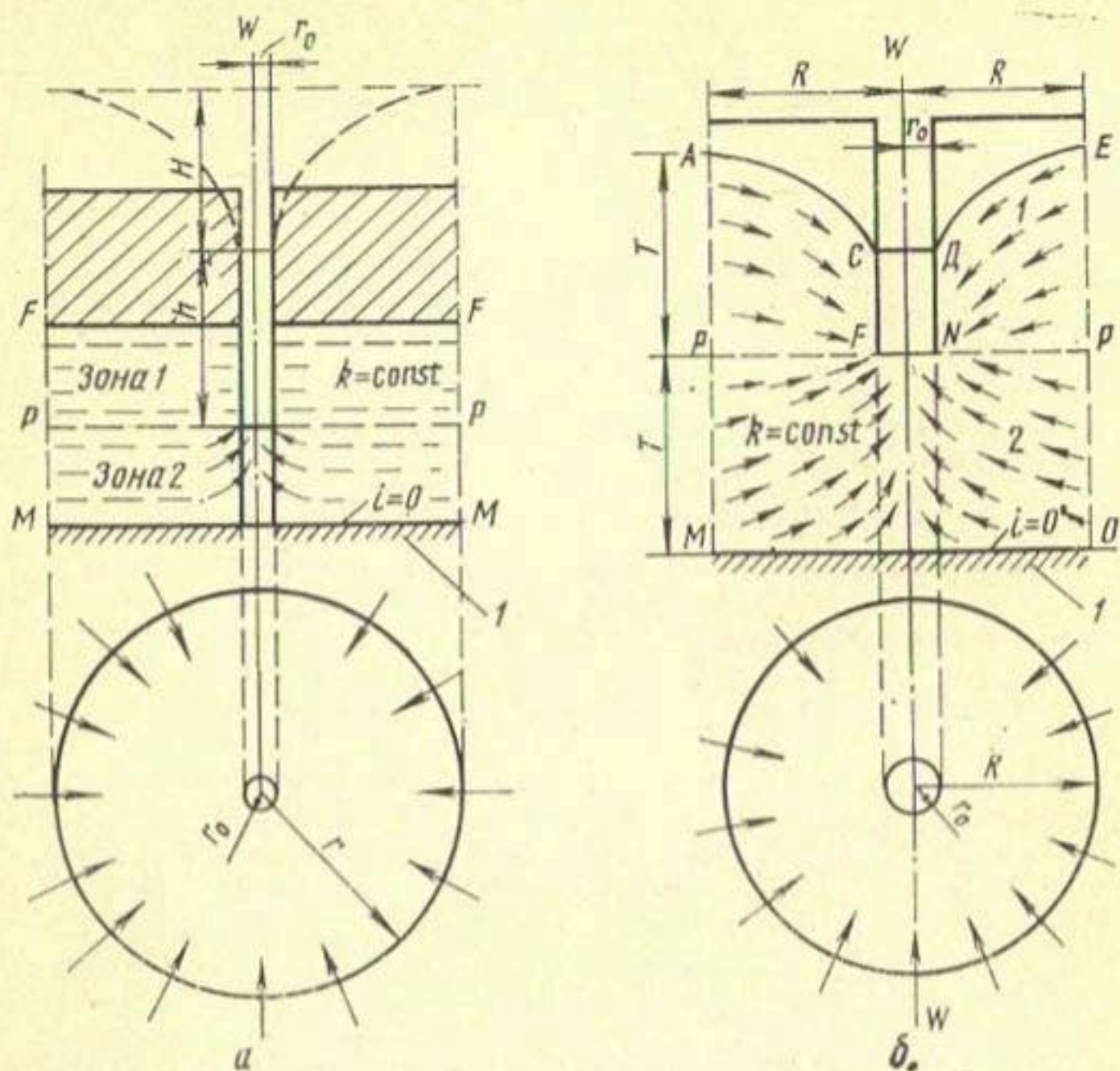
Рис. 1. Схема разбивки на фрагменты напорной (а) и безнапорной (б) области фильтрации.
