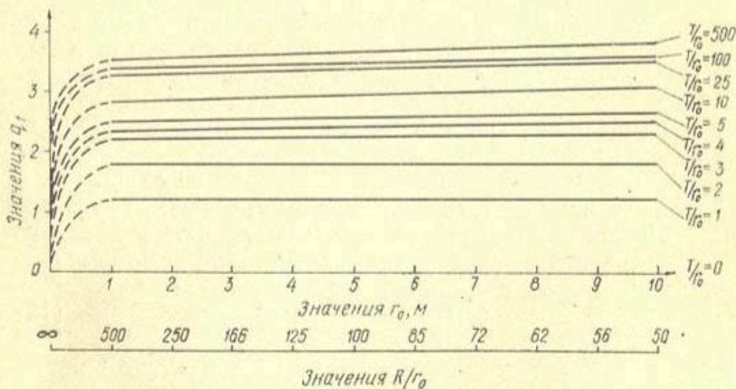
Рис. 13. График изменения расхода q_1 в зависимости от значений r_0 и T при R=500 .
