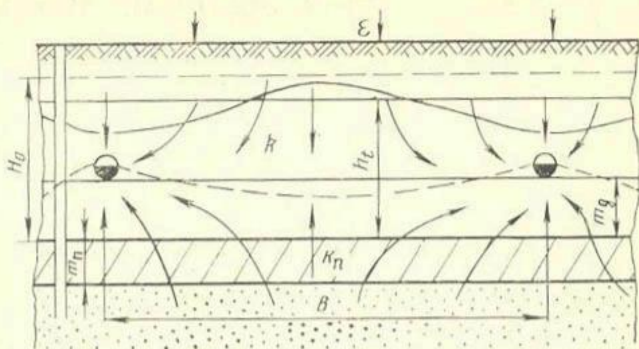
Рис. 1. Схема к расчету динамики уровня грунтовых вод при одновременном напорном и инфильтрационном питании: I — дрена.
