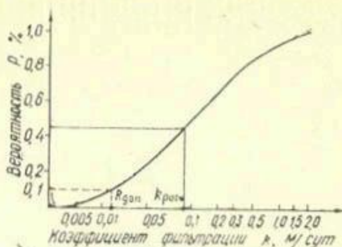
Рис. 2. Интегральное распределение коэффициентов фильтрации средних минеральных грунтов.
