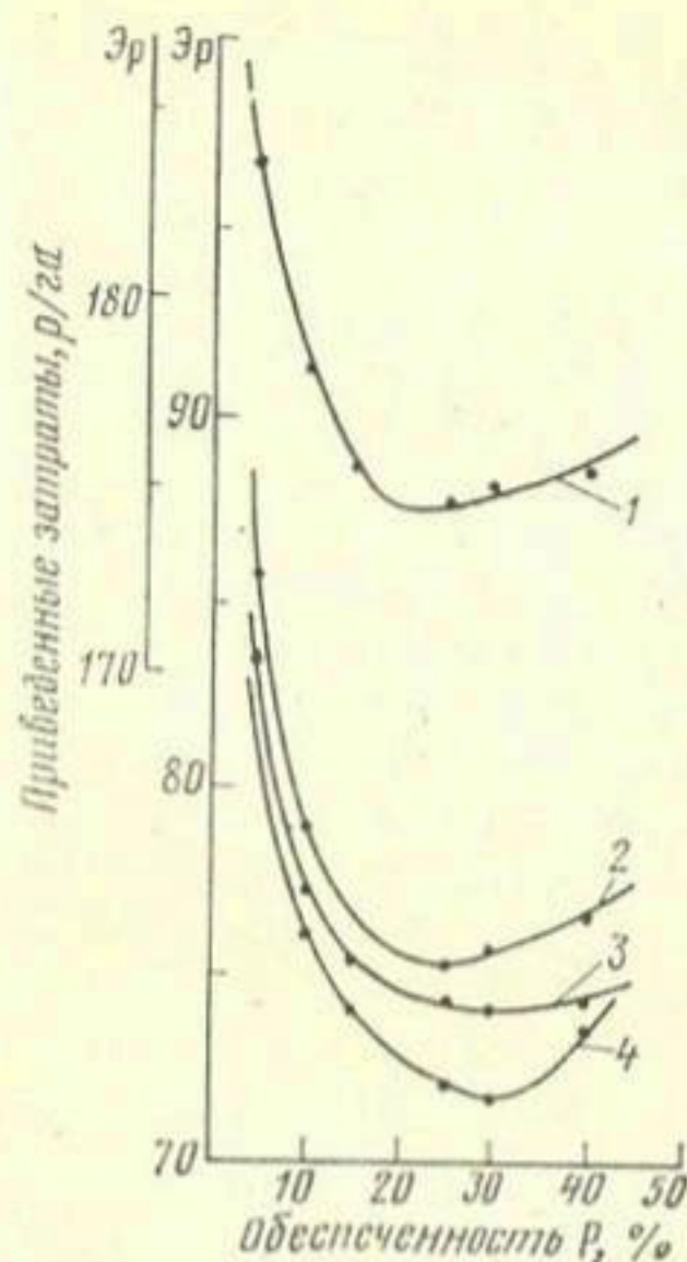
Рис. 2. График для определения расчетной обеспеченности максимальных расходов весеннего половодья при разных способах осушения:
