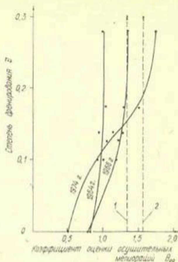
Рис. 3. График зависимости коэффициента оценки осушительных мелиораций B_{oc} от степени дренирования:
