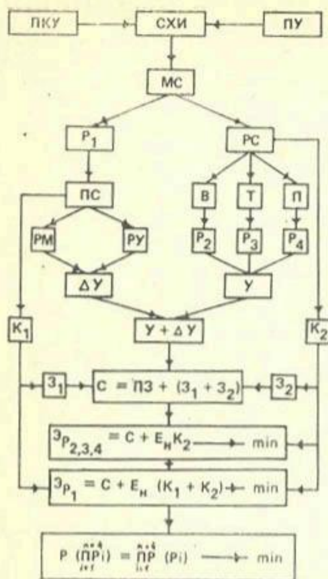
Рис. 1. Принципиальная схема выбора расчетной обеспеченности осушительных систем.
