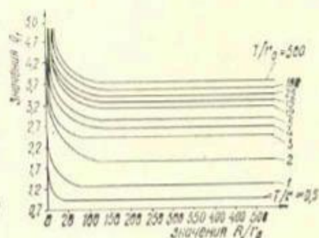
Рис. 9. Кривая изменения приведенного расхода q_1 в зависимости от отношения R/r_0 для различных значений T/r_0 .
