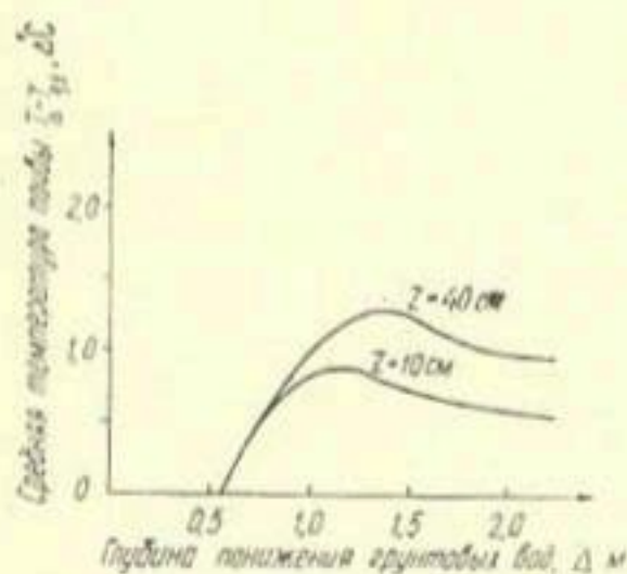
Рис. 5. Зависимость средней за вегетацию температуры торфяной почвы T на глубине z=10 и 40 см от глубины понижения грунтовых вод \Delta при дождевании пшеницы.
