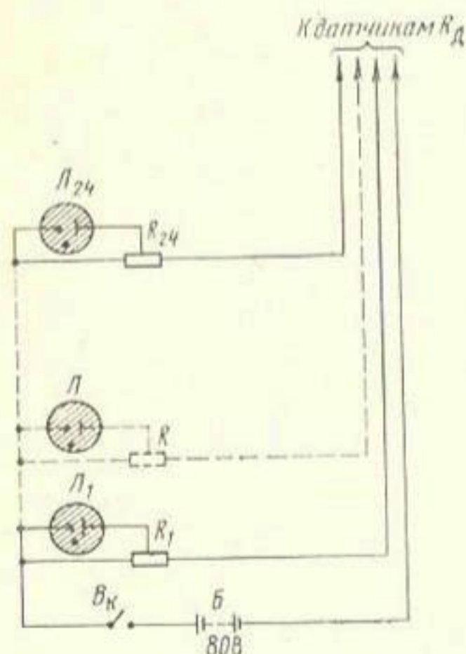
Рис. 2. Схема указателя глубины промерзания электрического мерзлотомера:
