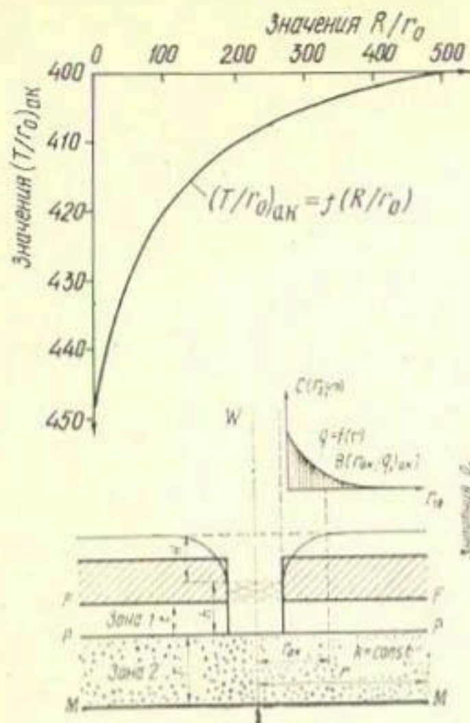
Рис. 8. Схема к определению значения (r_0)_{ак} .
