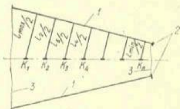
Рис. 1. Расположение пробных дрен и водомерных колодцев при полевом методе определения междренних расстояний.
