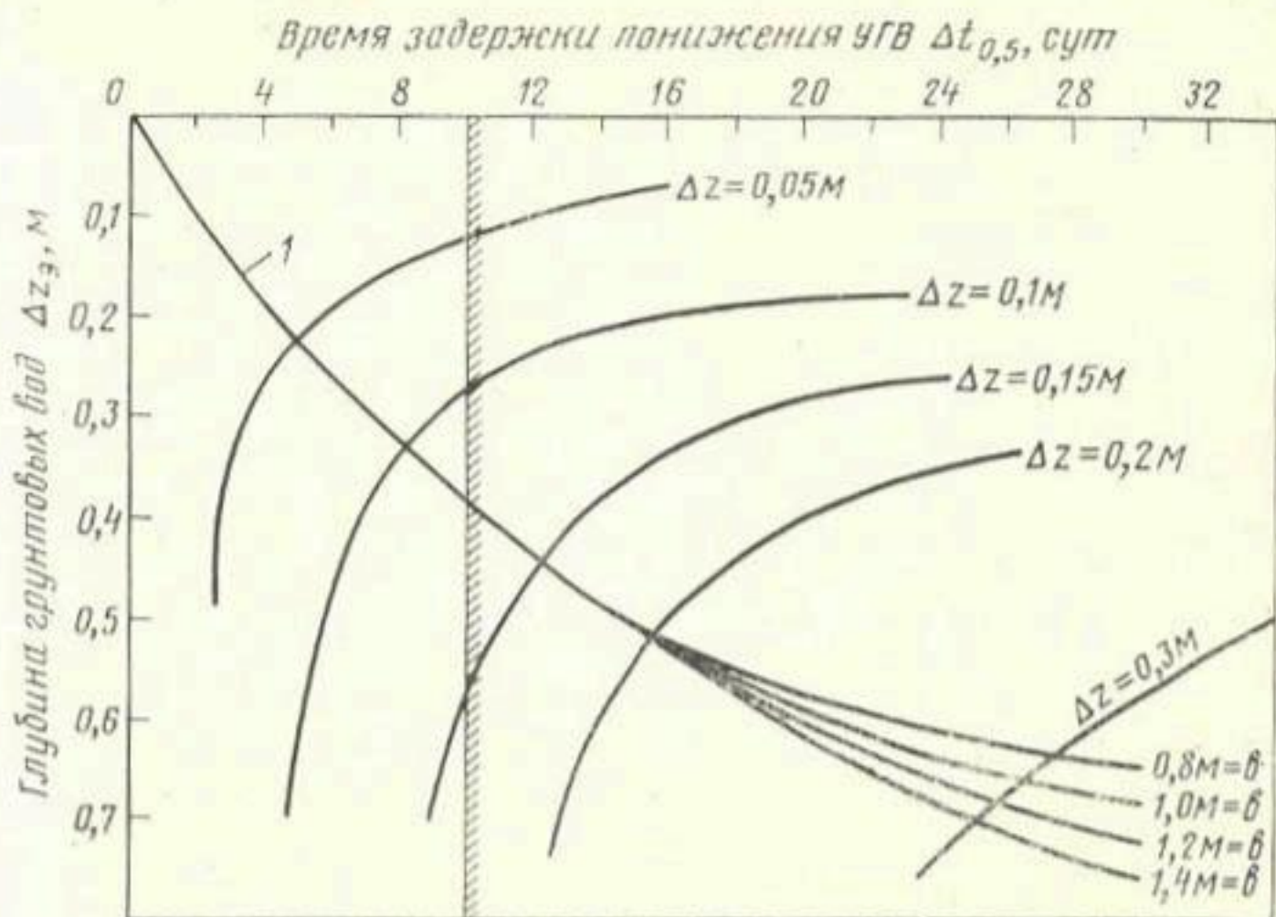
Рис. 1. Ход понижения уровня грунтовых вод в середине между дренами при расчетном режиме и зависимость \Delta z = f(z_0, \Delta t_{0.5}) : 1—расчетный режим; \Delta z —отклонение глубины уровней грунтовых вод, м; \Delta z_0 —глубина уровня грунтовых вод на эталонном участке, м; \Delta t_{0.5} —время задержки понижения уровня грунтовых вод до нормы осушения, равной 0,5 м, сут.
