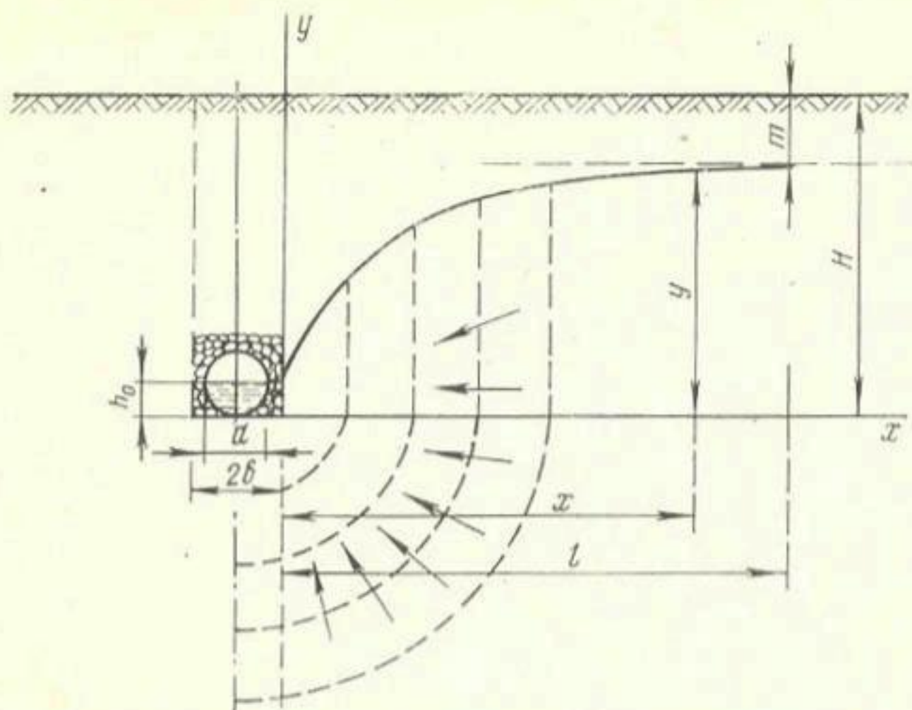
Рис. 1. Схема расчета закрытого дренажа в зонах с продолжительными осадками.
