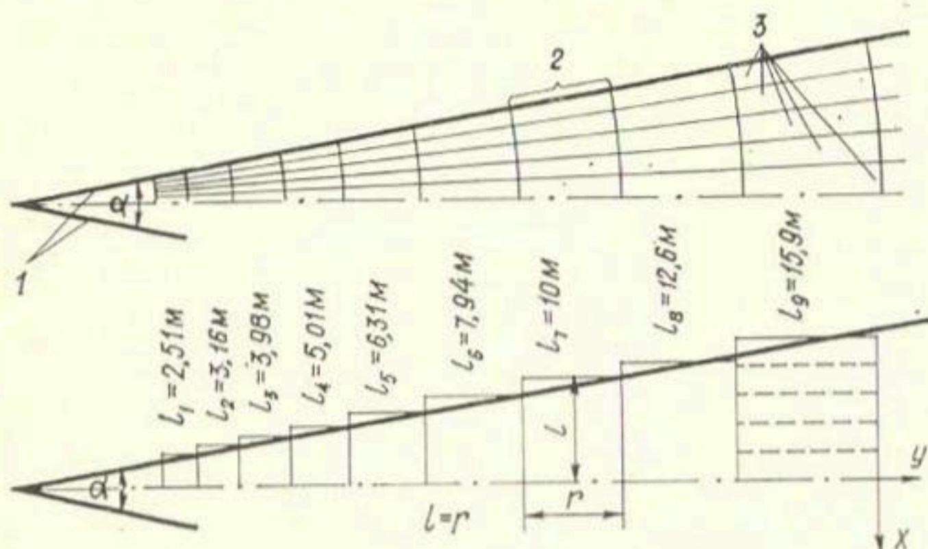
Рис. 2. Схематизация области фильтрации «дренажного клина» при \alpha = 26^\circ \text{C} :
