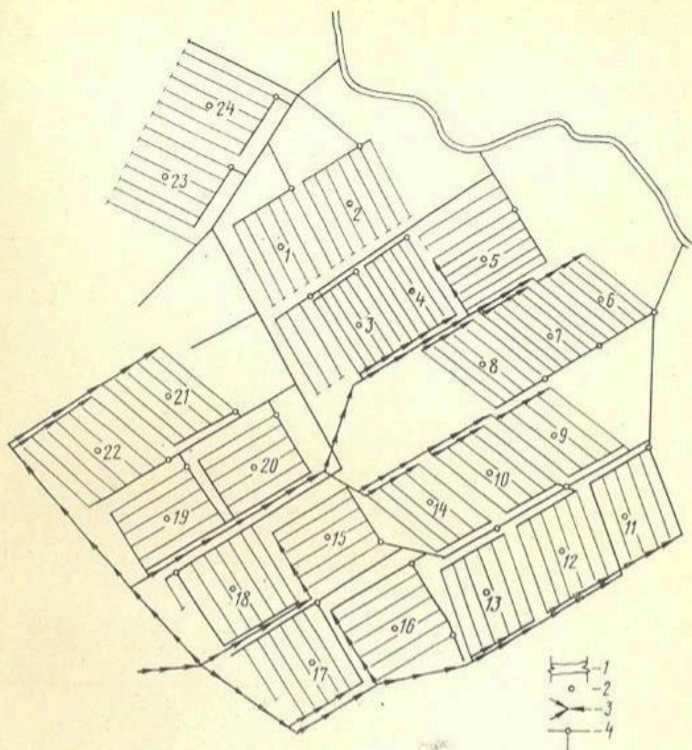
Рис. 1. Схема коллекторно-дренажной сети опытного участка «Молодая»:
