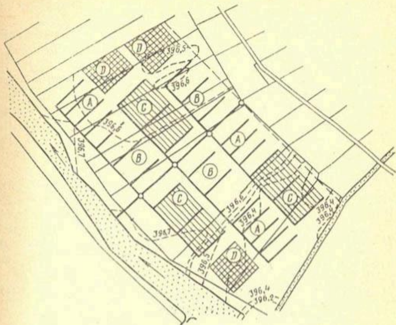
Рис. 1. Схема опытного участка Хехст в Австрии:
