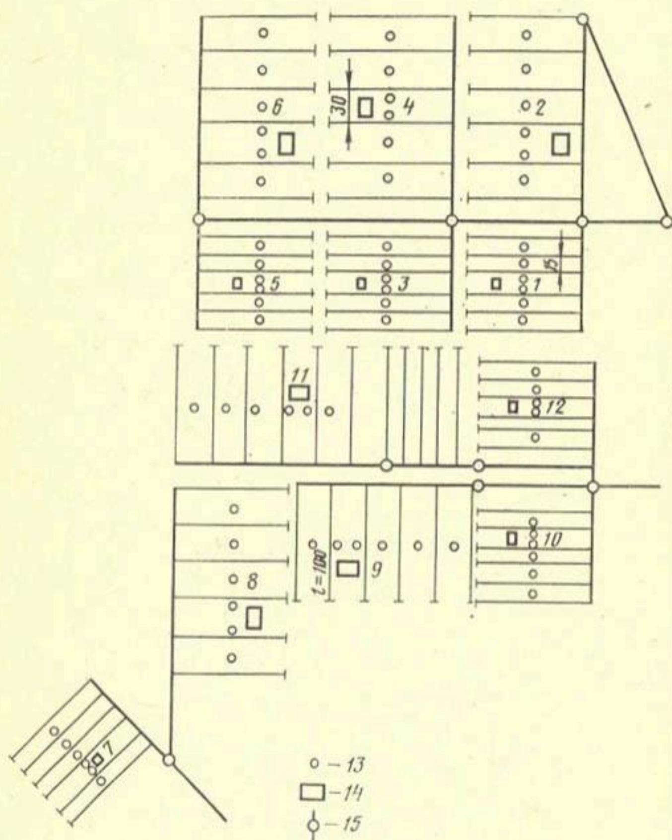
Рис. 2. План коллекторно-дренажной сети опытного участка «Пындино». Варианты опыта:
