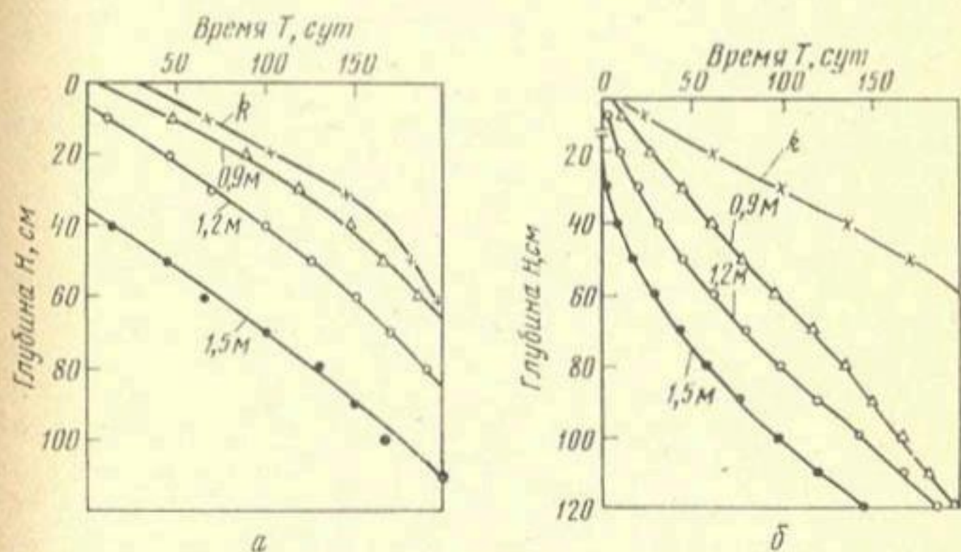
Рис. 4. Кривые продолжительности (обеспеченности) стояния уровней грунтовых вод на суглинистых почвах в системах глубокого (1,5 м), среднеглубокого (1,2 м), мелкого (0,9 м) дренажа и на контрольном (недренированном) участке (опытный объект «Римей-кас» в совхозе «Ауструми» Валмиерского района):
