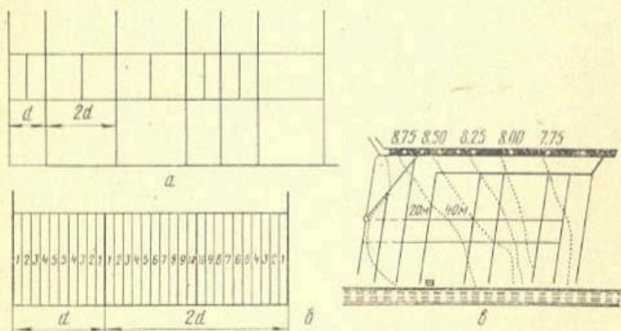
Рис. 5. Принципиальная схема опытов и опытный участок Уибын в Швеции:
