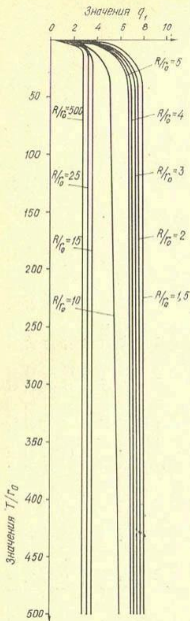
Рис. 6. График изменения приведенного расхода q_1 = f(R/r_0, T/r_0) .
