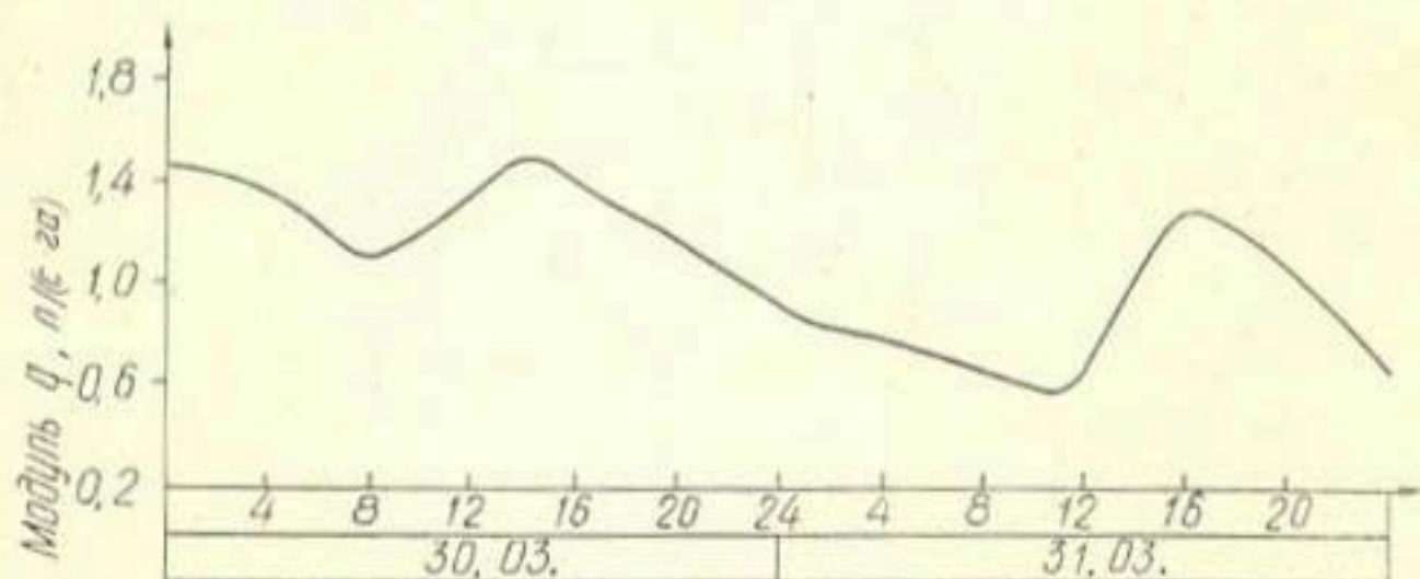
Рис. 2. Календарный график дренажного стока, зарегистрированный самописцем уровня «Валдай» в системе опытного пластмассового дренажа, заложенного на объекте «Бауска» Бауского района.
