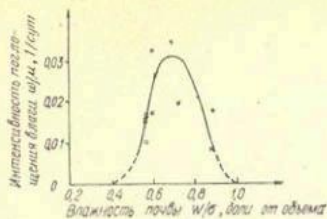
Рис. 7. Зависимость интенсивности поглощения влаги корнями растений \omega/\mu от влажности почвы w .
