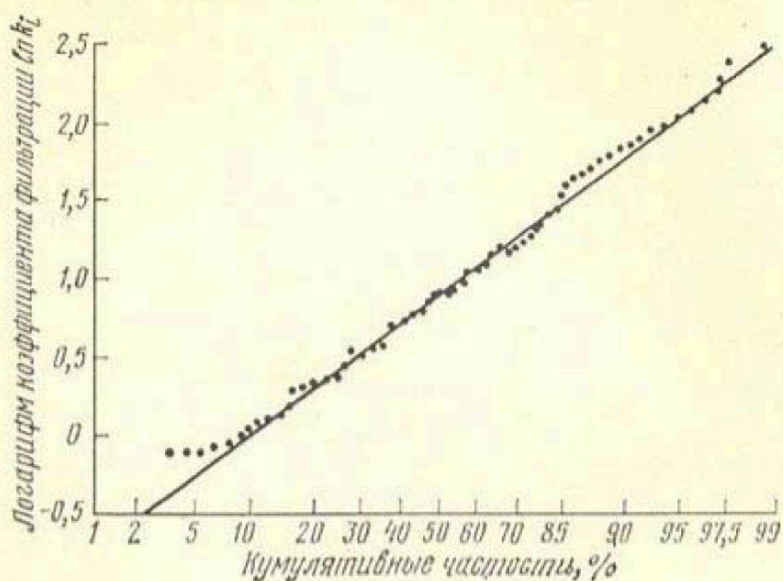
Рис. 1. График накопленных частот логарифмов значений водопроницаемости.
