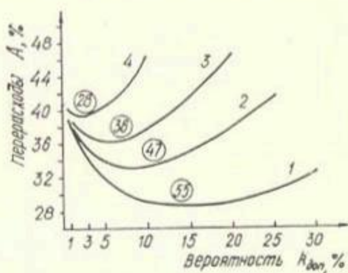
Рис. 3. Зависимости перерасходов A от вероятности k_{\text{дон}} и года конструкции (1...4) систем: 55, 47, 36, 28 — оптимальная вероятность k_{\text{расч}} ; 1, 2, 3, 4 — год реконструкции
