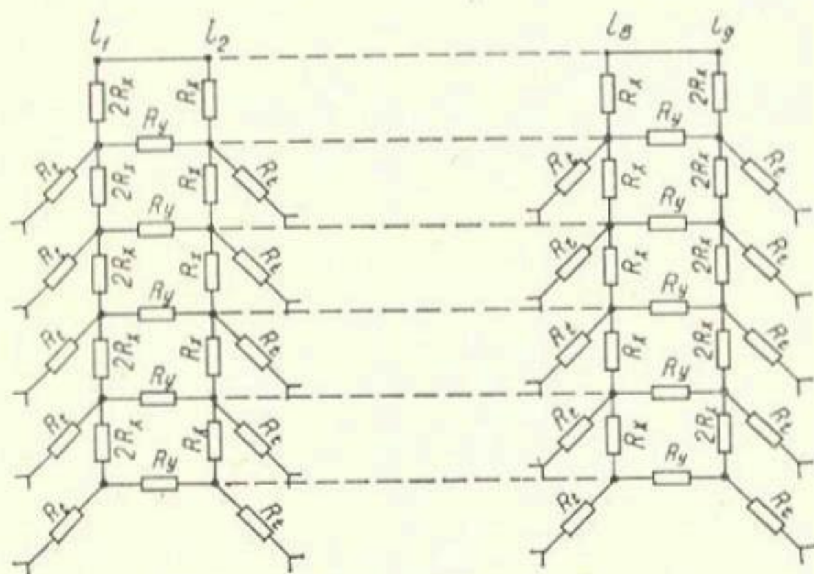
Рис. 3. Общая электрическая схема сеточной модели.
