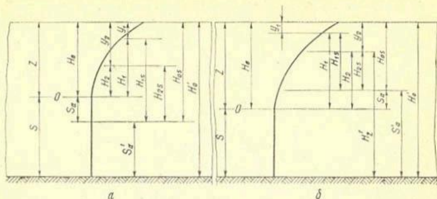
Рис. 1. Схемы расчета средних значений водно-физических свойств в неоднородных почвогрунтах.
