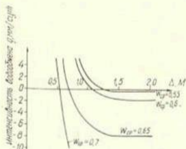
Рис. 2. Изменение средней за вегетацию интенсивности водообмена почвенных и грунтовых вод в зависимости от их глубины при различных значениях влажности почвы (влажность показана в долях от объема на кривых).
