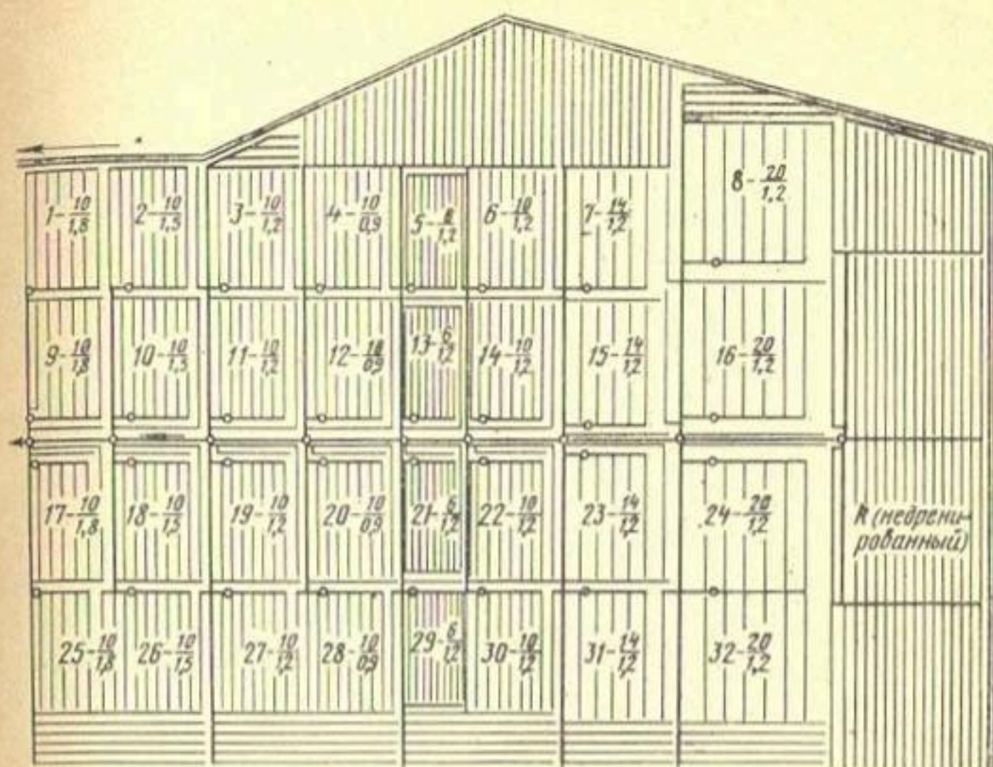
Рис. 1. Системы (варианты) опытного дренажа, заложенные на глинистых почвах на объекте «Силлауки» колхоза «Драудзиба Талсинского района Латвийской ССР:
