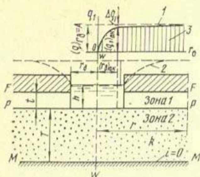
Рис. 11. Изменение расхода q_1 в зависимости от радиуса ко- лодца r_0 : 1 — асимптота; 2 — кривая напоров; 3 — эпюра q_1 = f(r_0) .
