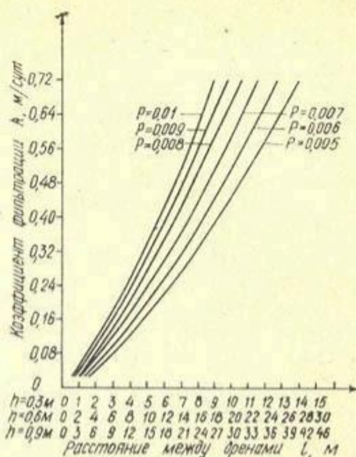
Рис 3. Изменение параметра l в зависимости от коэффициента фильтрации K и интенсивности питания P в формуле L = 2(l + b) .
