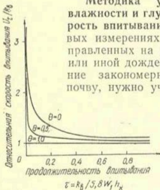
Рис. 8. Изменение динамики впитывания в зависимости от начальной влажности w_n :
