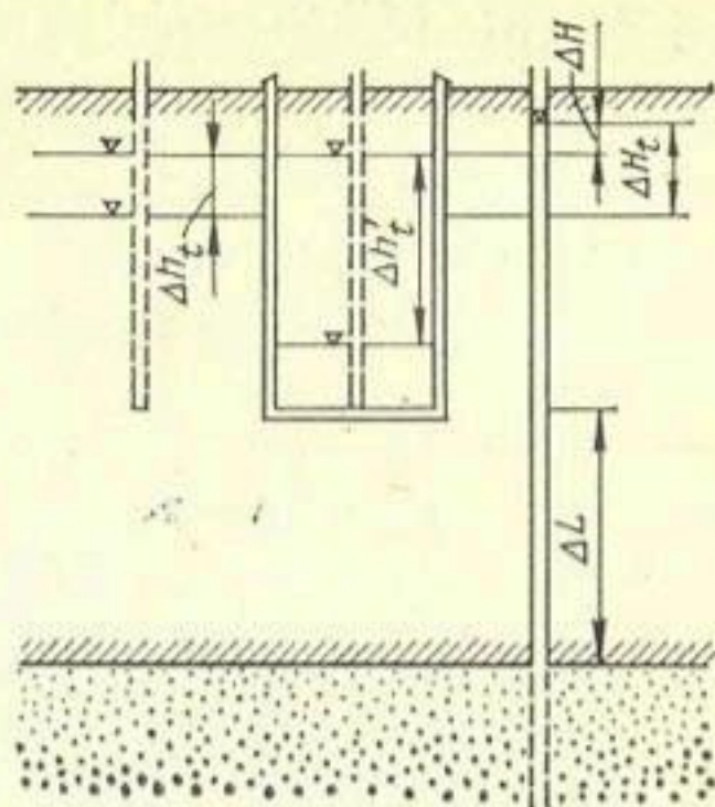
Рис. 4. Схема установки испарителя и пьезометров при определении притока напорных грунтовых вод.
