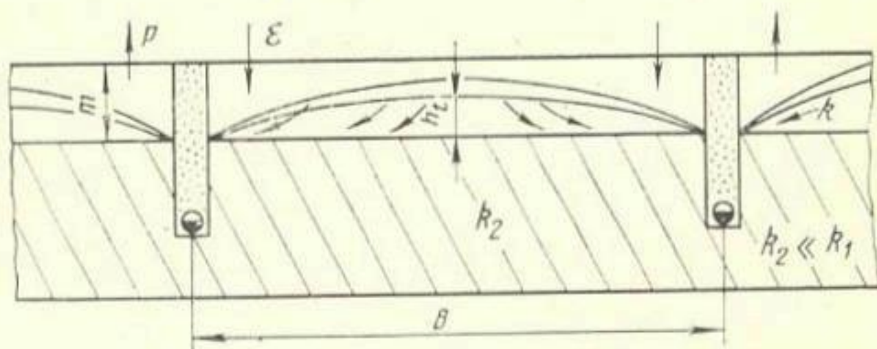
Рис. 3. Схема корнеобитаемого слоя тяжелых почв.
