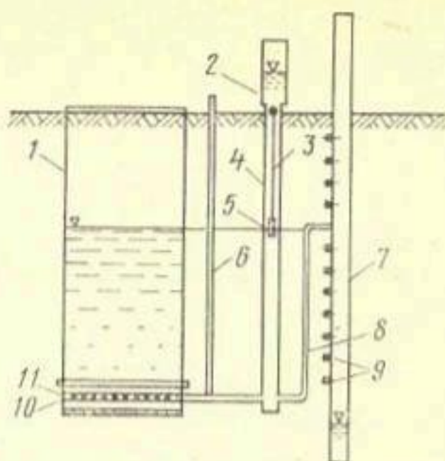
Рис. 1. Схема металлического сварного лизиметра с автоматическим устройством регулирования уровня грунтовых вод: 1 — корпус; 2 — компенсатор; 3 — тросик; 4 — компенсационная труба; 5 — поплавок; 6 — наблюдательная труба; 7 — инфильтрационная труба; 8 — сливная резиновая трубка; 9 — штуцер; 10 — поддон; 11 — перфорированная труба.
