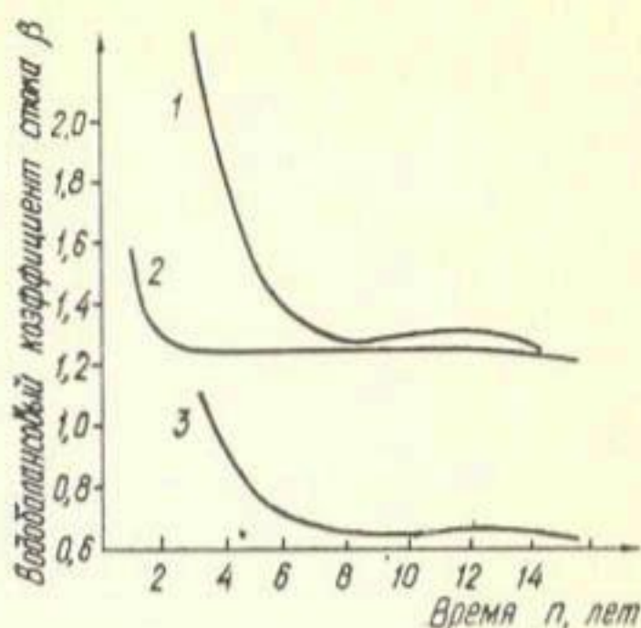
Рис. 1. Изменение воднобалансового коэффициента стока по скользящим n -летиям:
