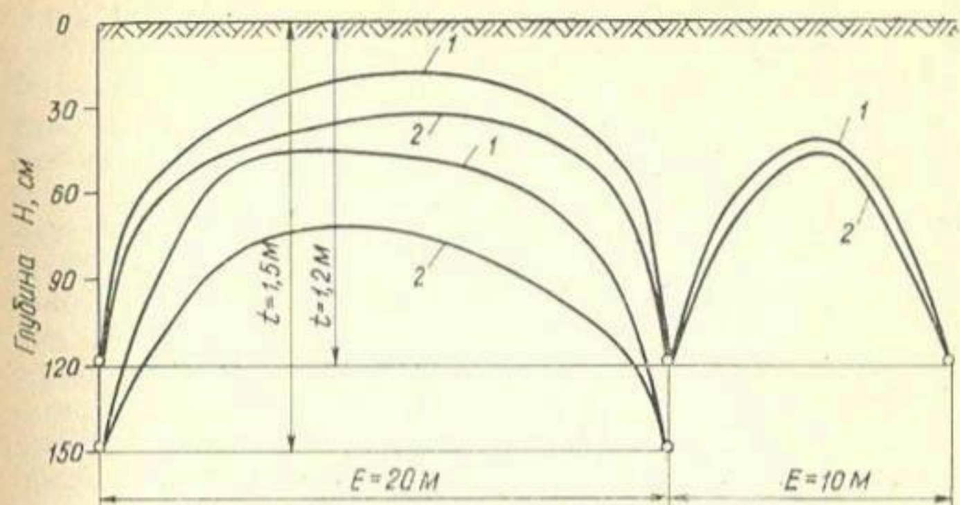
Рис. 3. Характерные кривые депрессии уровней грунтовых вод на тяжелых слабопроницаемых почвах ( k=2 \dots 16 см/сут) в системах глубокого (1,5 м) и среднеглубокого (1,2 м) дренажа при междренном расстоянии 20 и 10 м на опытном объекте «Дегумнирки» совхоза «Айвибекте» Мадоуского района.
