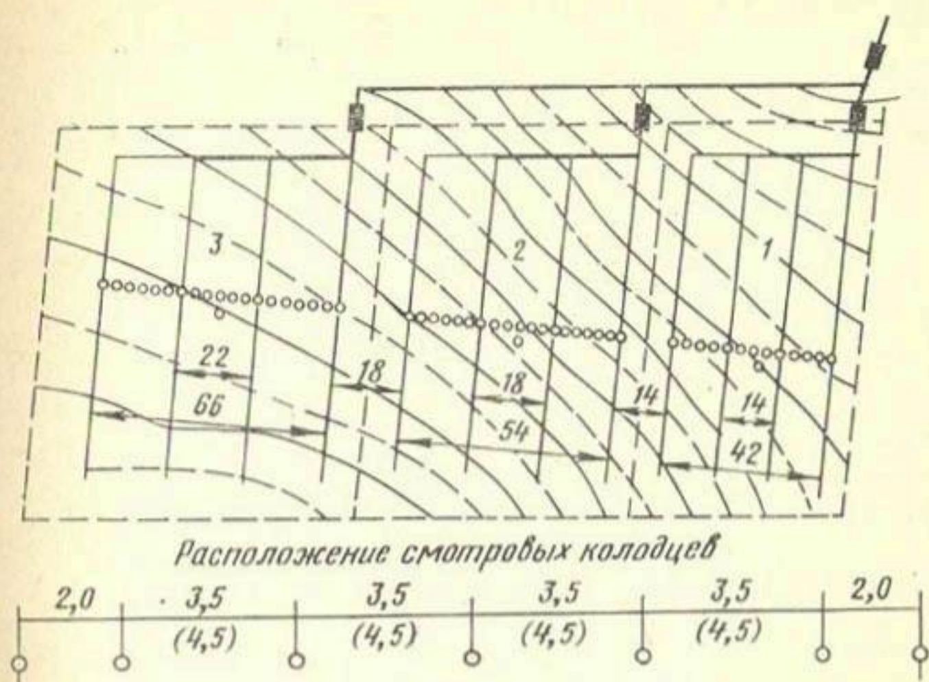
Рис. 3. Схема опытного участка Пургшталь в Австрии.
