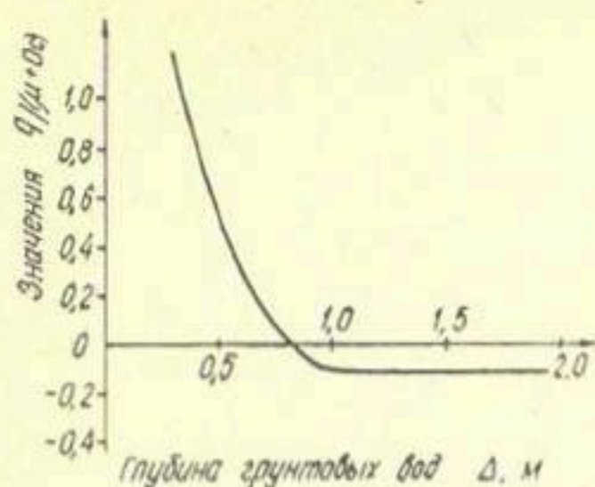
Рис. 3. Изменение суммарного за сезон водообмена зоны аэрации с грунтовыми водами, отнесенного к суммарной водоподаче q(m+O_c) , в зависимости от глубины грунтовых вод при дождевании трав.
