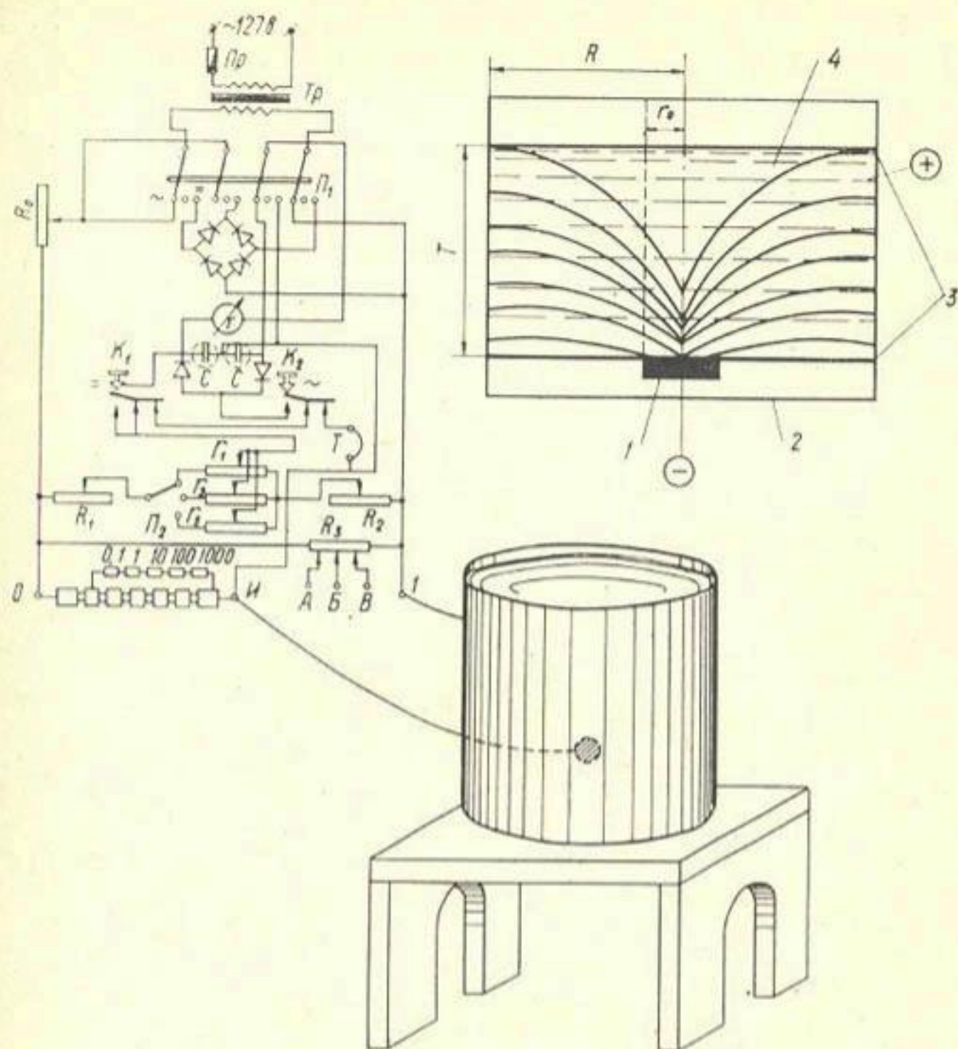
Рис. 4. Схема (а) и вертикальное сечение модели (б) опыта по определению расхода q_1 методом ЭГДА: 1 — ртуть; 2 — дерево; 3 — латунь; 4 — жидкость.
