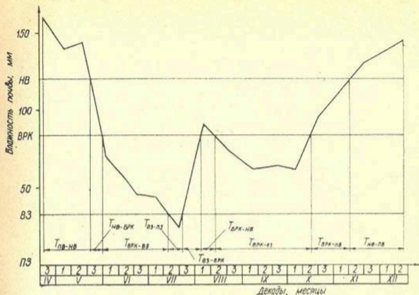
Рис. 2. Динамика общих запасов влаги на 5-м опытном участке дренажа учебного хозяйства Литовской СХА (слой почвы 0...40 см).
