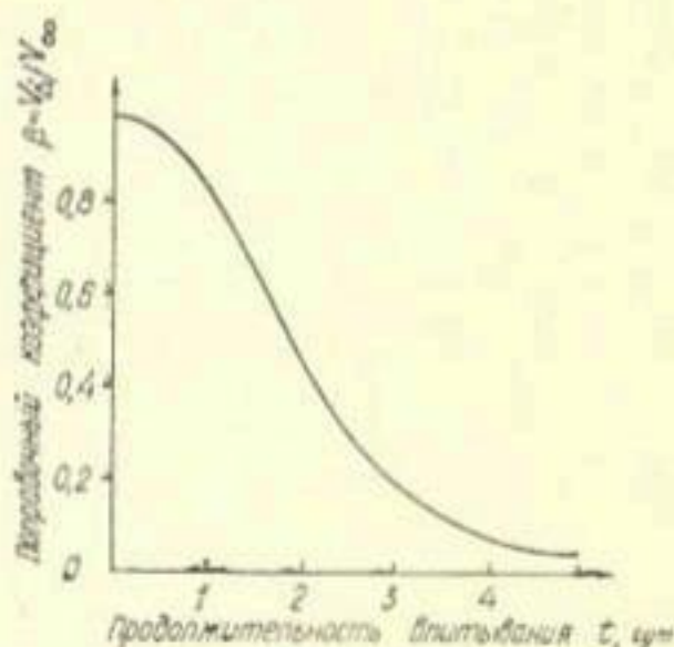
Рис. 9. График изменения поправочного коэффициента \beta = V_\Delta / V_\infty в формуле (18) в зависимости от глубины грунтовых вод \Delta .
