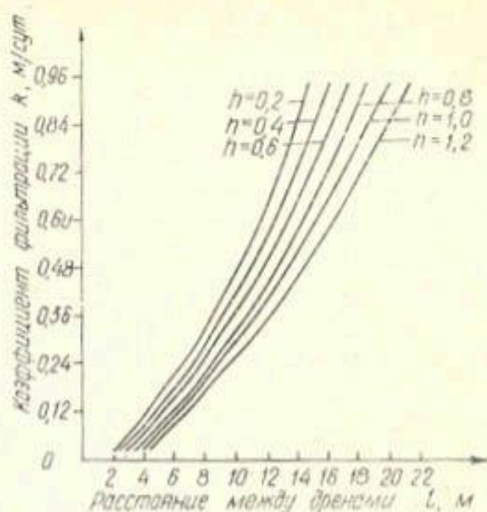
Рис. 4. Изменение параметра l в зависимости от коэффициента фильтрации K и перепада напора h с учетом интенсивности P = 0,02K + 0,0076 .
