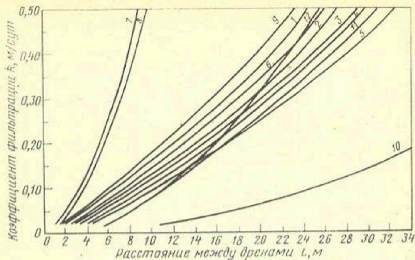
Рис. 2. Расчетные значения междренних расстояний, рекомендуемые различными авторами:
