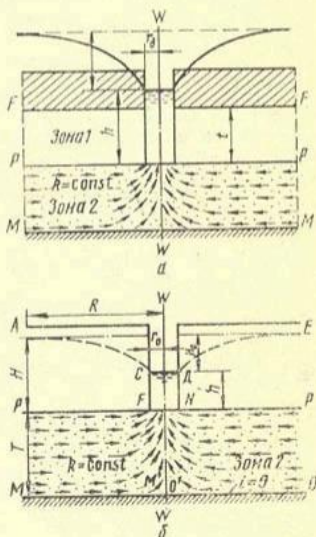
Рис. 3. Зоны фильтрации, питающие дно колодца: а — напорного потока; б — безнапорного потока.
