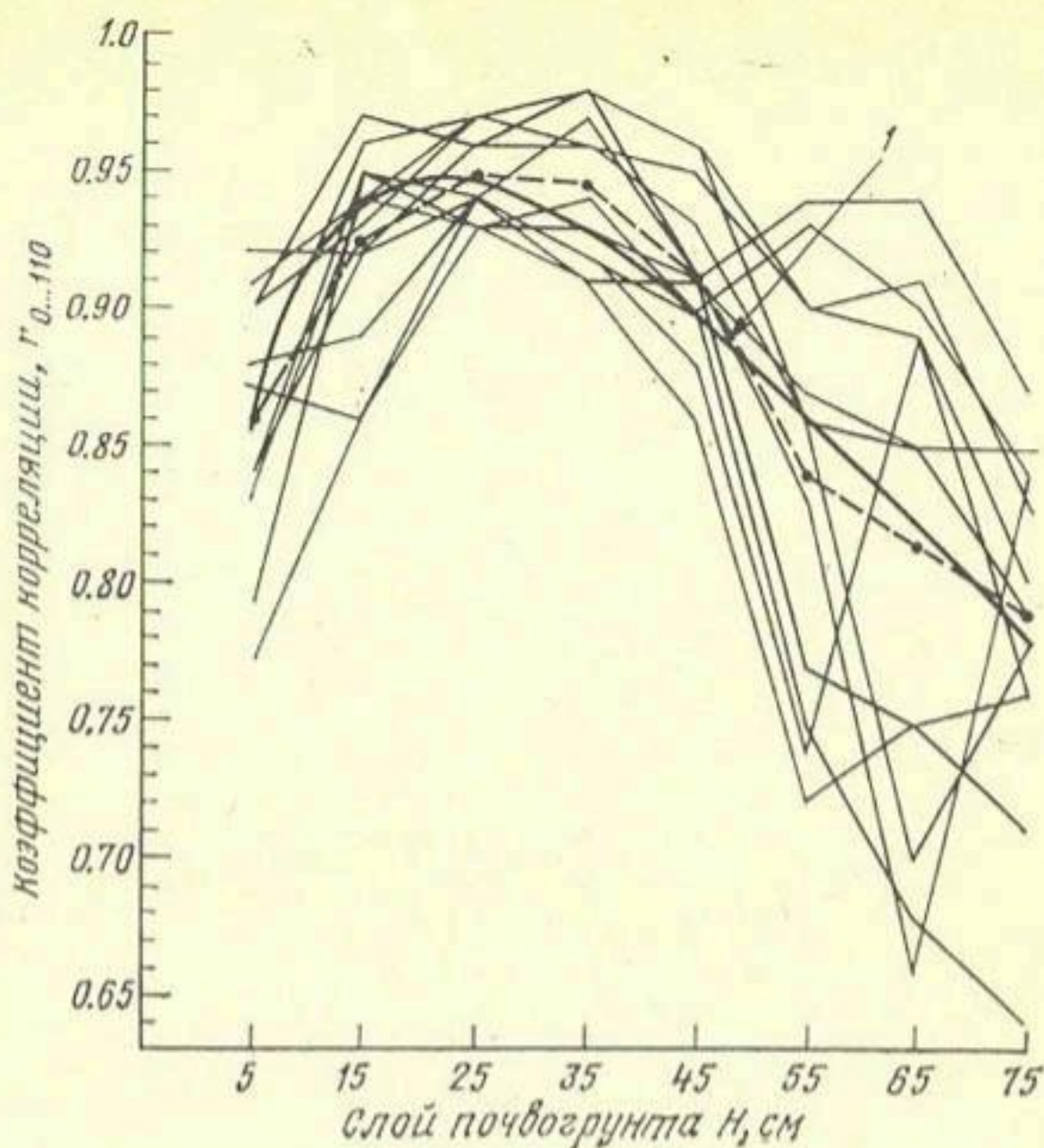
Рис. 2. Результаты корреляционного анализа и нахождение формы зависимости почвенной влажности 10-сантиметровых слоев со средней мощностью слоя 0...110 см по данным трехлетних наблюдений на четырех водобалансовых площадках:
