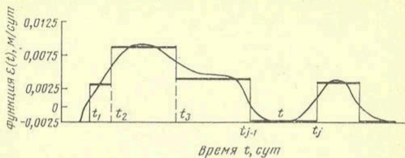
Рис. 2. Аппроксимация кривой инфильтрационного питания ступенчатой кривой.
