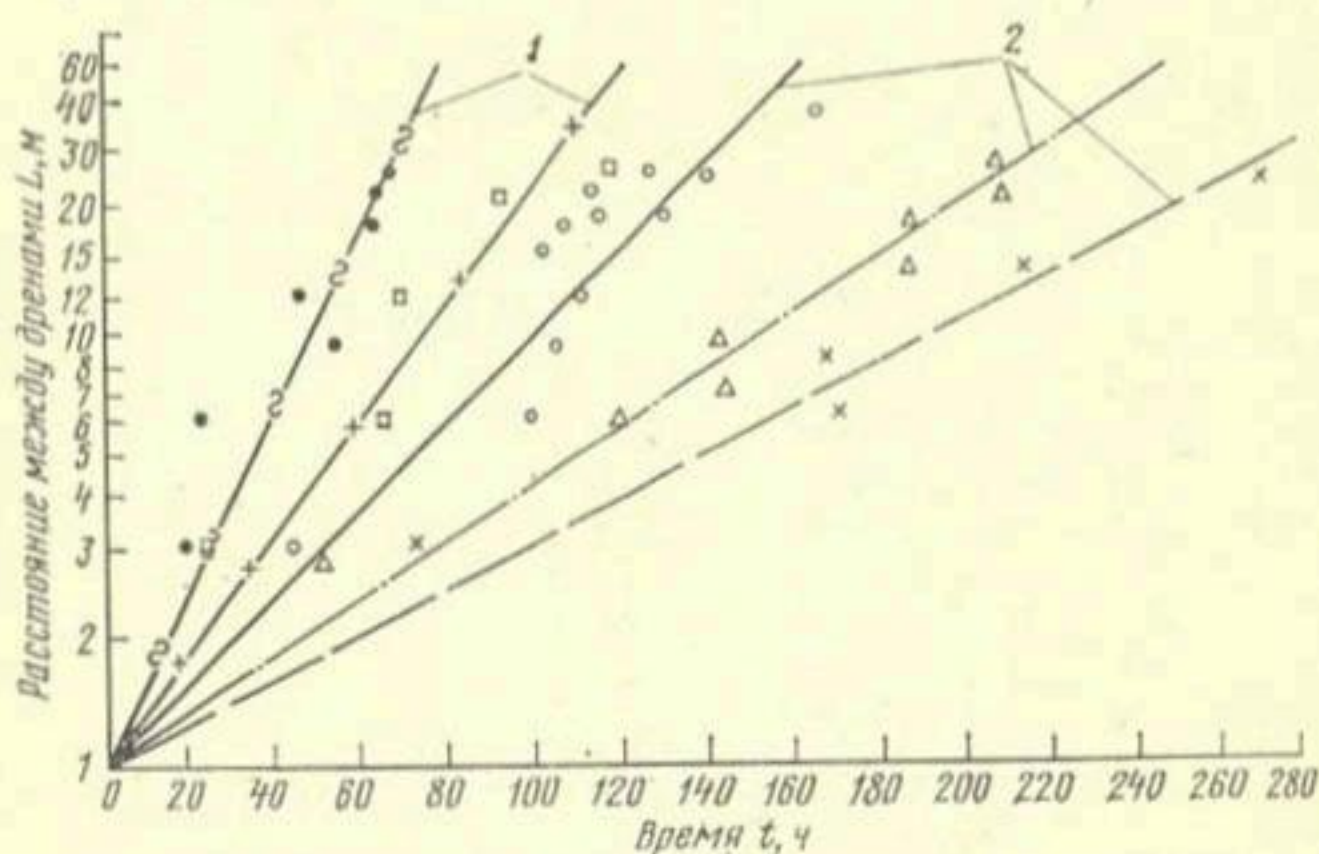
Рис. 4. Зависимость t=f(L) для тяжелых суглинков (ОПХ Карельской ОМС):
