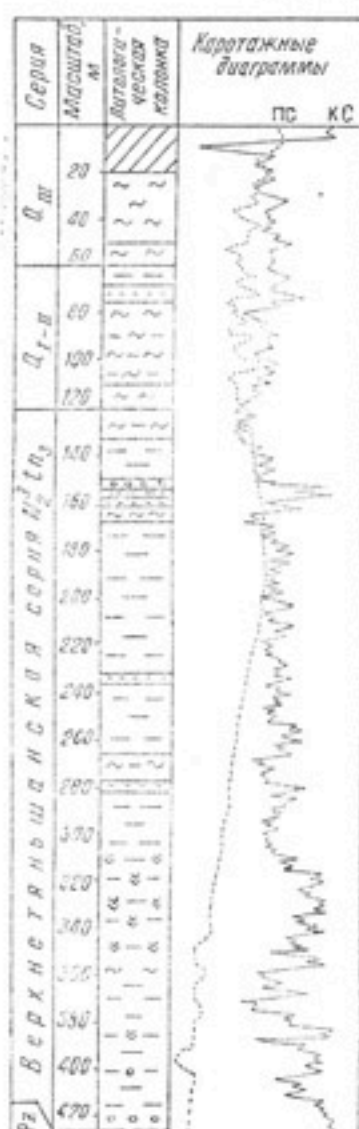
Рис. 11. Характер строения верхнетяньшанской серии на окраине преднуратинской пролювиальной равнины, разрез скв. 4.
