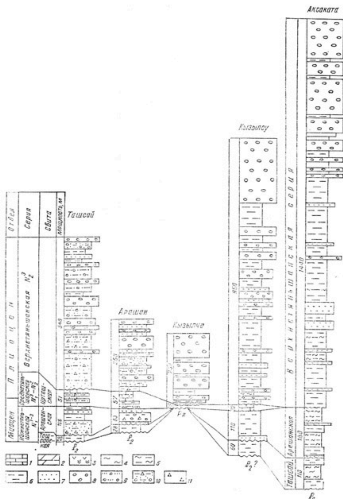
Рис. 3. Схема сопоставления опорных разрезов неогена долины Чирчика (Ак-Са-ката, Кызыласу) и Ангrena (Ташсай, Арашан, Кызылча). Литологические типы пород:
