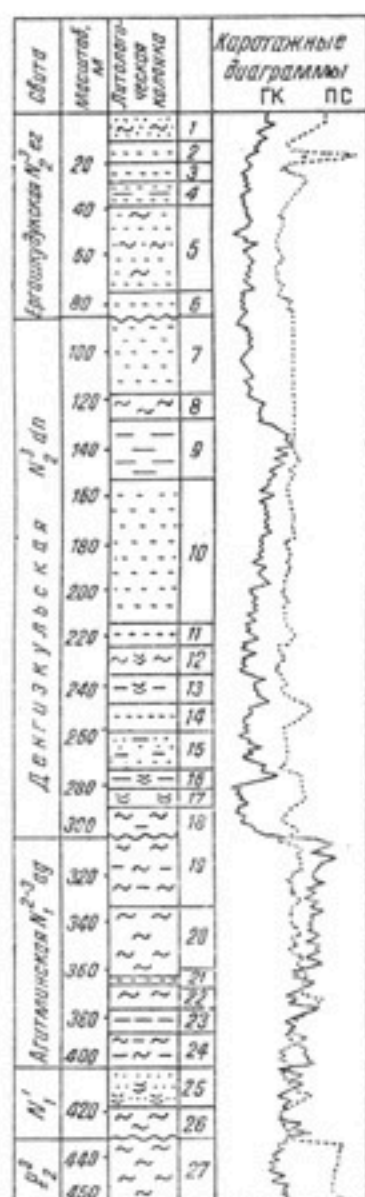
Рис. 19. Строение денгизкульской и ергашкудукской свит в Восточных Кызылкумах, скв. 3.
