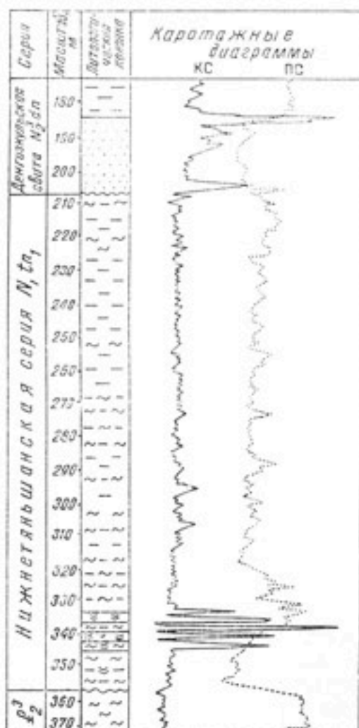
Рис. 7. Переслаивание (инт. 320—358) прибрежно-морских и лагунных глин и гипсов (повышение значения КС) с красноцветными континентальными алеврито-глинистыми породами нижнетяньшанской серии, скв. 5.
