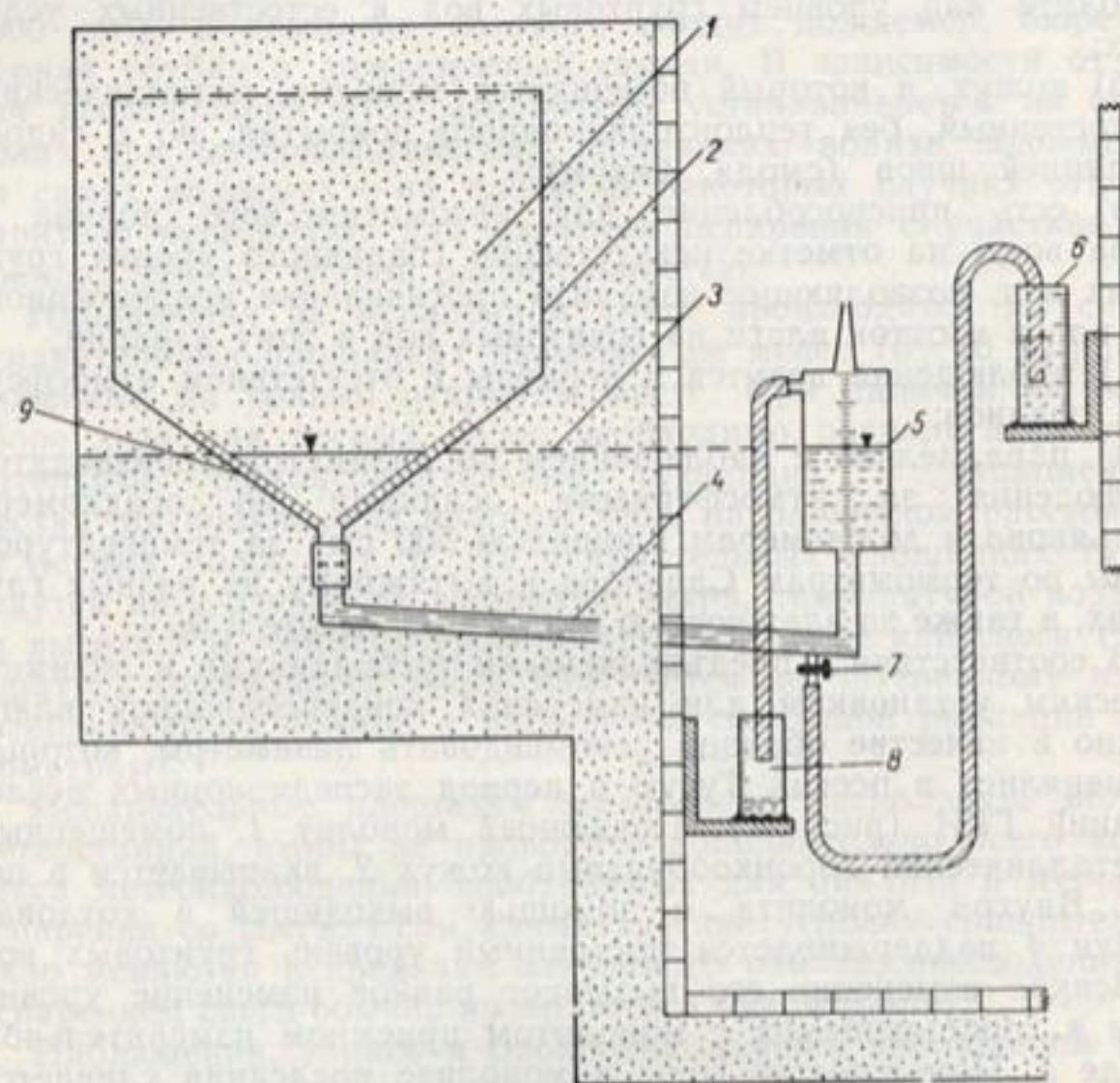
Рис. 21. Схема лизиметрической установки для измерения конденсации водяных паров в песке (разрез).
