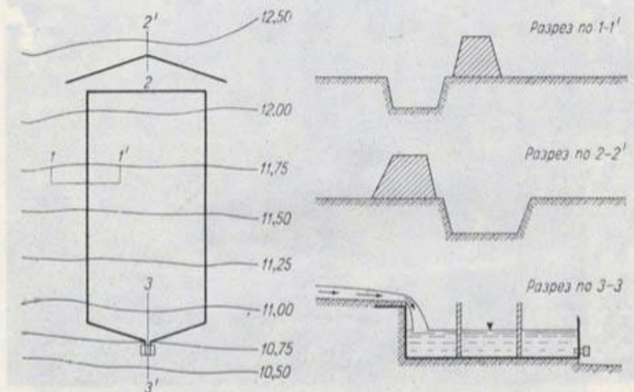
Рис. 9. План стоковой площадки, поперечные и продольные разрезы водораздельных и измерительного устройств.
