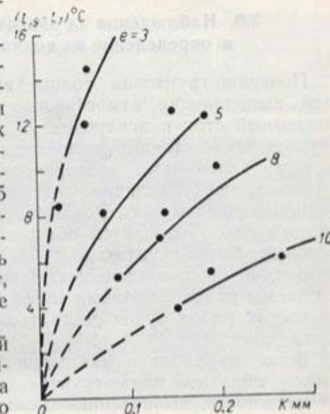
Рис. 22. Зависимость конденсации паров воздуха в слое песка 0,5 м от амплитуды колебаний температуры поверхности песка (t_{19} - t_7) и влажности воздуха e для температуры воздуха на 19 ч, равной 20° C.
