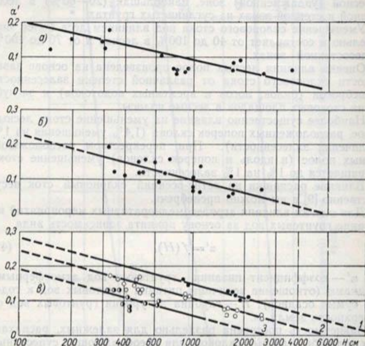
Рис. 34. Зависимость коэффициента питания грунтовых вод a' от глубины залегания их уровня H в средний по увлажненности год в лесостепной зоне для залежи (а), пашни (б) и лесных полос (в).
