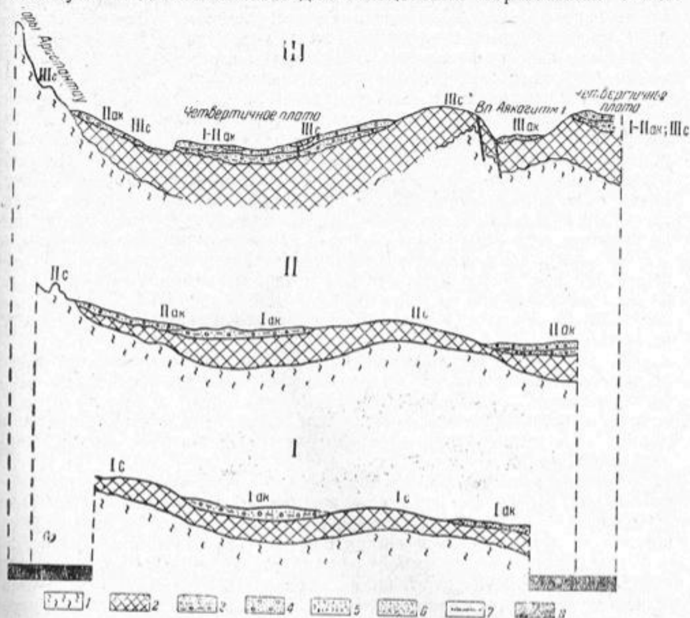
Рис. 6. Геоморфолого-структурные профили.
