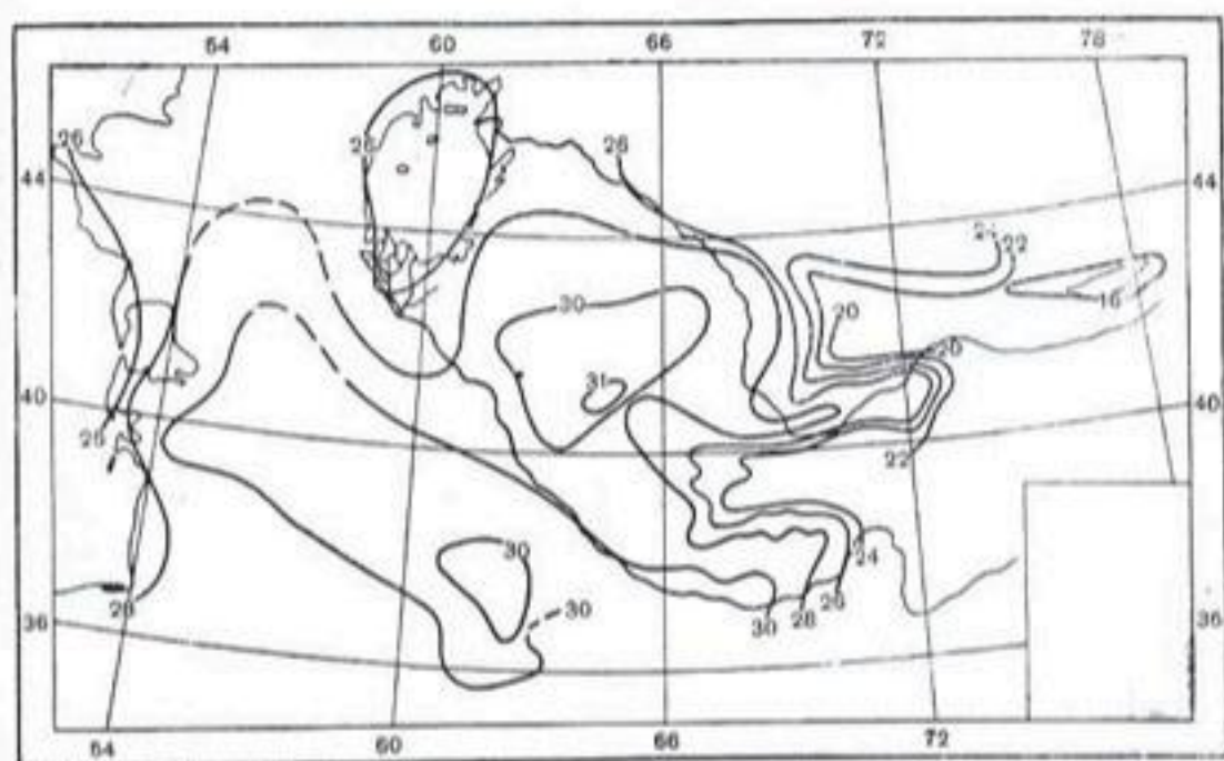
Рис. 53. Средняя месячная температура воздуха. Июль.
