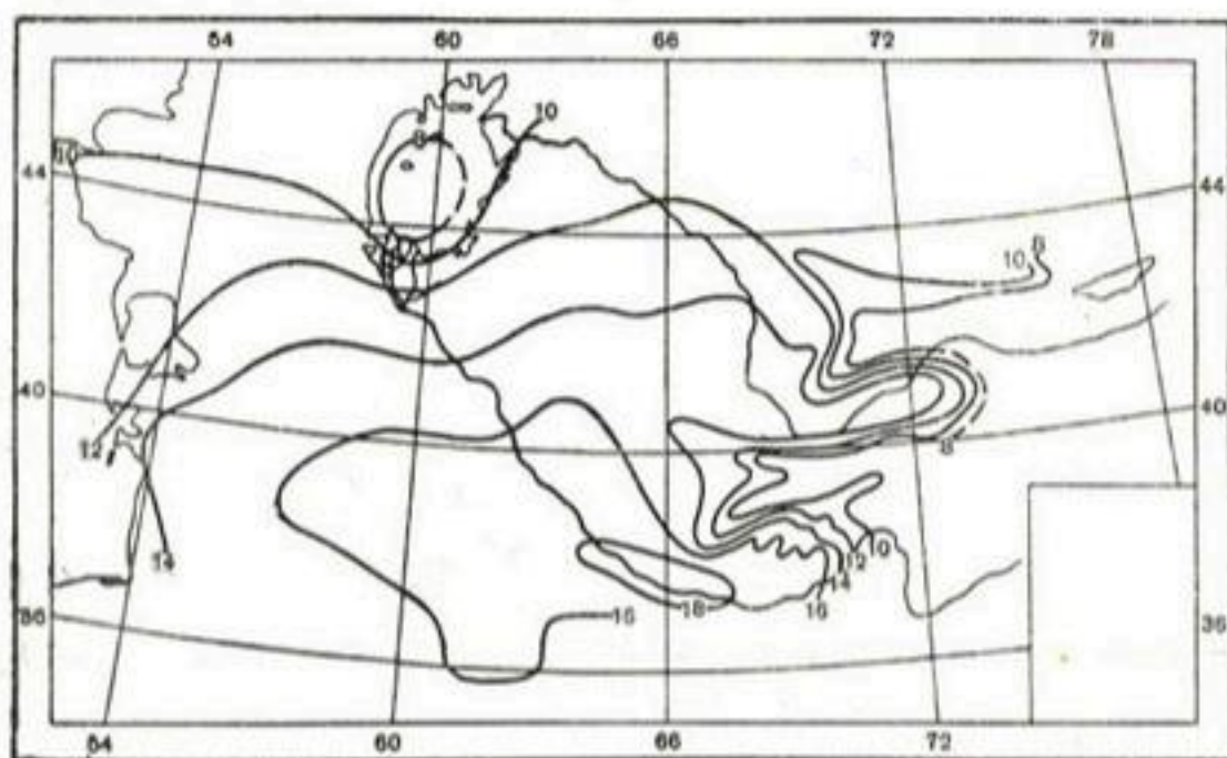
Рис. 52. Средняя месячная температура воздуха. Апрель.
