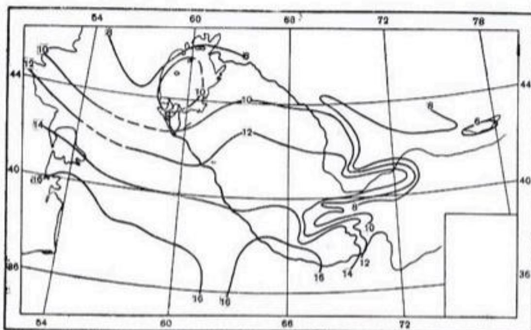
Рис. 54. Средняя месячная температура воздуха. Октябрь.
