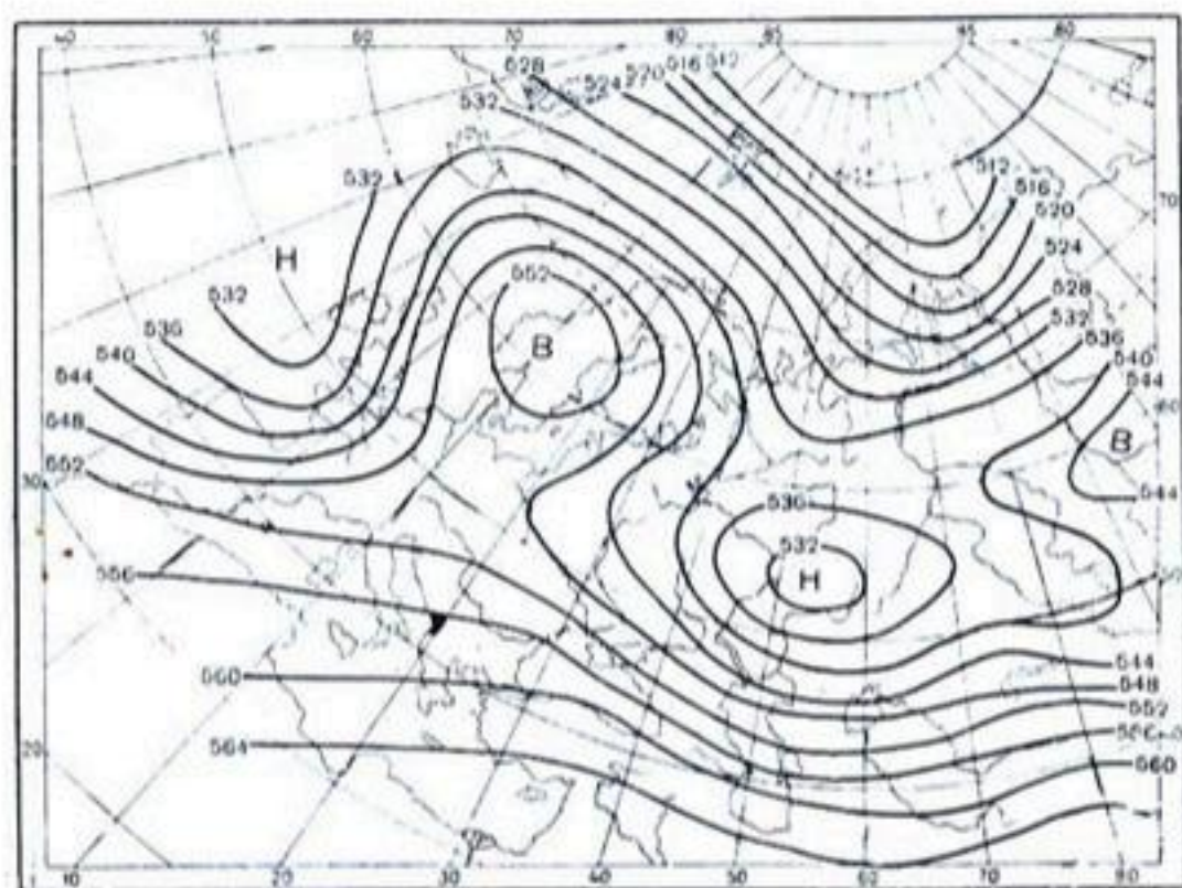
Рис. 17. Карта AT_{500} . 2—7/V 1947 г.
