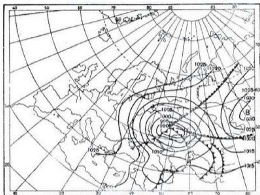
Рис. 42. Карта погоды, 15 час. 24/I 1951 г.
