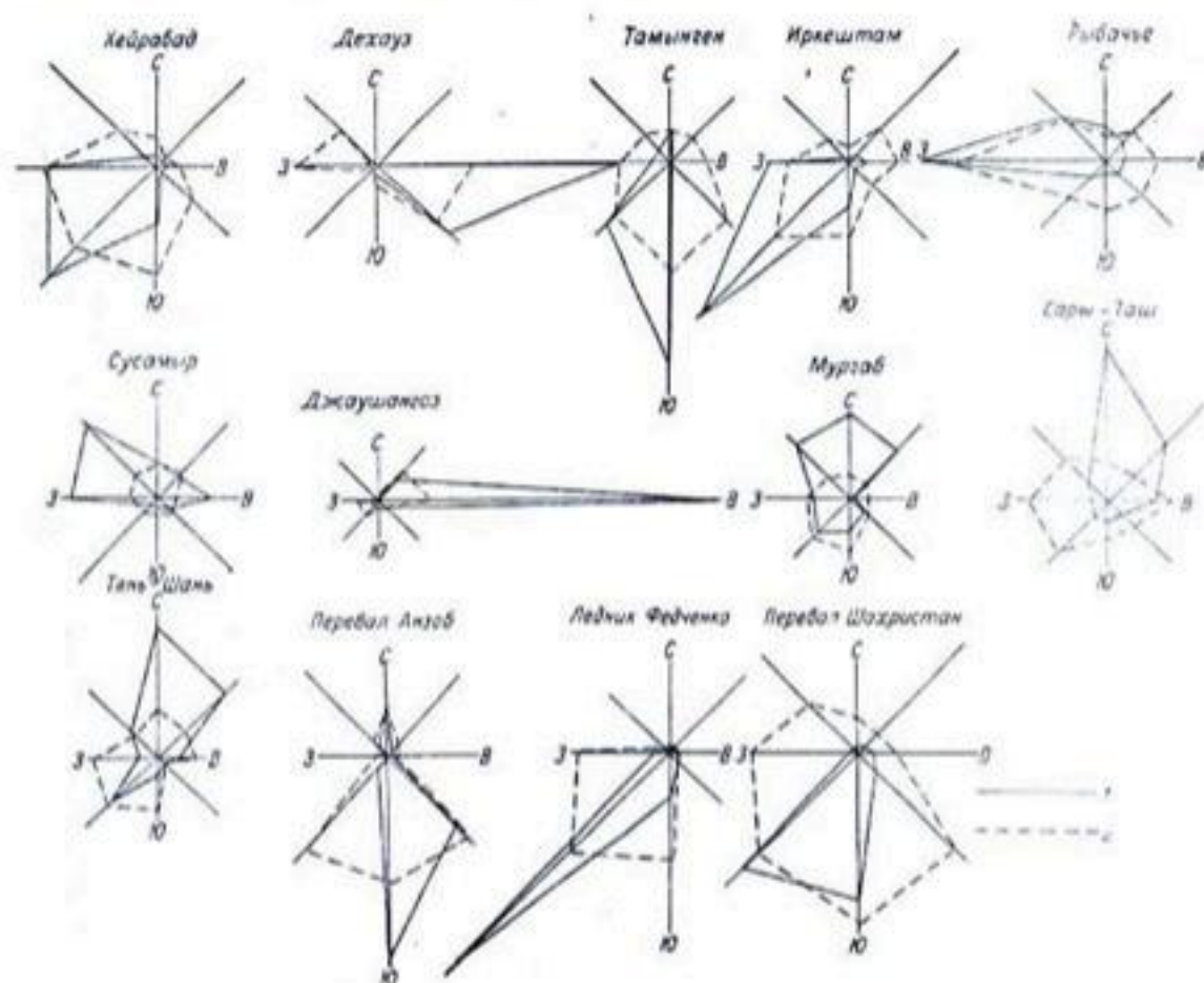
Рис. 45. Розы ветров в горной и высокогорной областях. Январь. 1 — направление ( ^{\circ} /а), 2 — скорость (м/сек.).
