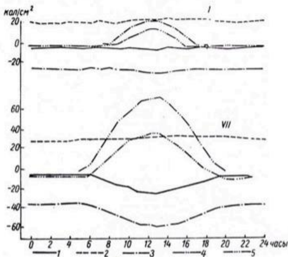
Рис. 13. Суточный ход суммарной радиации, излучения и радиационного баланса. Январь, июль. Ташкент, обсерватория. Излучение: 1 — эффективное, 2 — атмосферы, 3 — земли, 4 — суммарная радиация, 5 — радиационный баланс по наблюдениям Айзенштата над оголенной поверхностью.
