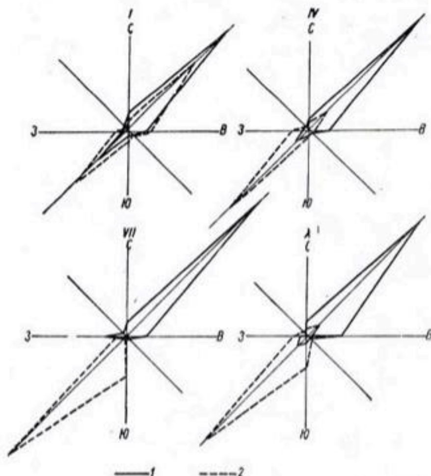
Рис. 41. Розы ветров в 1 час (1) и 13 час. (2). Аблык.
