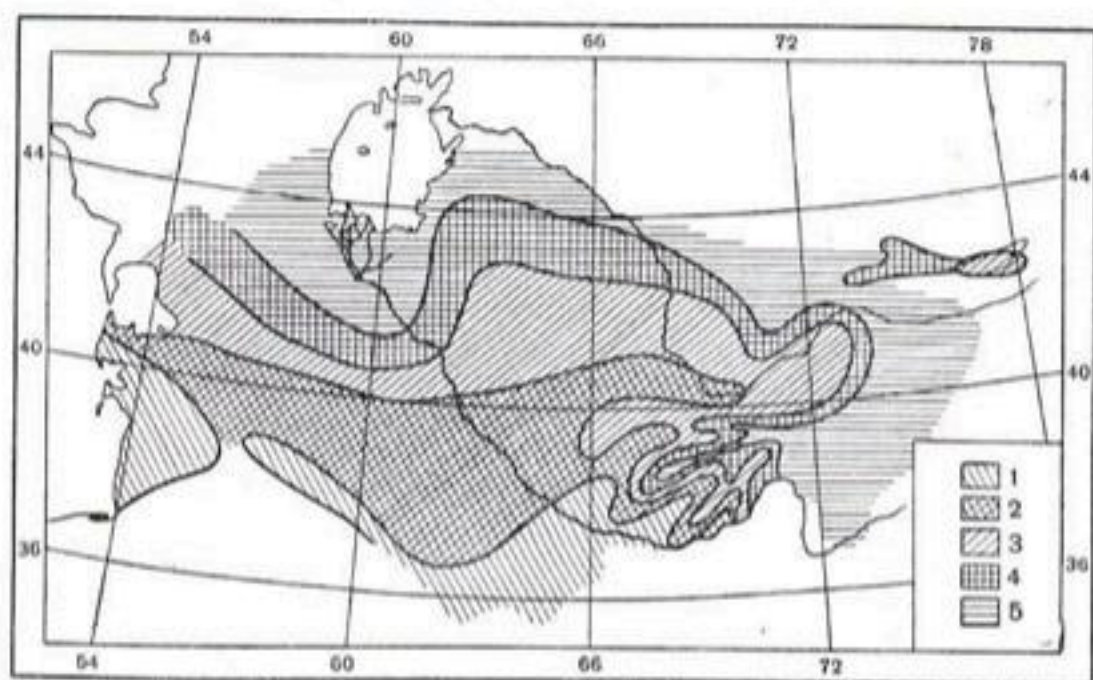
Рис. 60. Продолжительность устойчивых морозов.
