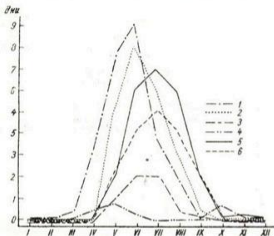
Рис. 90. Годовой ход числа дней с грозой. 1 — Перевал Анжоб, 2 — Сары-Таш, 3 — Мургаб, 4 — Ледник Федченко, 5 — Тинь-Шаньская обсерватория, 6 — Алтиярк.
