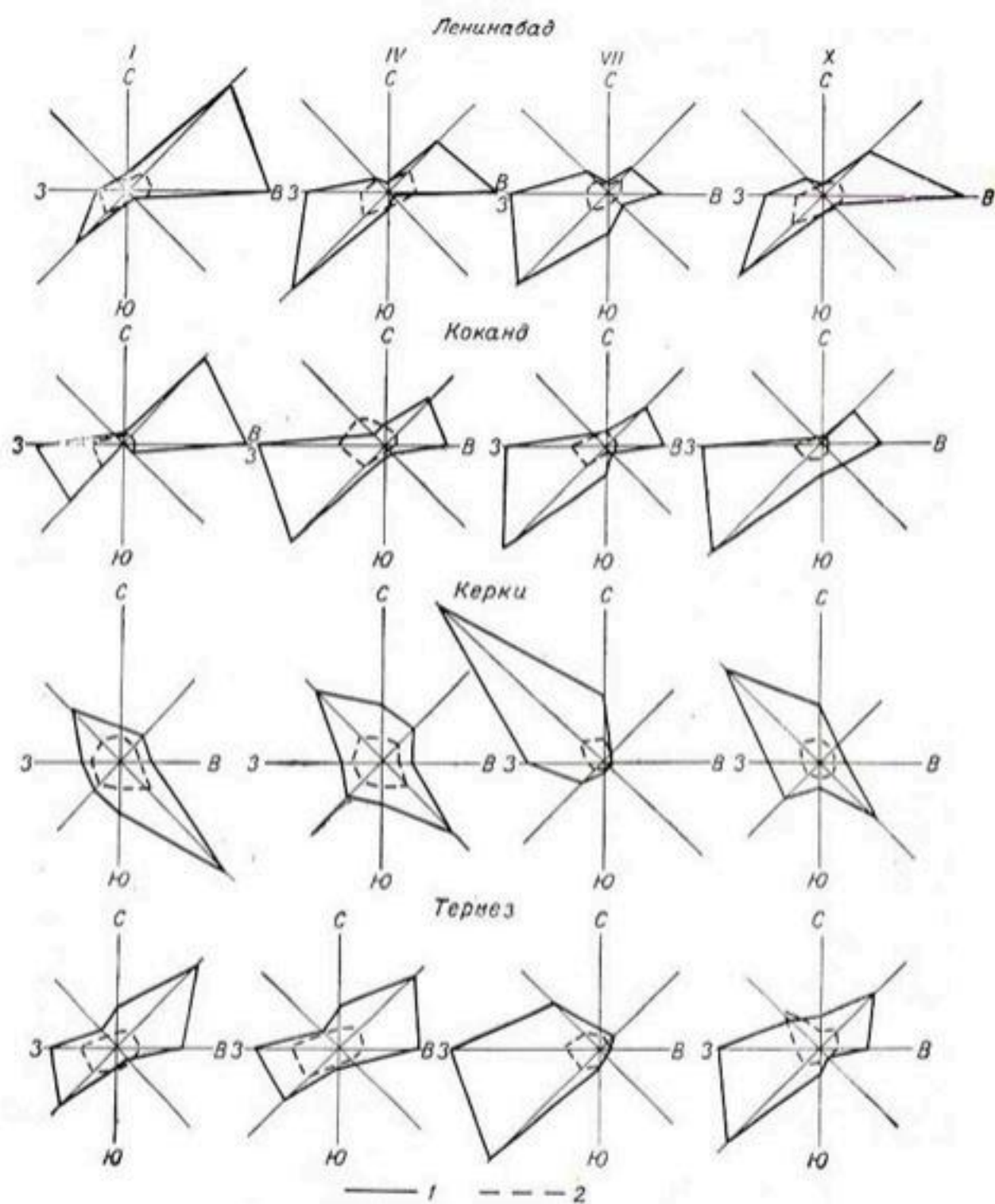
Рис. 39. Направление и скорость ветра. 1 — направление ( ^{\circ}/а ), 2 — скорость (м/сек.).
