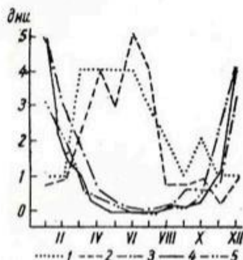
Рис. 83. Годовой ход числа дней с туманами.
