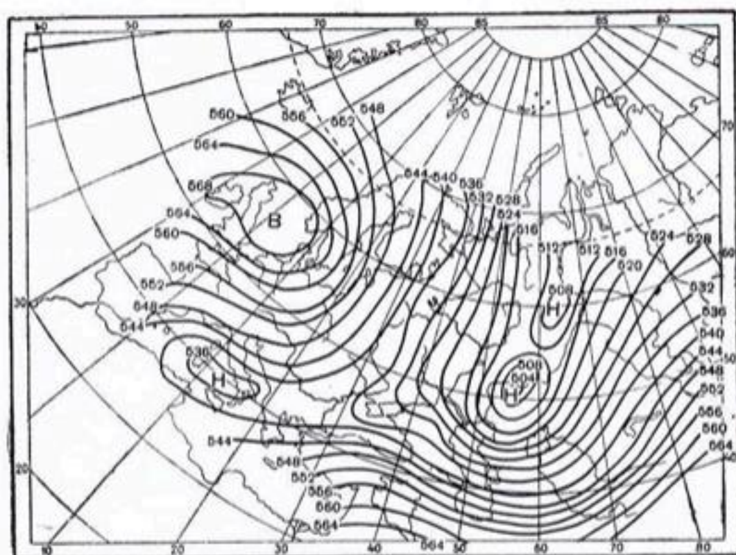
Рис. 18. Карта AT_{500} . 18 час. 20/І 1950 г.
