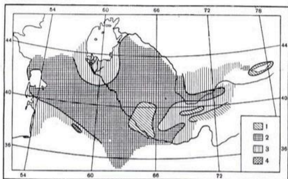
Рис. 82. Годовое число дней с туманами. 1 — 0—10, 2 — 11—20, 3 — 21—45, 4 — более 45 дней.
