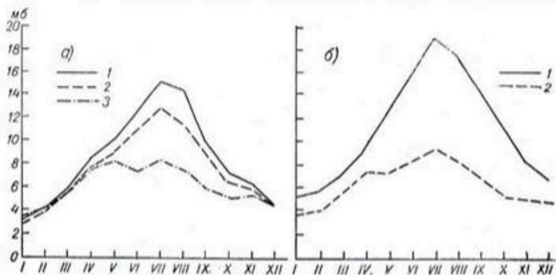
Рис. 64. Годовой ход абсолютной влажности воздуха на равнинах.
