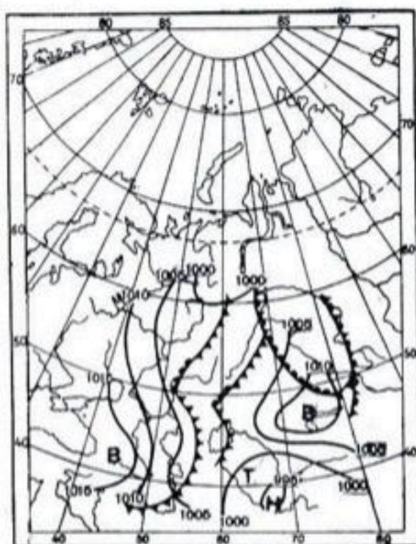
Рис. 20. Карта погоды. 15 час. 21/VII 1948 г.
