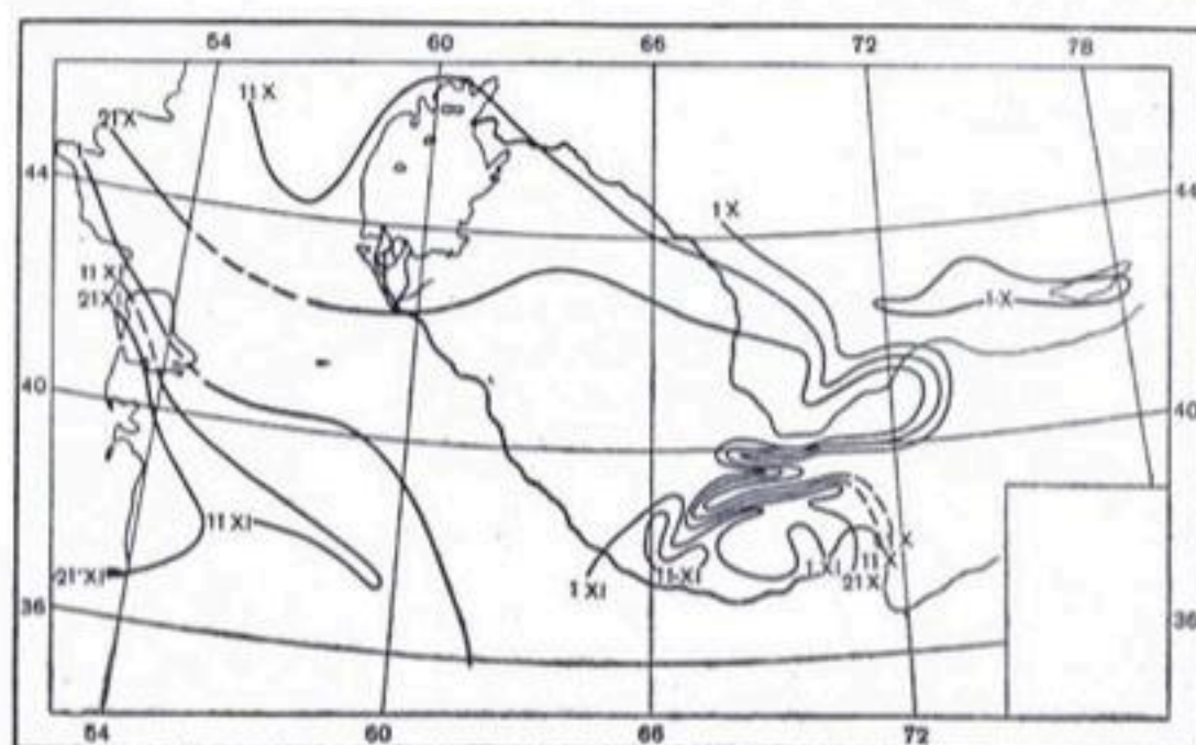
Рис. 59. Средняя дата первого осеннего заморозка.
