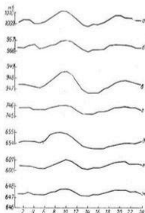
Рис. 34. Суточный ход давления воздуха. Январь.
