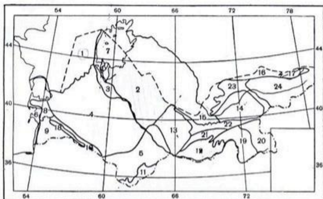
Рис. 93. Схематическая карта климатических районов.
