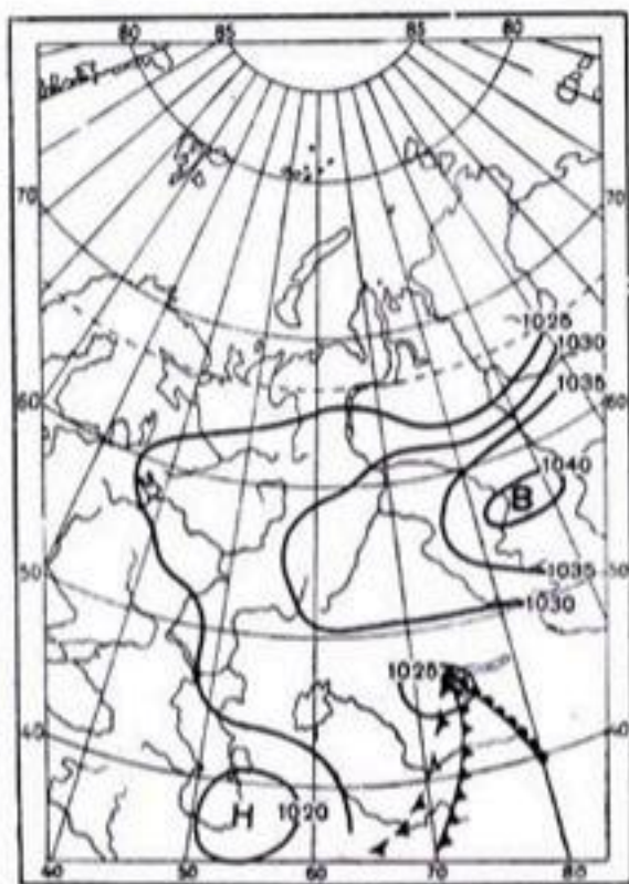
Рис. 86. Карта погоды. 07 час. 15/XII 1939 г.
