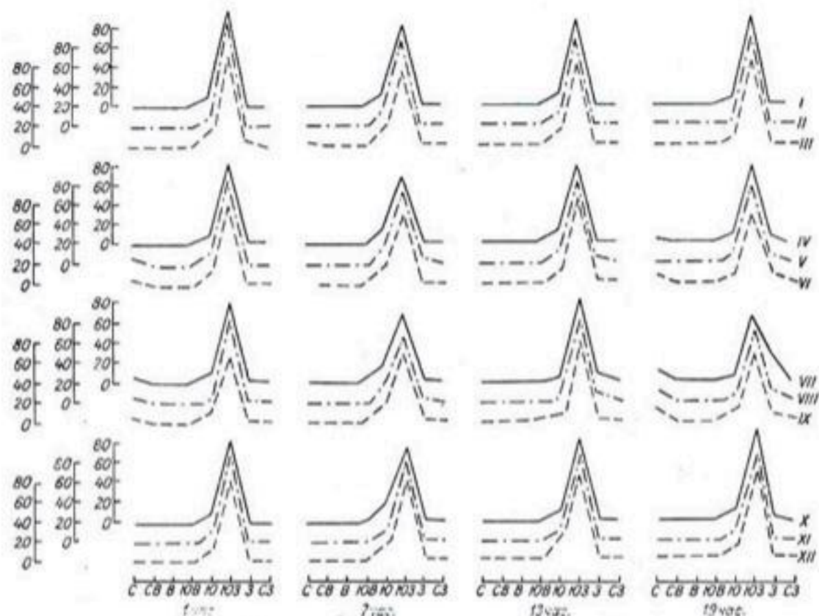
Рис. 50. Годовой и суточный ход ветра (°/в). Ледник Федченко.
