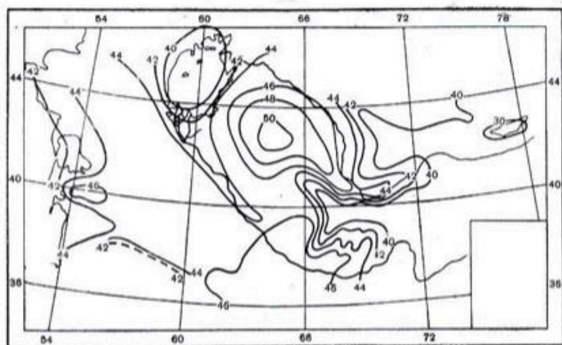
Рис. 55. Абсолютный максимум температуры воздуха (по срочным наблюдениям).
