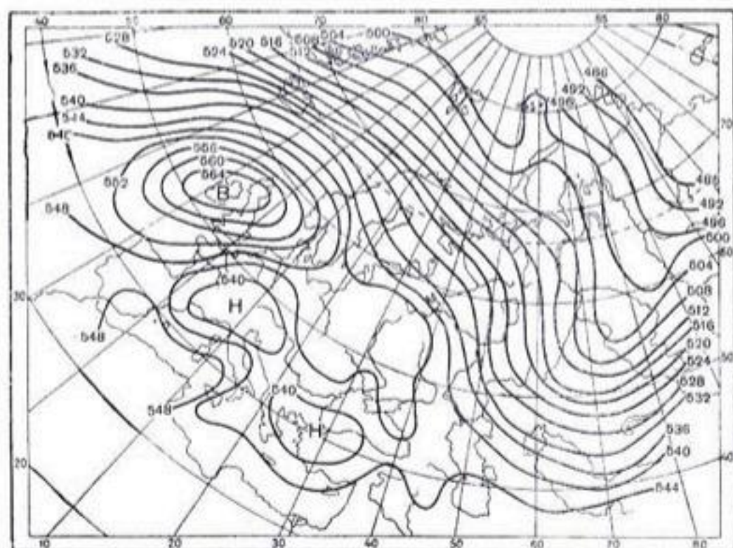
Рис. 16. Карта AT_{500} 17—21/XII 1948 г.
