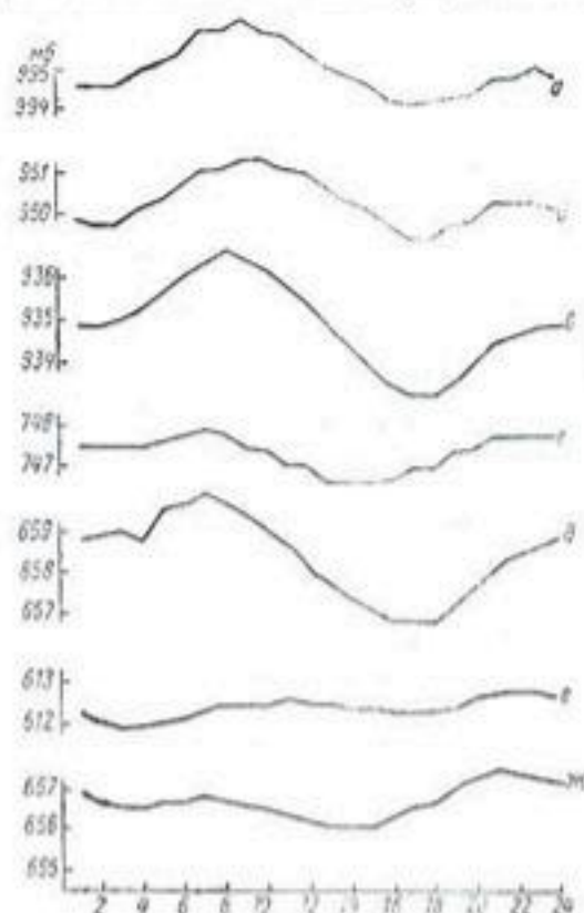
Рис. 35. Суточный ход давления воздуха. Июль.
