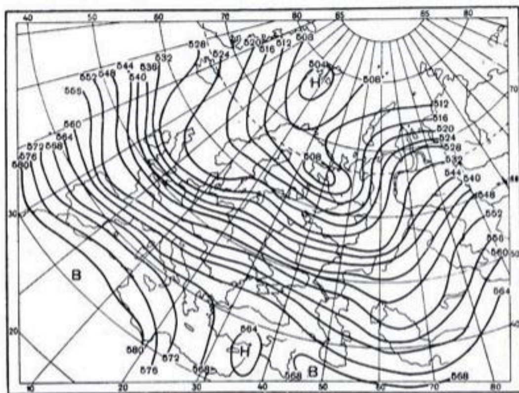
Рис. 14. Карта AT_{500} . 06 час. 19/III 1951 г.
