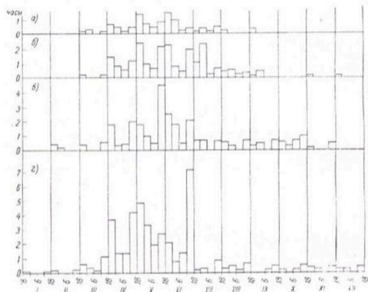
Рис. 91. Продолжительность гроз (часы) в различные интервалы суток. а — Зеагли, б — Ташкент, обсерватория, в — Ашхабад, г — Сталинабад.
