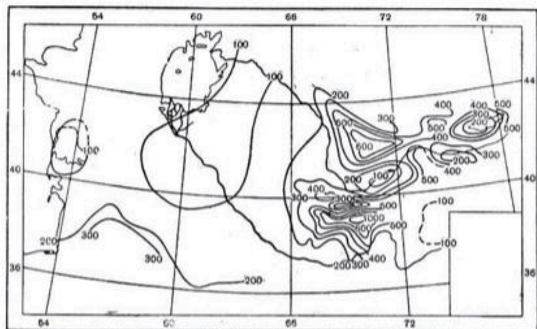
Рис. 72. Количество осадков (мм) за год.
