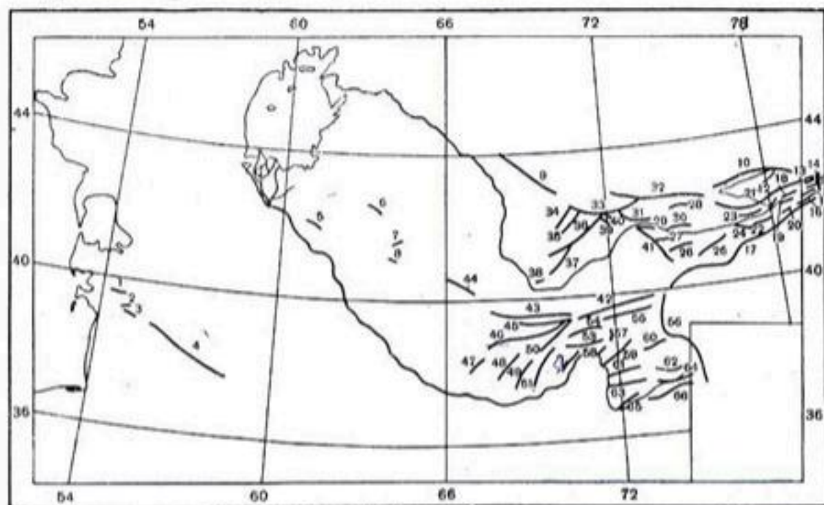
Рис. 1. Схема основных горных хребтов Средней Азии.
