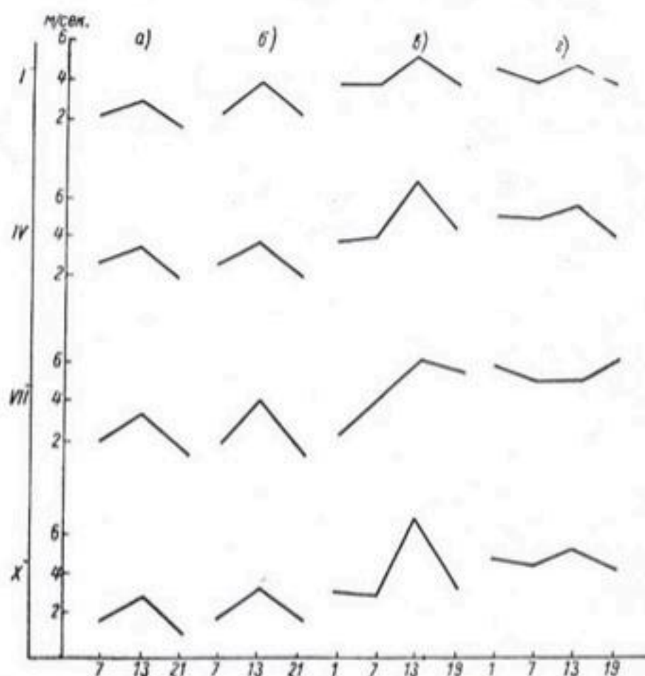
Рис. 37. Суточный ход скорости ветра. а — Турткуль, б — Вайрам-Али, в — Чурук, г — Зеагли.
