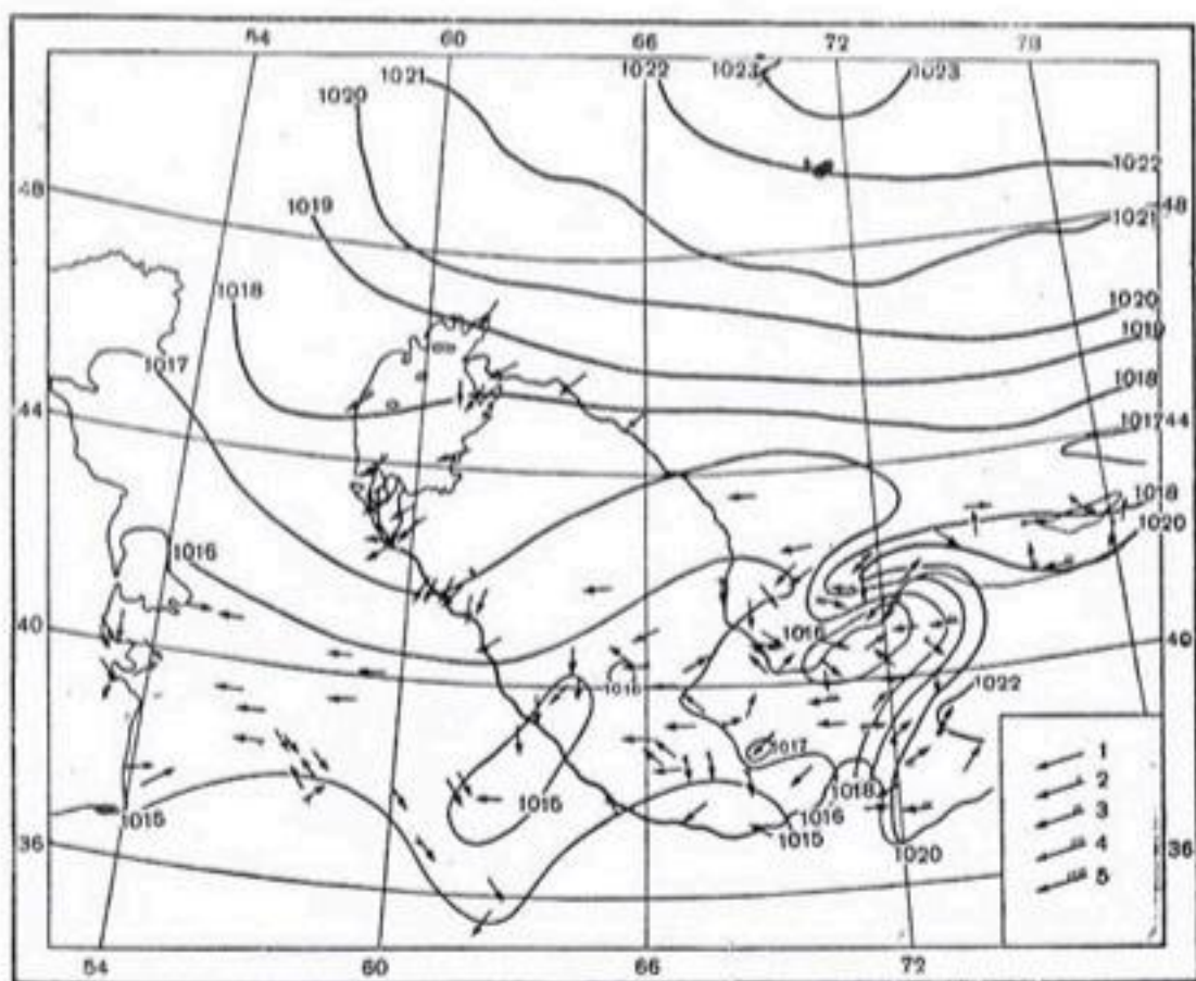
Рис. 30. Давление воздуха на уровне моря и преобладающие направления ветра. Апрель.
