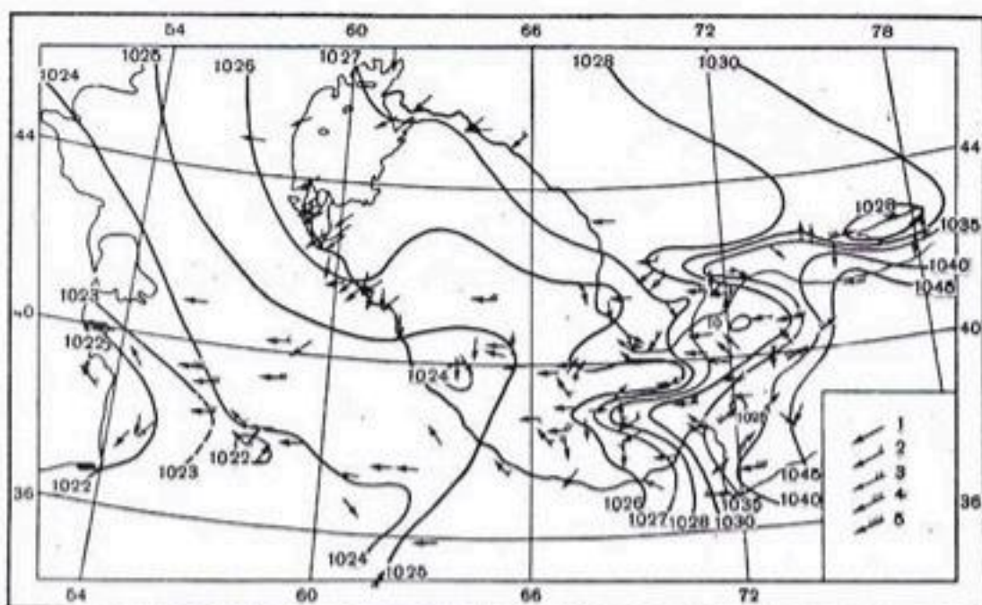
Рис. 29 Давление воздуха на уровне моря и преобладающие направления ветра. Январь.
