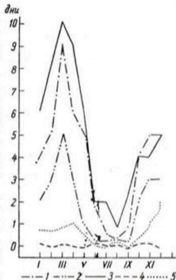
Рис. 84. Годовой ход числа дней с туманами.
