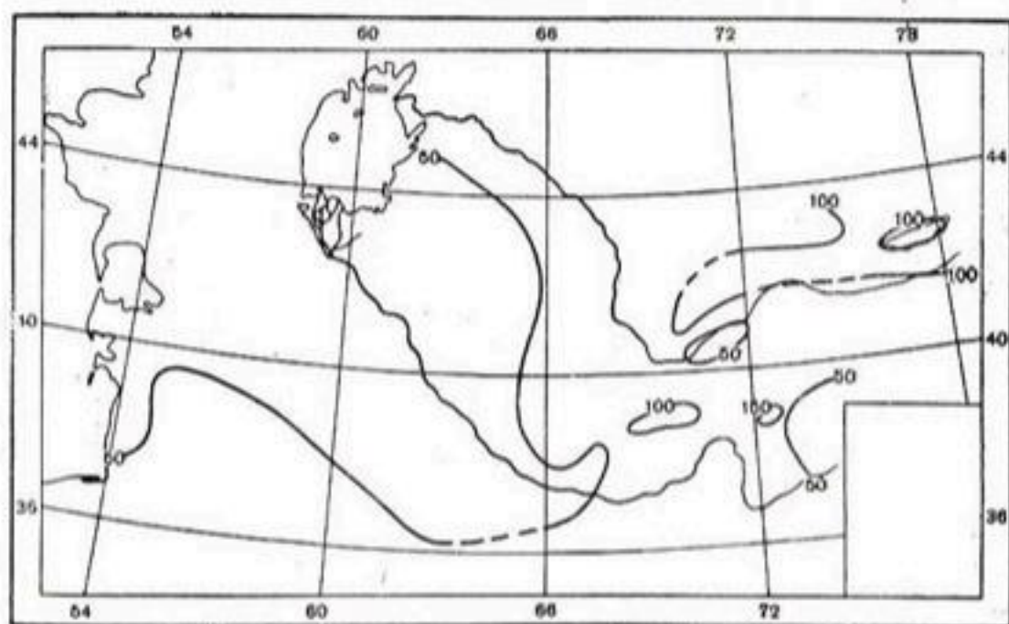
Рис. 77. Среднее годовое число дней с осадками > 0,1 мм.
