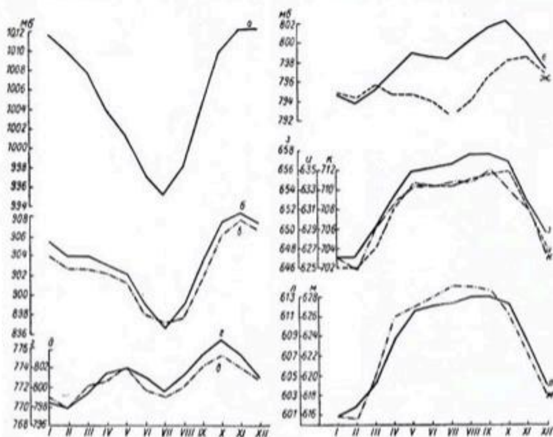
Рис. 33. Годовой ход давления воздуха.
