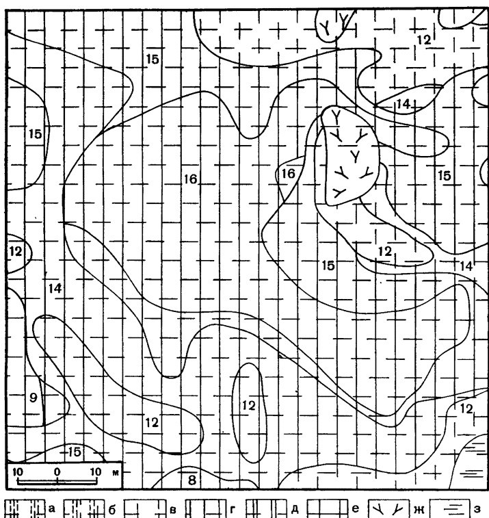
Рис. 1. Почвенный покров холма моренного рельефа Жемайтйской возвышенности
