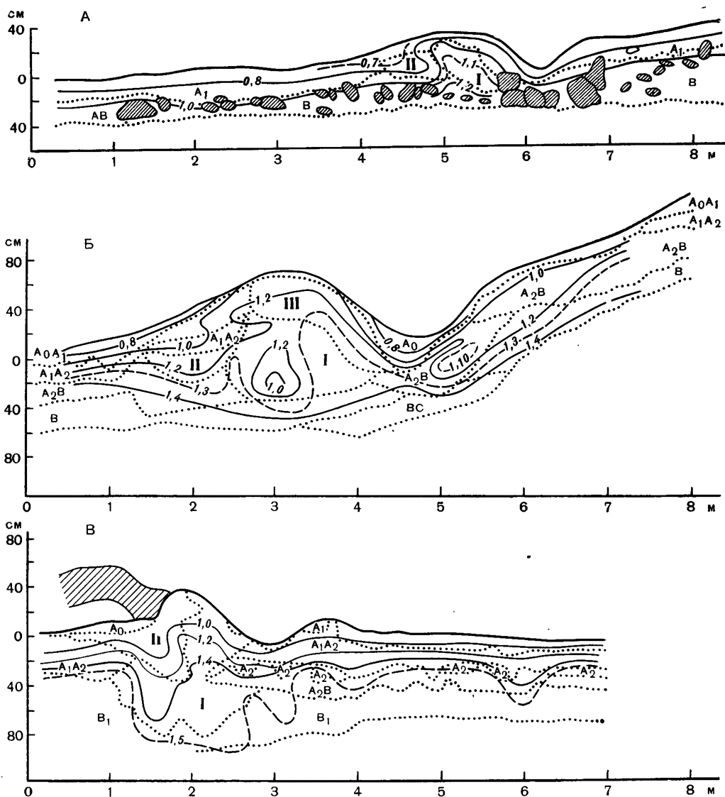
Рис. 2. Распределение ОБ в вывалах
