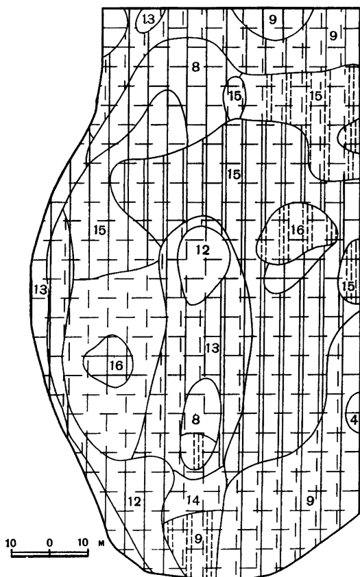
Рис. 1. Почвенный покров холма моренного рельефа Жемайтйской возвышенности
