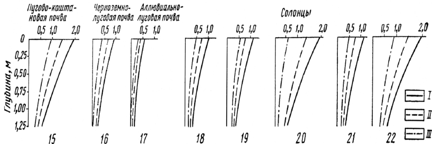
Рис. 6. Прогноз вторичного засоления почв в зоне орошения Северо-Крымского канала при отрицательном водном балансе ( V_1 - U_2 = 0,00027 м в сутки; грунтовые воды расходуются на испарение: D^* = 0,00086 м 2 в сутки). Варианты прогноза: I – грунтовые воды не разбавлены; II – грунтовые воды разбавлены на 1/4 ; III – грунтовые воды разбавлены на 1/2 . Номера ключевых участков от 1 до 22, их местоположение:
