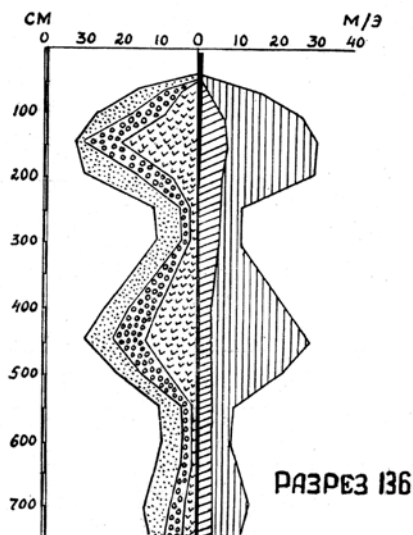
Рис. 18. Солевой профиль степного солончаковатого солонца высокого Присивашья.
