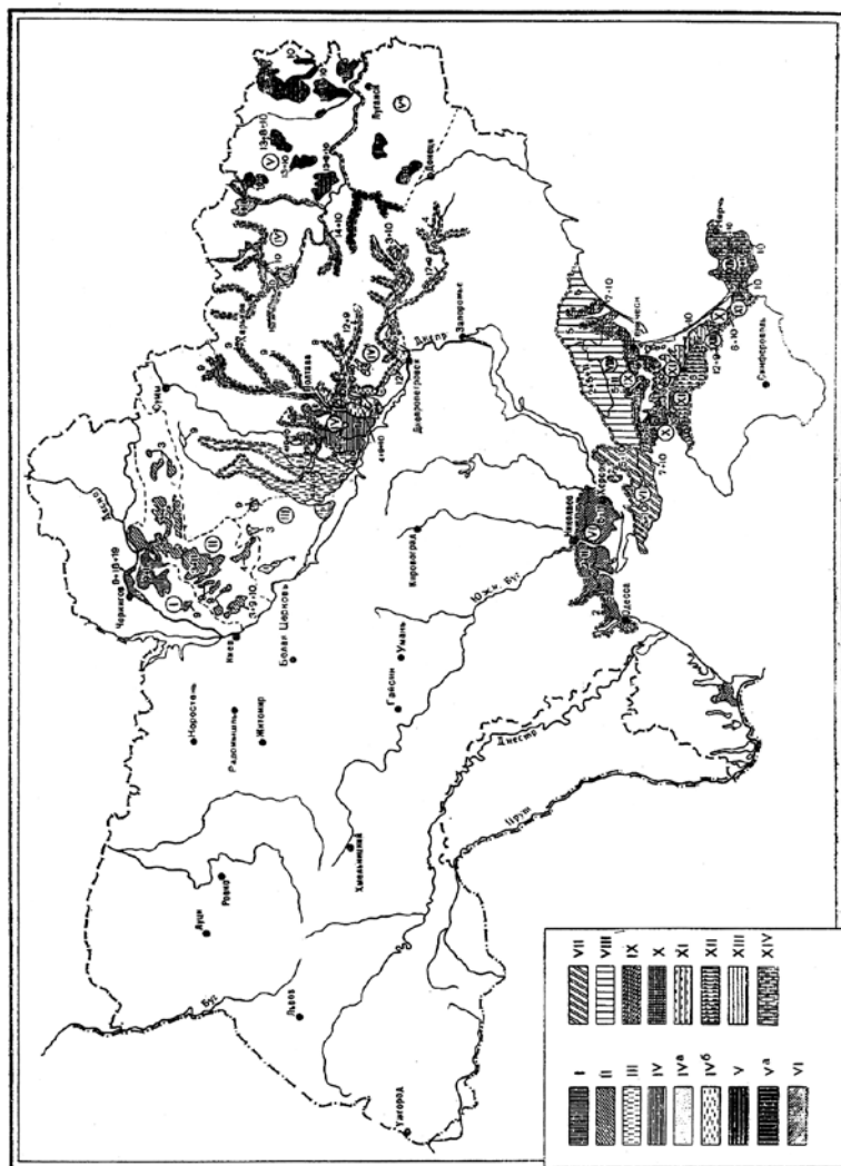
Рис. 1 Картосхема районов распространения и присмов улучшения солонцовых почв УССР (составила А. В. Новикова, редактор Н. К. Крупский).
