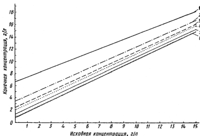
Рис. 5. График зависимости конечной концентрации растворов от исходной их концентрации при различном отношении твердой и жидкой фаз в водной суспензии. Составила А.В. Новикова. Отношение твердой фазы к жидкой в водной суспензии: 1 — 1 : 1; 2 — 1 : 3; 3 — 1:5; 4 — 1 : 10; 5 — 1 : 20; 6 — 1 : 50.
