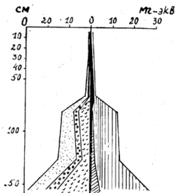
Рис. 10. Солевой профиль лугового солончаковатого солонца низменного побережья Сиваша. Разрез 124. Совхоз «Молодая гвардия»
