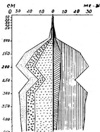
Рис. 14. Солевой профиль лугово-степной темно-каштановой солонцеватой почвы слабоприподнятого Присивашья. Разрез 119. Совхоз «Молодая гвардия» Азовского района.
