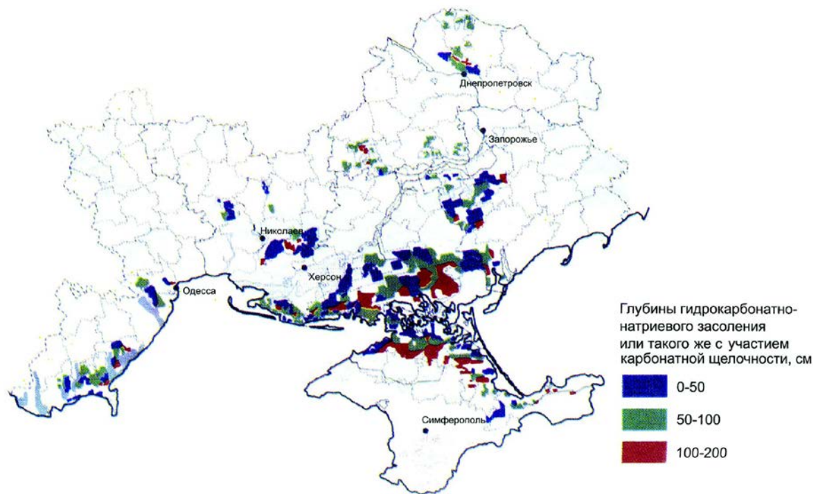
Рис. 2 – Картосхема глубин залегания соды в почвах юга Украины при орошении
