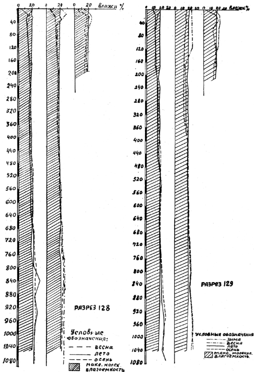
Рис. 4. Динамика влажности степного солонча.
