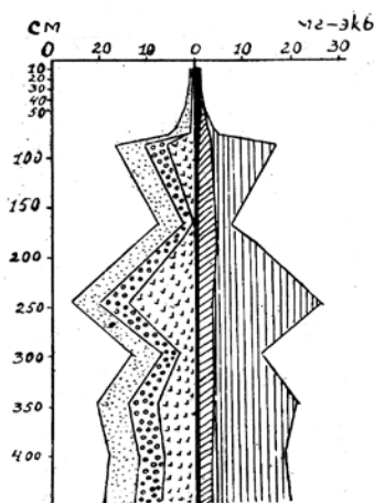
Рис. 12. Солевой профиль лугово-степного глубокосолон- чаковатого солонца слабопри- плоднотого Присивацья. Разрез 117.
