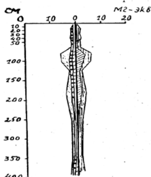
Рис. 16. Солевой профиль лугово-каштановой осолоделой почвы. Разрез 139, с. Будановка Красно-Перекопского района.
