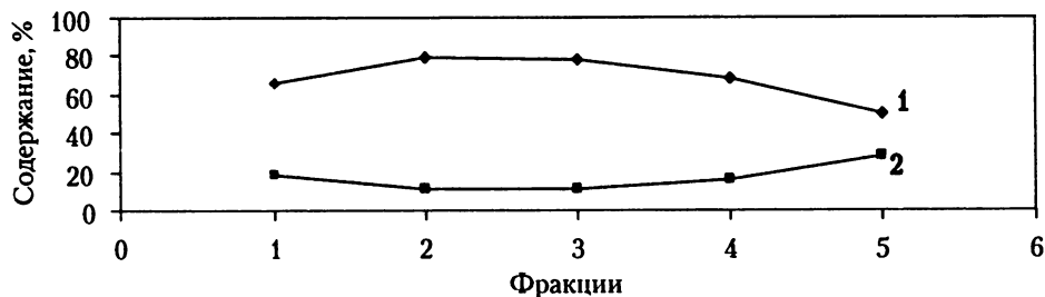
Рис. 9.1. Содержание SiO 2 (1) и R 2 O 3 (2) в гранулометрических фракциях: 1 – песок; 2–4 –пыль: 2 – крупная, 3 – средняя, 4 – мелкая; 5 – ил
