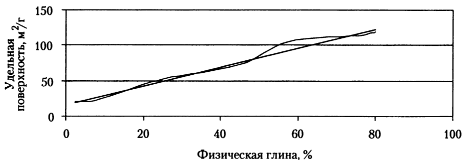
Рис. 2.1. Зависимость удельной поверхности горной породы от содержания в ней физической глины (частиц < 0,01мм)
