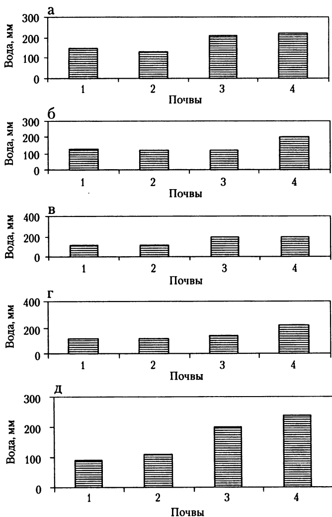
Рис. 6.3. Запасы воды в слое 0–50см разных суглинистых и глинистых почв: а – май, б – июнь, в – июль, г – август, д – сентябрь. 1, 2 – типичный чернозем, дубрава и степь; 3, 4 – краснозем (Чаква, плантации мандарин и чая)
