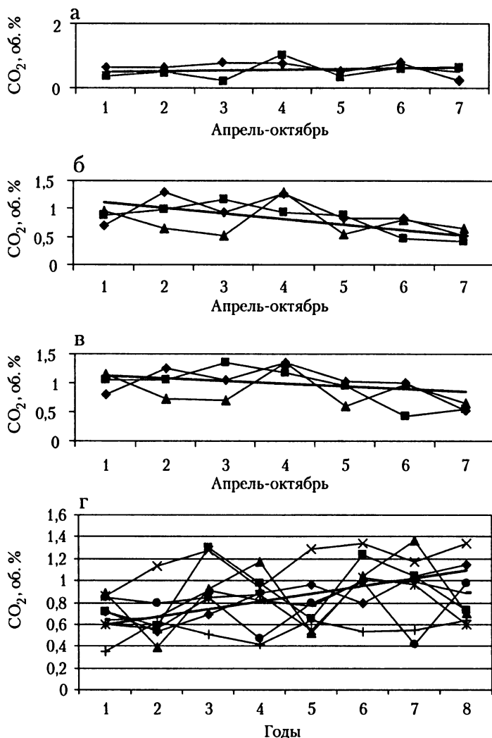
Рис. 8.2. Варьирование содержание \text{CO}_2 в воздухе чернозема обыкновенного в течение года: а – 20, б – 50, в – 70; г – варьирование по годам
