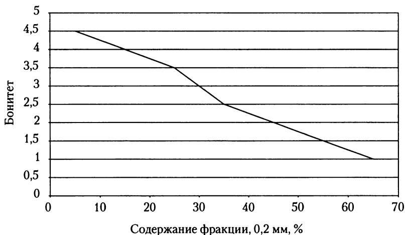
Рис. 4.3. Зависимость бонитета сосны от гранулометрического состава почв
