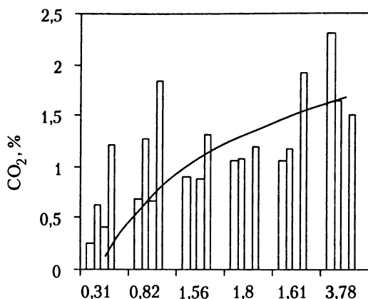
Рис. 8.1. Концентрация CO 2 в почвенном воздухе разных почв
