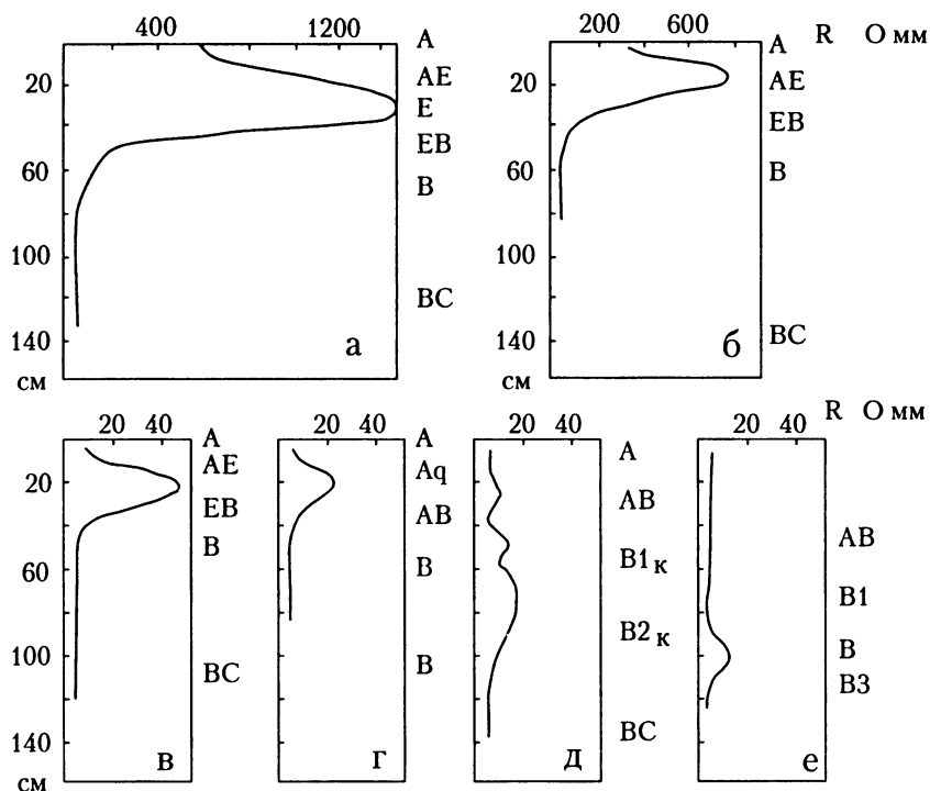
Рис. 4.4. Кривые электрического сопротивления (Ом·м) основных типов почв: а – дерново-подзолистые песчаные; б – дерново-подзолистые суглинистые; в – серые лесные; г – темно-серые лесные; д – черноземы ЦЧО (Курская обл.); е – светло-каштановые (Волгоградская обл.). Справа от колонок – генетические горизонты
