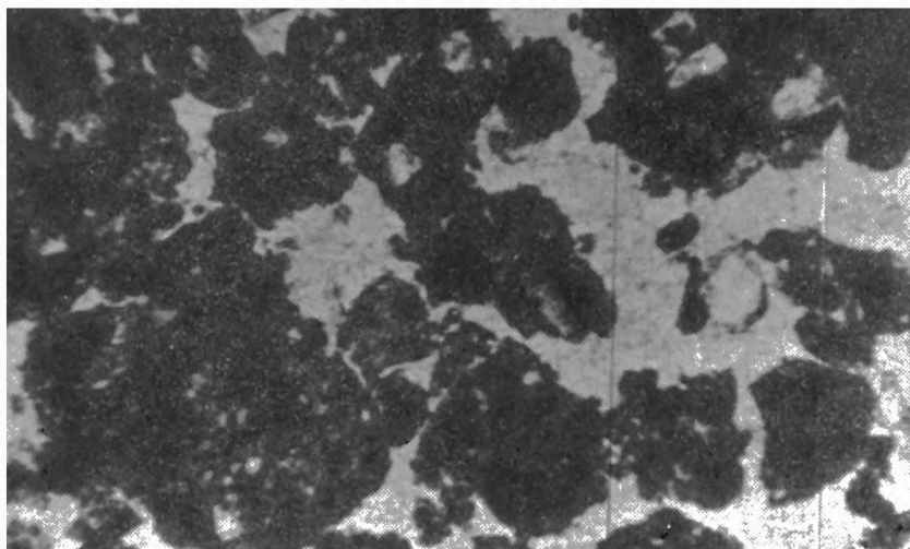
Фото 1. Сложные поры упаковки в горизонте оксид почв энтропс, штат Минас-Жерайс, Бразилия. Па- раллельные николи, ув. 71х.
