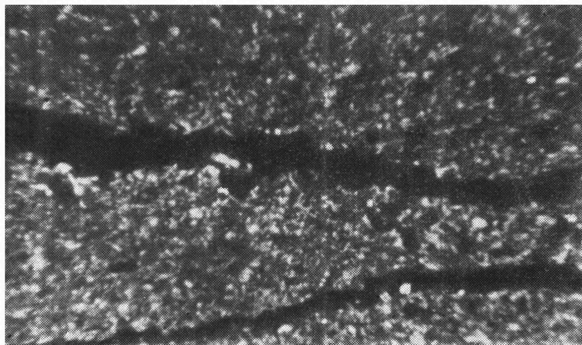
Фото 3. Прямые трещины в поверхностных горизонтах почв торрифлювент, штат Аризона. Скрещенные никколи, ув. 71х.
