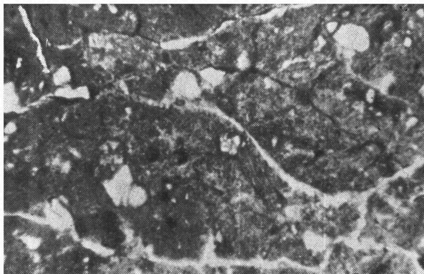
Фото 4. Косые трещины в горизонте аржиллик в почве галларгид, штат Аризона. Параллельные никколи, ув. 71х.
