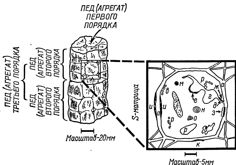
Р и с. 6. Схематическое изображение некоторых микроморфологических признаков.
