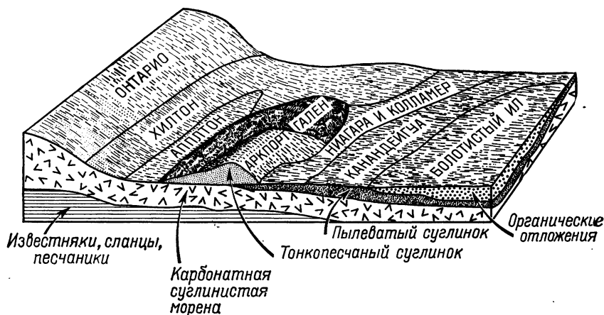
Р и с. 56. Блок-диаграмма почвенных ландшафтов; графство Дженессси, в западной части штата Нью-Йорк (Wulforst, Wertz, Leonard, 1969).
