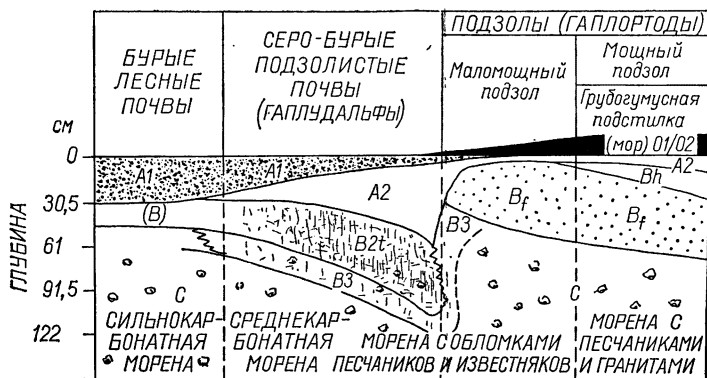
Р и с. 12. Катена бурые лесные почвы — подзолы, штат Нью-Йорк. (См. Cline, 1953).
