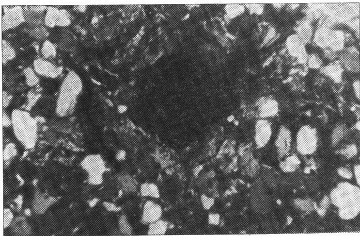
Фото 10. Аржиллан с низкой степенью ориентации на песчаных зернах. Погасание скорее пятнистое, чем отчетливо полосчатое. Скрещенные николи, ув. 71х.
