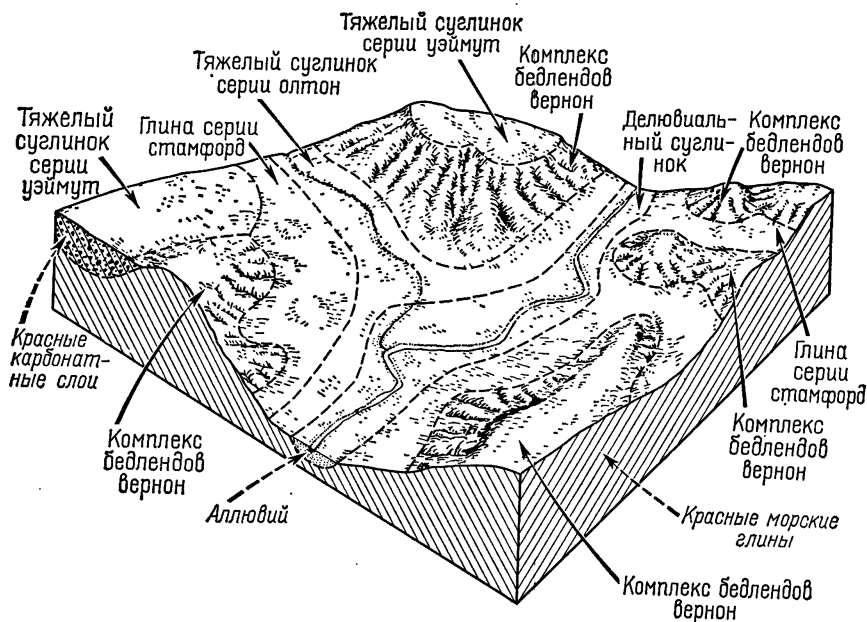
Рис. 29. Блок-диаграмма почвенных ландшафтов в графстве Раннелс; центральная часть штата Техас (Wiedenfeld, Barnhill, Novosad, 1970).
