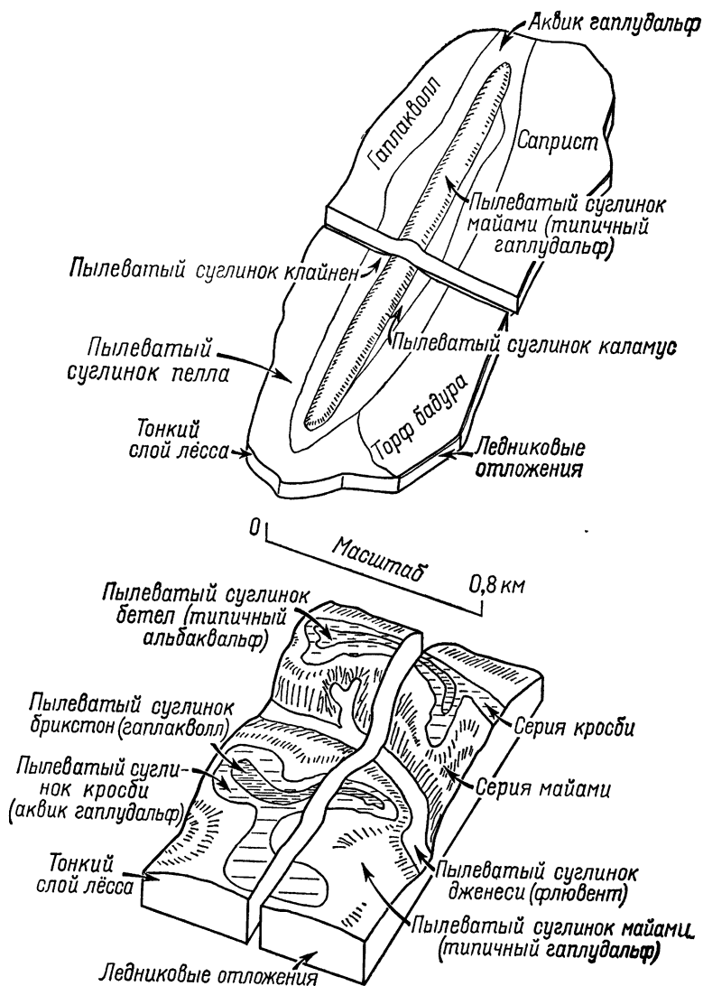
Рис. 59. Различное топографическое положение пылеватых суглинков Майами — типичного гajлудальфа в южной части Висконсина (Hole, Lee, Grisbauer, 1953) и на востоке центральной части штата Индиана (Bushnell, 1930).
