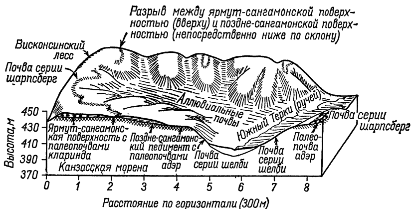
Р и с. 24. Блок-диаграмма части территории ручья Терка, графство Адэр, штат Айова, иллюстрирующая положение почв на разных элементах рельефа. (Обобщено по картам и рисункам — Ruhe, Daniels, Cady, 1967.)
