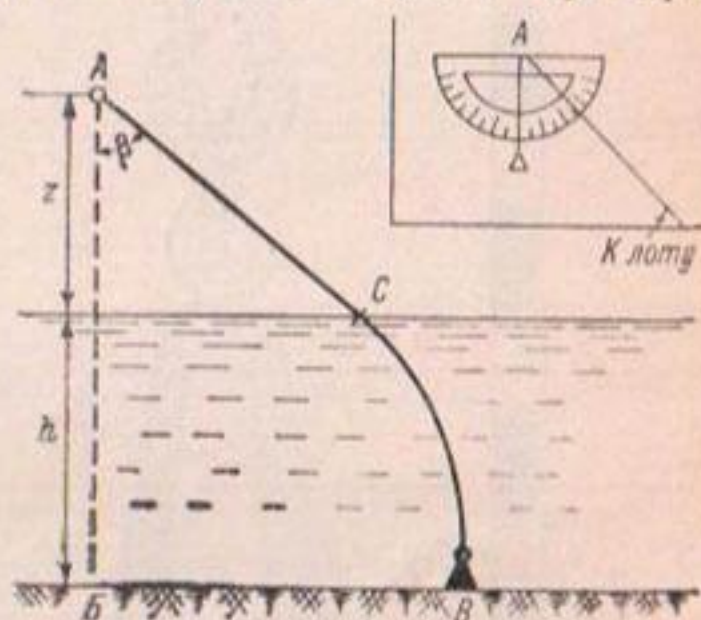
Рис. 104. Относ лота.
