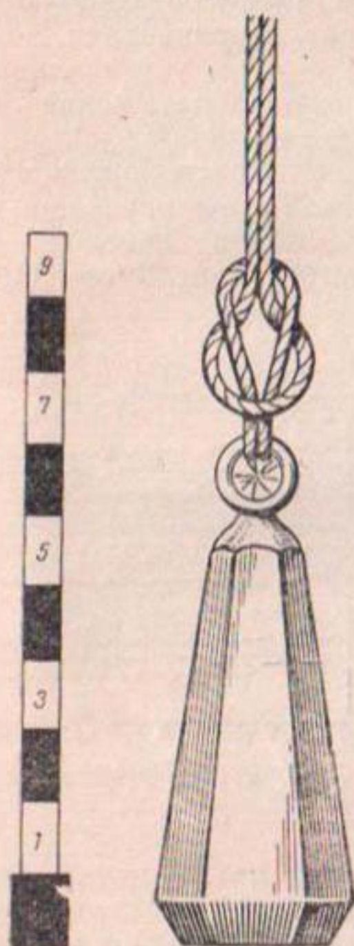
Рис. 100. Наметка. Рис. 101. Лот.
