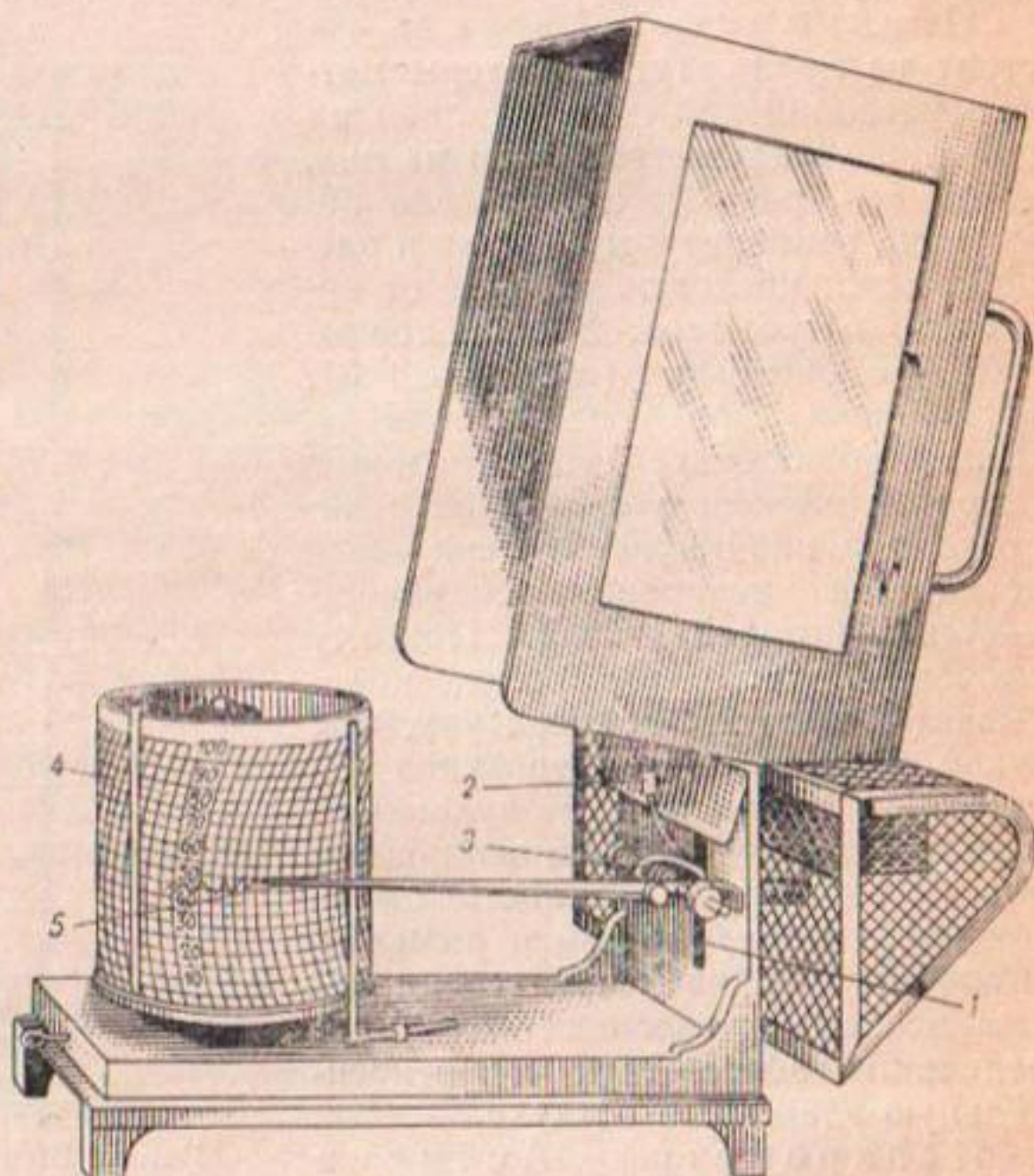
Рис. 8. Гигрограф.
