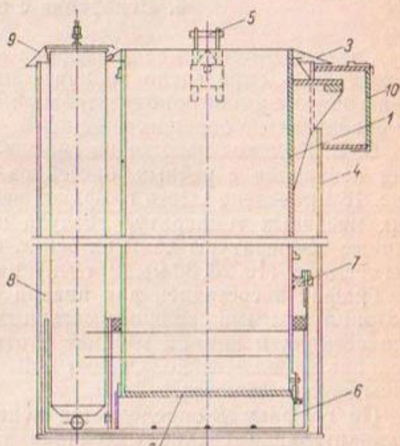
Рис. 13. Лизиметр ГР-80.
