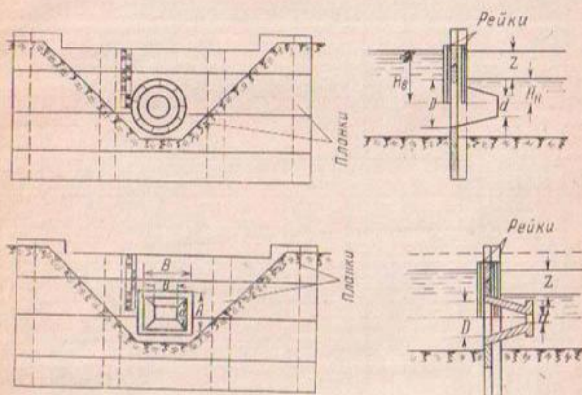
Рис. 142. Насадки-водомеры
