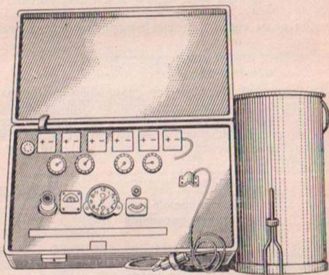
Рис. 124. Измеритель расхода воды ИРВ-52.
