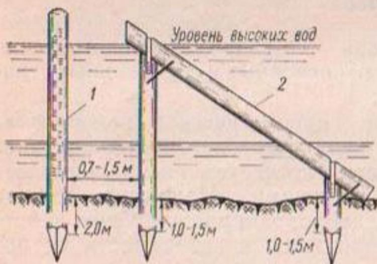
Рис. 80. Речной водомерный пост. 1 — рейка укреплена на свае; 2 — ледорез для защиты рейки от плавающих предметов.
