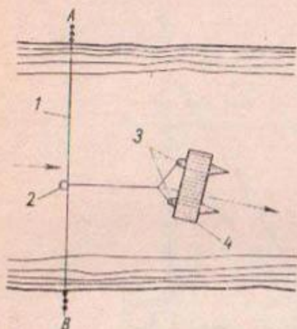
Рис. 94. Паром-самолет.
