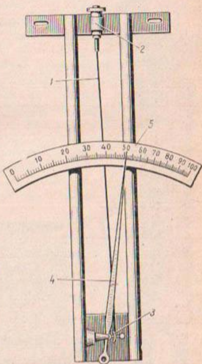
Рис. 6. Волосной гигрометр.
