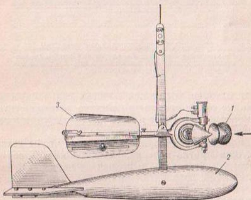
Рис. 118. Вертушка ИВХ.
