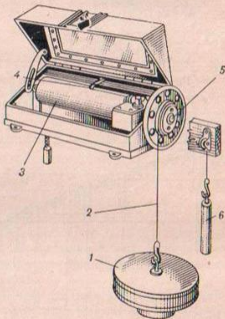
Рис. 85. Самонисец уровня «Валдай». 1 — пустотелый поплавок; 2 — провод; 3 — барабан; 4 — каретка с пером; 5 — ко- лесо; 6 — противовес.
