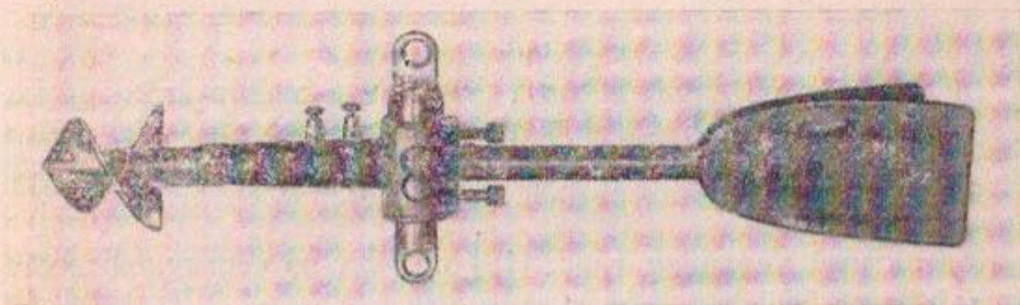
Рис. 117. Вертушка ВБ-61.
