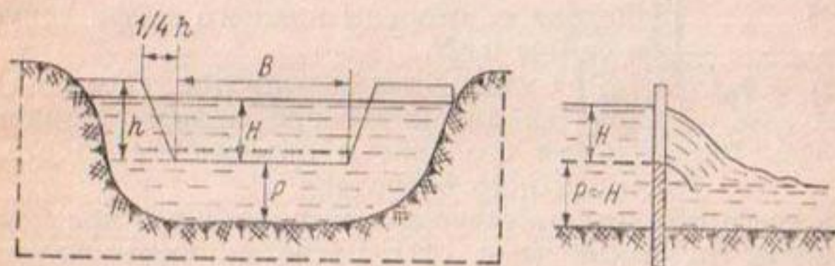
Рис. 140. Трапецеидальный водослив.
