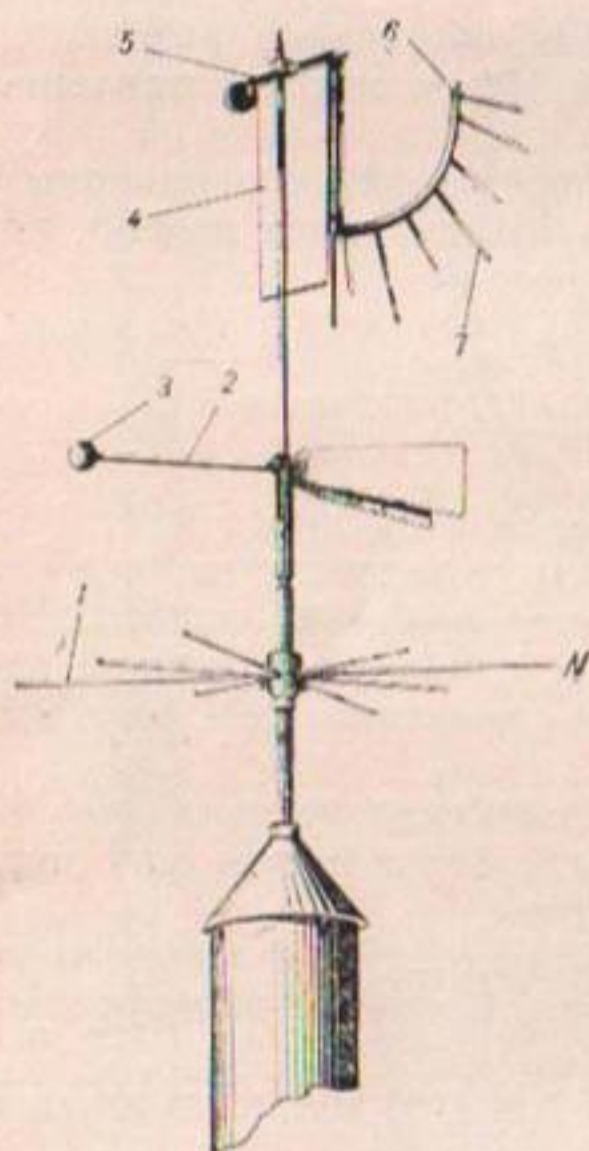
Рис. 29. Флюгер Вильда.
