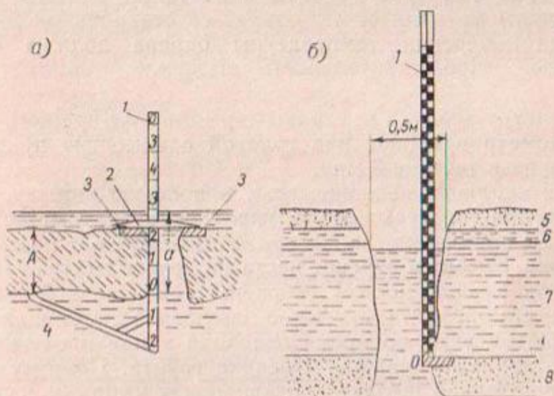
Рис. 95. Ледомерные рейки.
