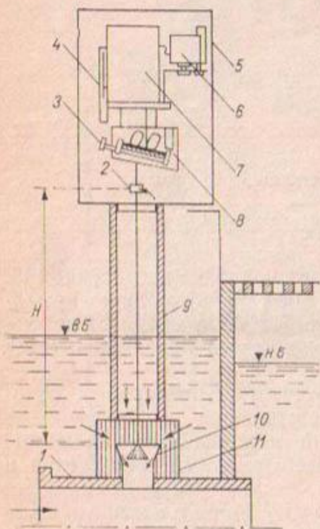
Рис. 148. Многопредельный расходоуказатель ДРС-66.
