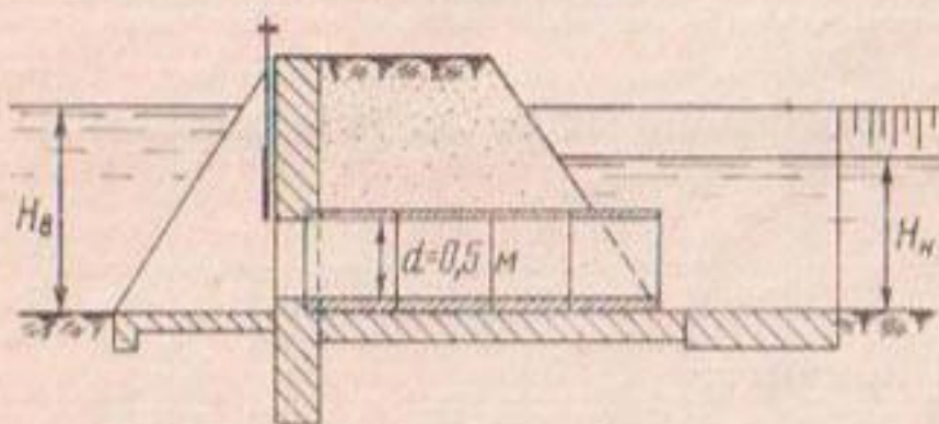
Рис. 149. Трубчатый водовыпуск.
