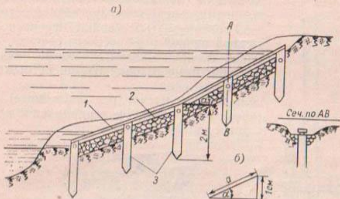
Рис. 82. а — схема установки наклонной рейки. 1 — наклонная рейка, 2 — щебенчатая подготовка, 3 — свая. б — расчет делений наклонной рейки.
