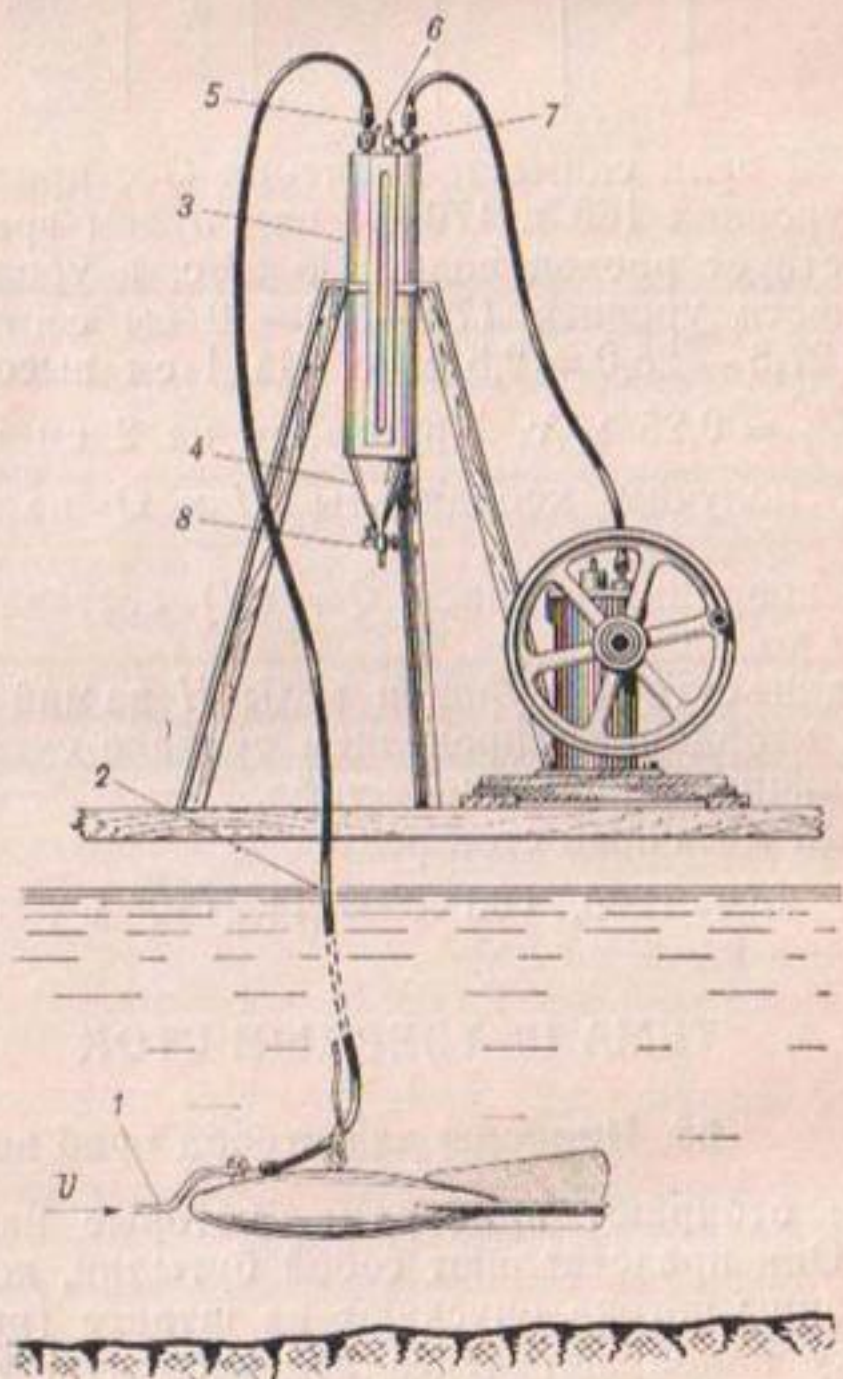
Рис. 134. Вакуумный батометр.
