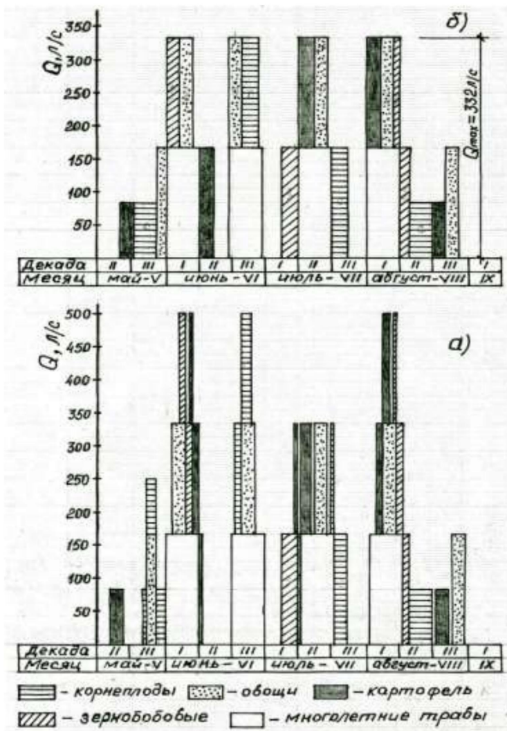
Рис. 2.4 Графики водоподачи на орошение овощекормового севооборота дождеванием ДКШ-64А: а) неукomплектованный; б) неукomплектованный
