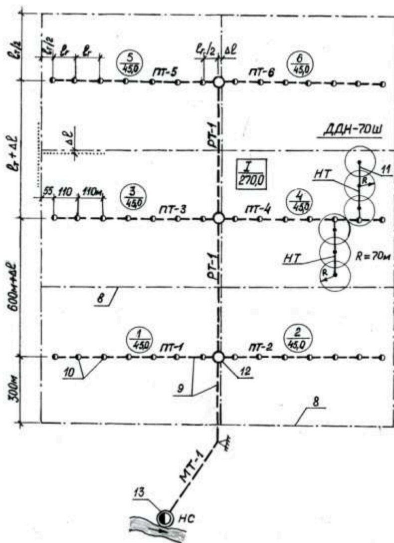
Рис. 3.1 Схема оросительной сети при орошении дождеванием ДДН-70Ш (I-й вариант сети)
