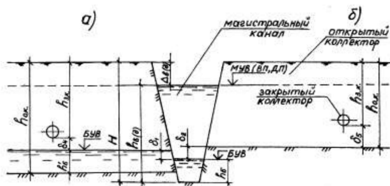
Рис. 6.5 Схема вертикального сопряжения к определению глубины проводящей осушительной сети:
