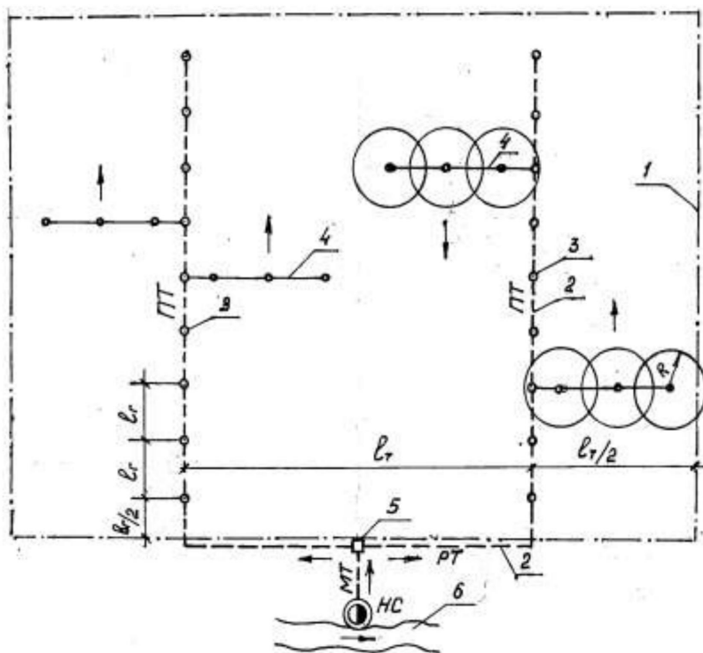
Рис.1.2.1 Схема орошения дождевальными агрегатами: ДДН-70Ш, ДДН-100Ш, ДДН-150Ш
