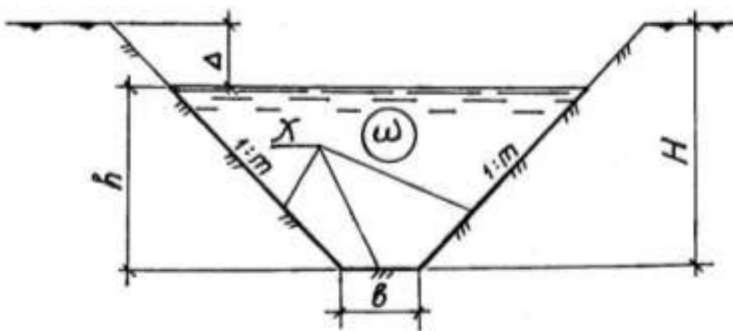
Рис.6.2 Параметры поперечного сечения канала
