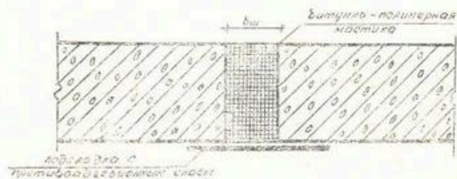
Рис. 5. Шов, герметизированный битумно-полимерной мастикой
