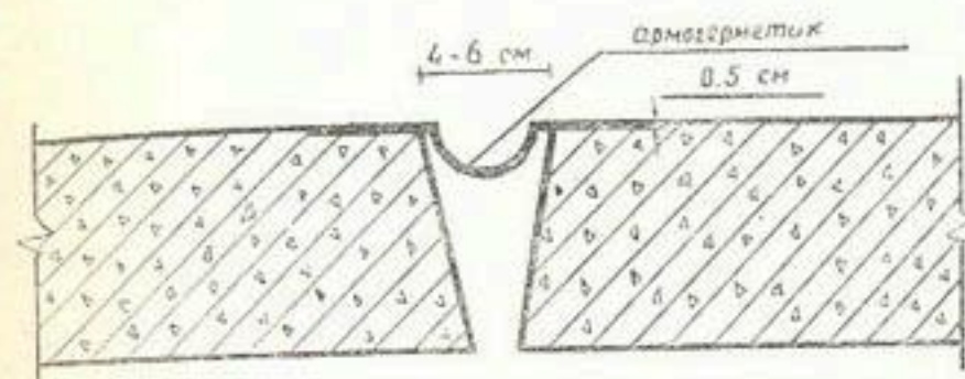
Рис. 7. Шов, герметизированный армогерметиком.
