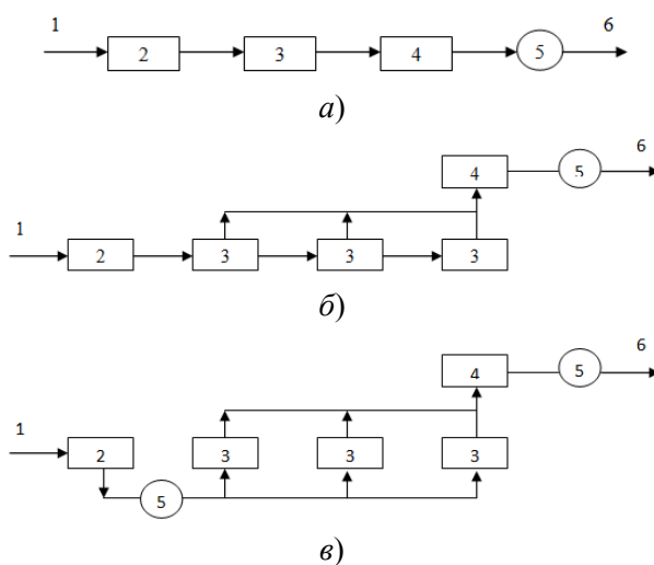
Рисунок 2 – Технологические схемы очистки дренажных вод
