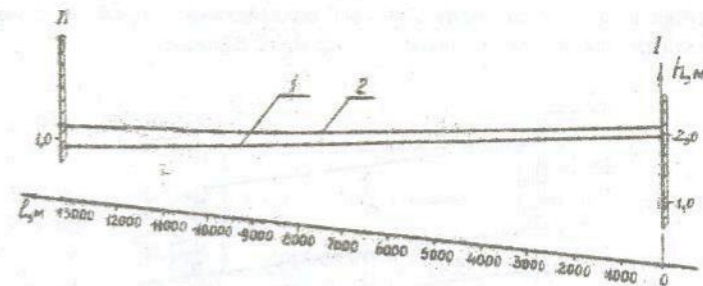
Рис.5. Кривые подпора воды в звене каскада: 1 - одновременное уменьшение расхода в начальном и конечном створах; 2 - уменьшение расхода в конечном створе и увеличение в начальном створе.
