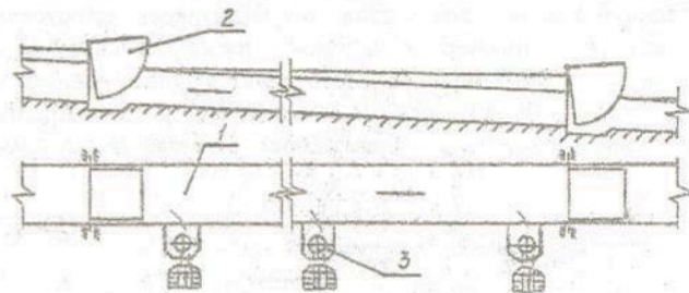
Рис.1. Компонентная схема участка канала системы водораспределения при каскадном регулировании с гидравлическими стабилизаторами расхода воды: 1-транзитный канал; 2-регулятор УНБ с защитой от переполнения канала; 3-водовыпуск, автоматизированный стабилизатором расхода воды.
