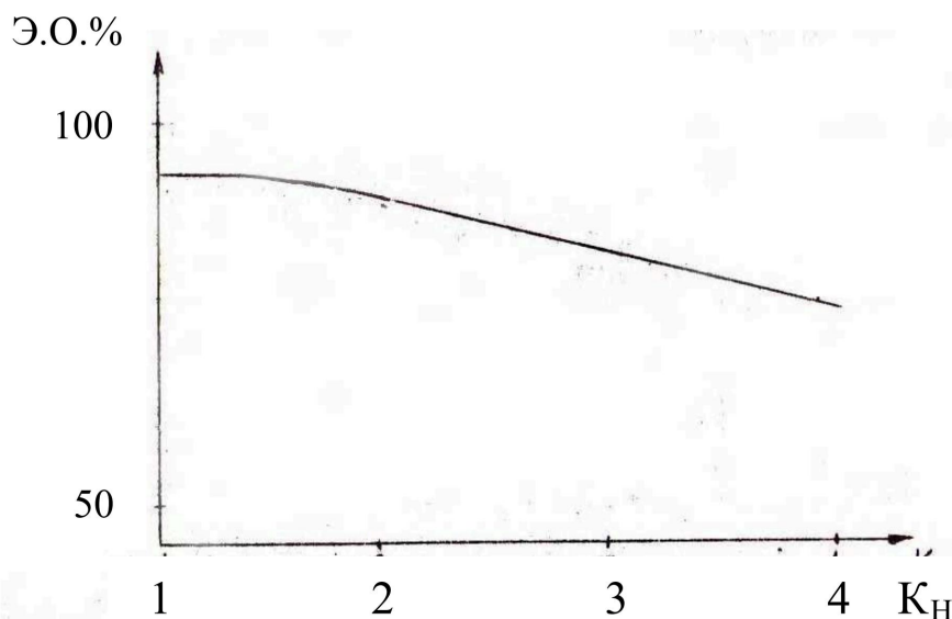
Рис.3.25. Зависимость эффекта биологической очистки (Э.О.) от коэффициента неравномерности ( K_n ): коэффициент неравномерности – отношение максимального количества примесей к среднему количеству примесей, поступающих со сточной водой в систему биологической очистки.
