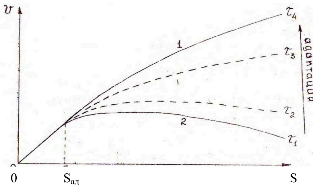
Рис.3.26. Зависимость скорости очистки ( v ) от концентрации примесей ( S ) сточной воды: 1- после завершения адаптационной перестройки биоценоза; 2- сразу после изменения концентрации примесей (без адаптации); S_{ag} - исходная концентрация примесей, к которой был адаптирован биоценоз до изменения режима; \tau - период адаптации ( \tau_1 = 0; \tau_4 > \tau_3 > \tau_2 > \tau_1 )
