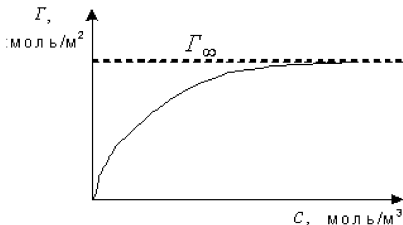
Рис. 3.14. Изотерма адсорбции
