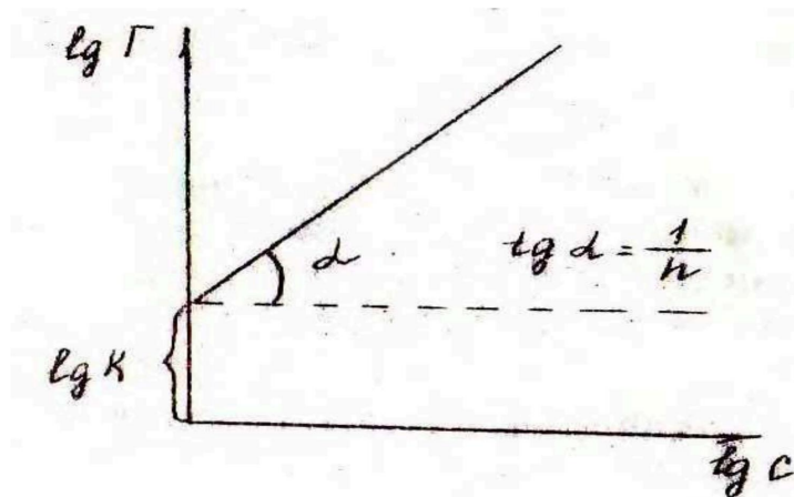
Рис.3.16. Изотермы адсорбции Фрейндлиха в двойном логарифмическом масштабе
