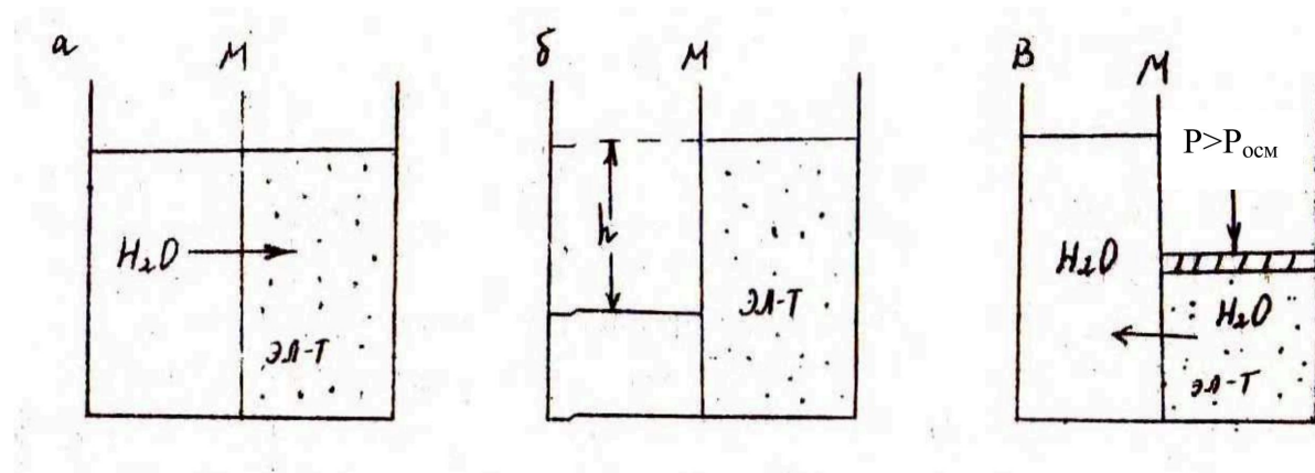
Рис.3.23 Схема возникновения осмотического давления и обратного осмоса: а – исходная система; б – равновесная система; в – обратный осмос.
