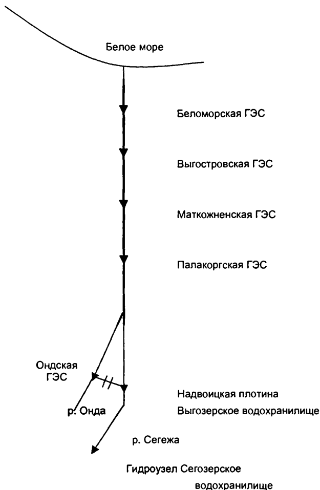
Рис. 3.3. Схема водохранилищ Выгского каскада ГЭС на р. Нижний Выг.
