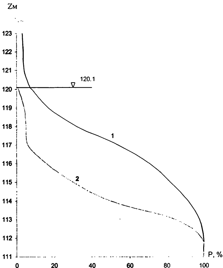
Рис. 4.2. Кривые продолжительности ежедневных уровней воды у г. Сунтар (588 км от ГЭС) на р.Вилуй с 1.06 по 20.06 1 – естественные, 2 – зарегулированные, \nabla – отметка выхода воды на пойму
