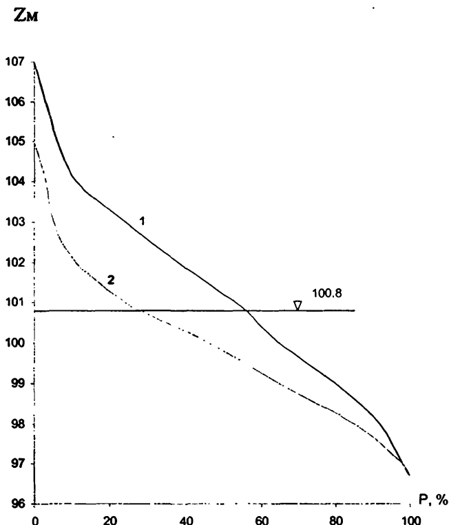
Рис. 4.3. Кривые продолжительности ежедневных уровней воды у с.Верхне-Вилуйск (896 км от ГЭС) на р.Вилуй с 1.06 по 30.06. 1 – естественные, 2 – зарегулированные, ▽ – отметка выхода воды на пойму
