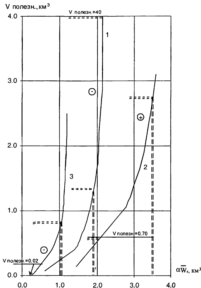
Рис.3.4. Кривые зависимости гарантированной водоотдачи ( a\overline{W}_r ) от полезного объема водохранилища ( V )
