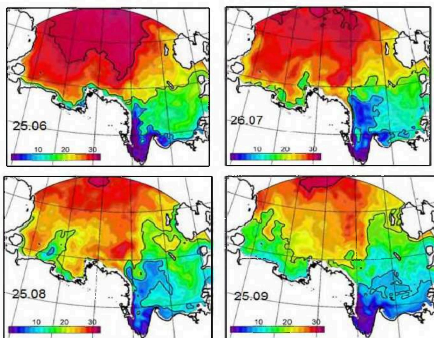
Рис. 3. Распространение пресных вод р. Лены. Распределение солёности в поверхностном слое восточной части моря Лаптевых в летний период 2008 г. Модельный расчет
