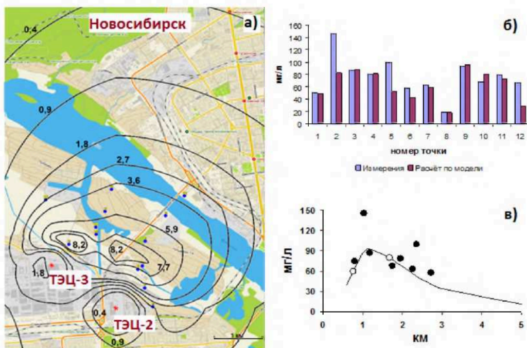
Рис. 4. Восстановленное суммарное поле выпадений пыли в снеге от ТЭЦ-2 и ТЭЦ-3 Новосибирска ( \text{г}/\text{м}^2 ) (а); измеренная и вычисленная концентрации пыли в точках отбора проб (б); восстановленная концентрация пыли в северо-восточном направлении от ТЭЦ (в); обозначения: \circ – опорные точки, \bullet – контрольные точки наблюдений, * – положение источников
