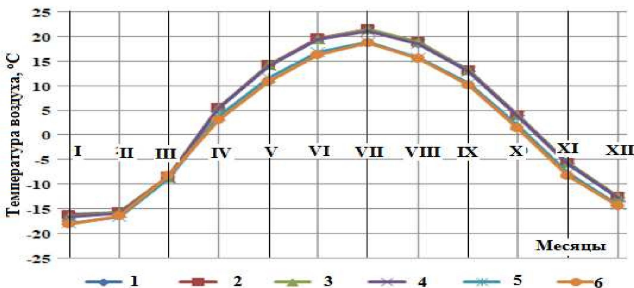
Рисунок 4 – Внутригодовые изменения температур воздуха в водосборных территориях бассейна реки Тобыл (1 – Костанай; 2 – Рудный; 3 – Лисаковский; 4 – Тобыл; 5 – Курган; 6 – Ялуторовск)
