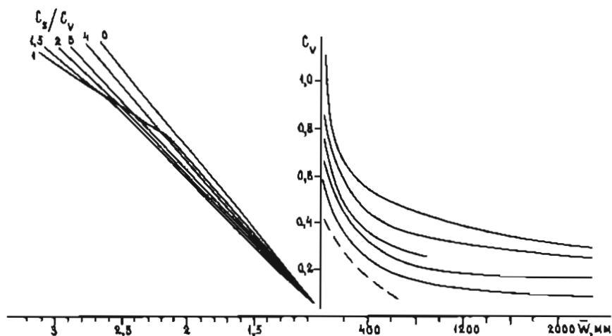
Рис. 16.3. Номограмма для расчета модульных коэффициентов снеговых нагрузок 5%-ной обеспеченности по трем статистическим параметрам - норме максимальных снегозапасов W , коэффициенту вариации C_v и асимметрии C_u ; для гор Сьерра Невада, 40-490 с.ш.; Скалистых гор, 35-390, 40-490, 50-590 с.ш.; северной части Берегового хребта, хр. Брукса и гор Маккензи
