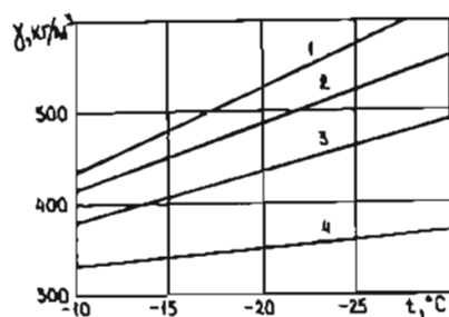
Рис.15.1. Зависимость плотности снега \gamma от температуры воздуха t и уплотняющих средств: 1 - вибратор массой 1,6 \text{ т} , 2 - вибратор 0,6 \text{ т} , 3 - каток с уплотнителем, 4 - каток без уплотнителя
