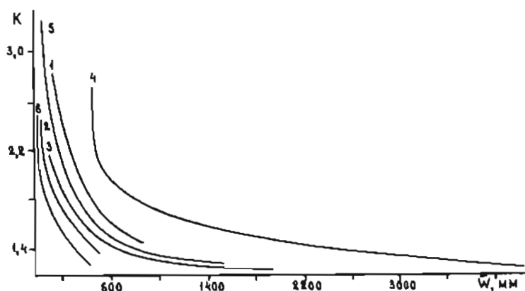
Рис. 16.2. Связь коэффициентов K отношения максимальных снегозапасов 5%-ной обеспеченности к их норме W для разных климатических областей Западной Европы. Пояснения в тексте
