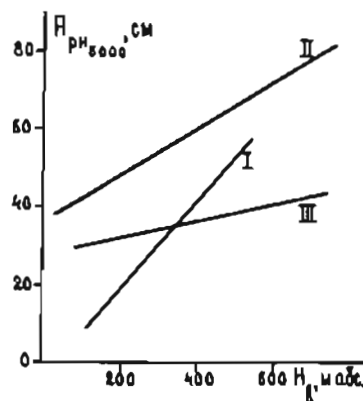
Рис.8.5. Связь средней многолетней толщины речных наледей, приведенной к площади водосбора 5000 \text{ км}^2 H_{пл, 5000} , с высотой местности H_{абс} в зоне БАМ. I-III - номера районов, границы которых приведены на рис.8.6
