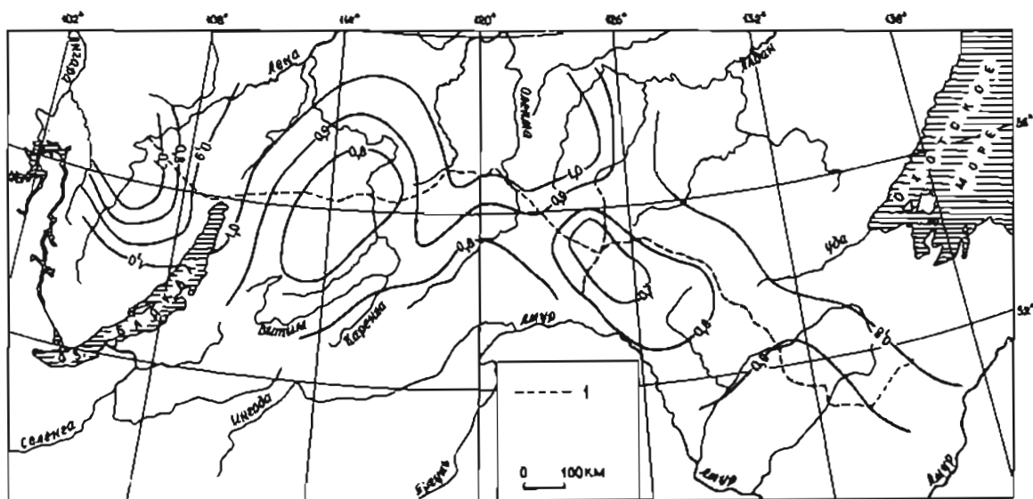
Рис.8.10. Вероятность P_r (частота) ежегодного образования речных наледей в зоне БАМ. 1-трасса БАМ
