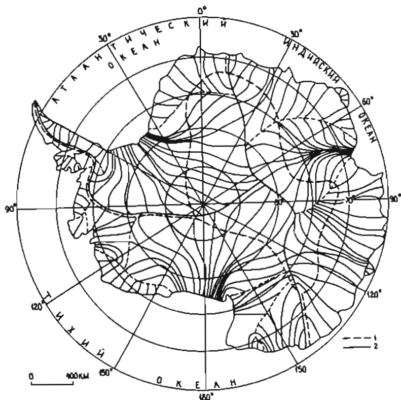
Рис. 12.1. Положение ледоразделов (1) и влагоразделов (2) трех океанов в Антарктиде
