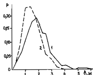
Рис.11.3. Распределение вероятностей P высот h торосов в Северном Ледовитом океане в апреле-мае по данным измерений: 1 - многолетние льды, 2 - однолетние льды
