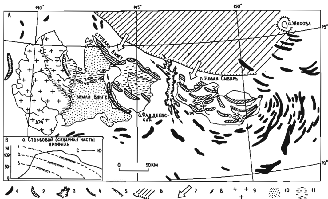
Рис.13.2. Ледниковые формы рельефа района Новосибирских островов (Гроссвальд, 1988б): А - гляцигеоморфологическая схема островов и окружающего шельфа, Б - положение "ярусных" долин на о. Столбовой: 1 - подводные гряды, 2 - дислокационные гряды на суше, 3 - туннельные долины, 4 - эрозионный уступ, 5 - "ярусные" долины, 6 - экзарационная депрессия на шельфе, 7 - направление движения льда, 8 - направления течения талой воды, 9 - коренные (скальные) породы, 10 - песчаные поверхности заандров, 11 - заболоченные участки
