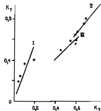
Рис. 9.3. Зависимость коэффициента стока талых вод K_t от коэффициента общего стока K_g в разных районах Канады: I - Саскачеван, II - Квебек-север, III - Квебек-юг
