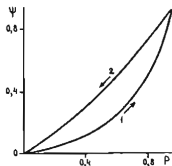
Рис.8.7. Связь относительных значений объема \Psi и площади P наледей подземных вод в холодный (1) и теплый (2) периоды года по средним многолетним данным
