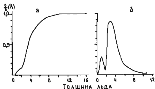
Рис.11.1. Интегральная функция распределения f(h) (а) и плотность вероятности (б) осадки морских льдов в центральной части моря Бофорта
