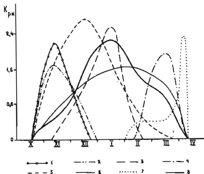
Рис. 8.9. Ход модульных коэффициентов питания речных наледей на территории юга Восточной Сибири (по материалам В.В.Кравченко, 1983). 1 - наледи при снежных нагрузках на ледяной покров, 2 - наледи при стеснении русла шугой, 3 - наледи при нарастании ледяного покрова, 4 - наледи при увеличении водности, 5 - наледи при промерзании подруслового потока, 6 - ключевые наледи, 7 - наледи талых снеговых вод, 8 - наледи всех видов вместе
