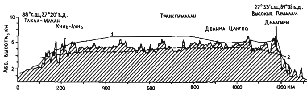
Рис.13.5. Реконструкция позднелайстоценового Центрально-Азиатского ледникового щита. По М.Куле (Kuhle, 1988). 1 - поверхность ледника, 2 - климатическая снеговая линия
