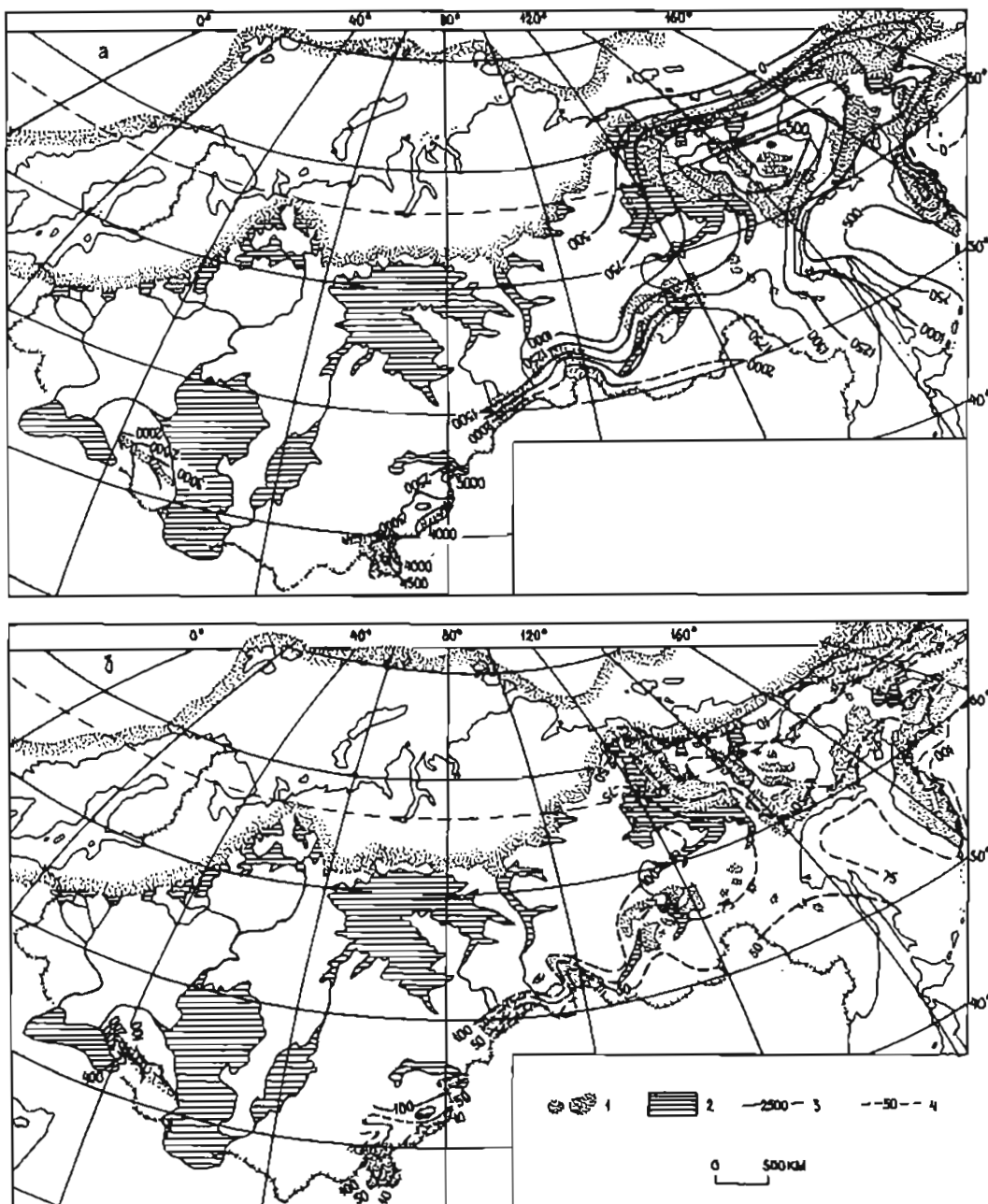
Рис.13.4. Высоты границы питания (а) и аккумуляция на этой высоте (б) у плейстоценовых ледников в горах на территории бывшего СССР. Реконструкцию выполнила Л.Н.Глебова. 1 - ледниковые щиты и горно-покровные комплексы, 2 - пресноводные бассейны, 3 - изохионы и их высота в м, 4 - изолинии аккумуляции (г/см 2 ), рассчитанной при допущении о снижении средней летней температуры на 7° относительно современной
