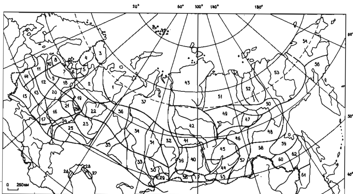
Рис.10.2. Районы однородного замерзания и вскрытия рек
