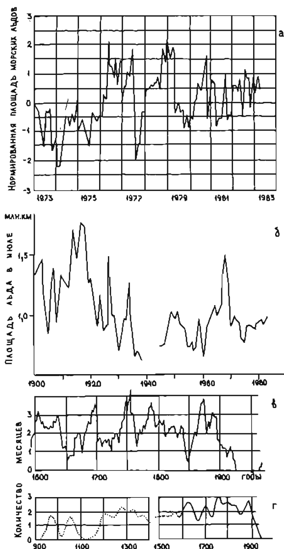
Рис. 11.4. Площадь морских льдов в Северном полушарии (а), в Северо-Европейском бассейне (б) и продолжительность ледового сезона у побережья Исландии (в - 10-летняя скользящая средняя, г - 30-летняя скользящая средняя)
