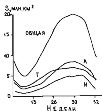
Рис.11.5. Средняя за 1973-1982 гг. площадь морских льдов S в Южном океане и его секторах: А - атлантическом, Т - тихоокеанском, И - индоокеанском
