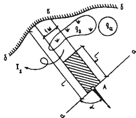
Рис.16.6. Схема к расчету переноса снега по методу балансов. Разъяснения в тексте
