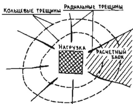
Рис.15.2. Типичное трещинообразование при сосредоточенной нагрузке на ледяной покров
