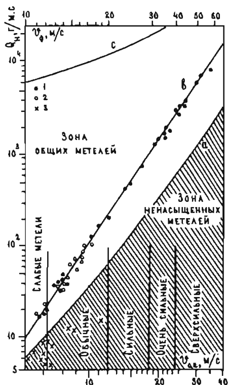
Рис.16.4. Зависимость общего твердого расхода снега Q_n при низовой метели от скорости ветра на высоте 0,2 м от поверхности земли V_{0,2} и на высоте флюгера V_{\phi} . 1 - измерения в большом аэродинамическом канале, 2 - полевые данные в условиях ненасыщенной метели, 3 - данные Д.Кобаяси (Kobayashi, 1972)
