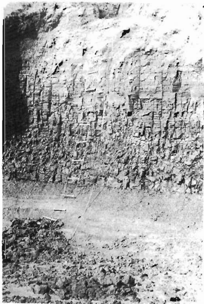
Рис. 8.4. Комплекс текстурообразующих и пластовых льдов. Оз. Ней-то на п-ве Ямал. Фото Г. И. Дубикова
