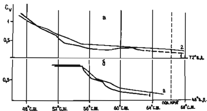
Рис. 9.5. Меридиональные профили изменений коэффициентов вариации C_v полного речного стока (1) и стока половодий (2); а - Европейская территория бывшего СССР, б - Западно-Сибирская низменность
