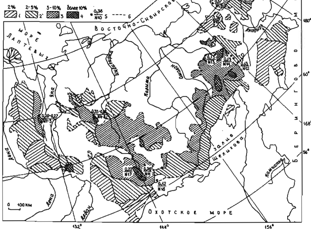
Рис.9.4. Карта коэффициента наледного стока рек Северо-Востока России, %: 1 - 2%, 2 - 2-5%, 3 - 5-10%, 4 - более 10%, 5 - местоположение бассейнов с аномально большой наледностью: в числителе значения коэффициента наледного стока, в знаменателе - номер бассейна по табл.9.3, 6 - граница массового распространения наледей подземных вод
