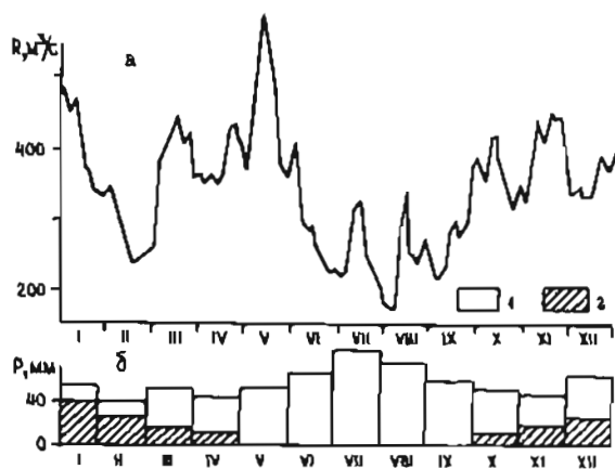
Рис.9.1. Гидрограф стока р.Одры в Польше (а) и ход осадков по месяцам, 1978 г. (б) 1 - жидкие осадки, 2 - твердые осадки
