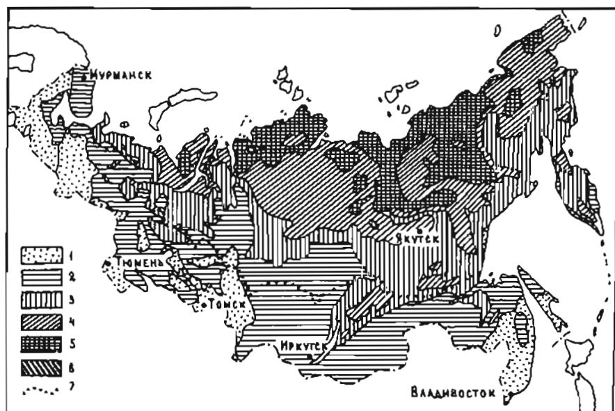
Рис.16.8. Влияние природных факторов Севера на стоимость гражданского строительства по С.А.Раките, 1983. Удорожание в процентах от нормы: 1 - 20-50, 2 - 51-100, 3 - 101-150, 4 - 151-200, 5 - 201-250, 6 - более 250, 7 - граница Крайнего Севера
