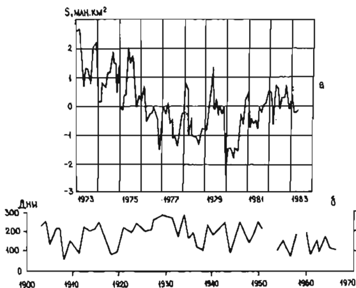
Рис. 11.6. Нормированная площадь морских льдов в Южном океане S (а) и продолжительность ледового сезона в районе Южно-Оркнейских островов (б)
