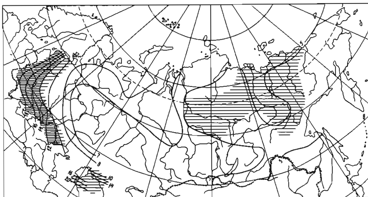
Рис.10.1. Средние квадратические отклонения от нормы сроков начала ледостава (а) и весеннего ледохода (б) на реках (в днях) и зоны значительной асимметрии распределения этих сроков: 1 - -0,3 > C_{\theta} > -0,6 ; 2 - C_{\theta} > 0,6 ; 3 - 0,3 < C_{\theta} < 0,6 ; 4 - C_{\theta} < 0,6
