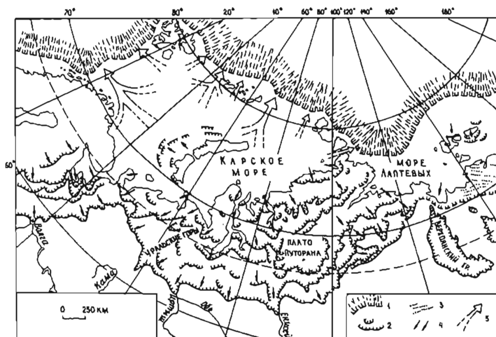
Рис.13.1. Главнейшие краевые образования и индикаторы движения последнего Евразийского ледникового покрова (Гросвальд, 1988а): 1 - материковый склон, 2 - краевые образования, 3 - гряды, разделяющие аласные долины на поверхности едочы, 4 - индикаторы движения льда, 5 - желоба-троги на шельфе
