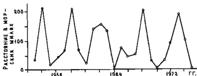
Рис.16.7. Расстояние от берега до границы плавучих льдов сплошностью 5 баллов и более на меридиане мыса Барроу в середине сентября. По У.Хиблеру (Hibler, 1980)
