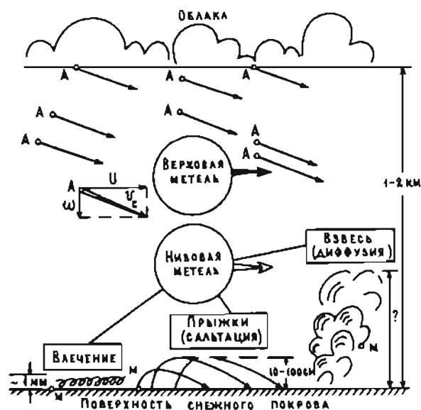
Рис.16.5. Виды метелей и способы движения метелевых частиц. Разъяснения в тексте
