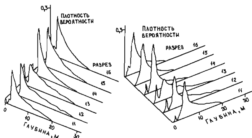
Рис.11.2. Плотность вероятности осадки морских льдов на 100-километровых профилях по меридиану 70^{\circ} з.д. от 85^{\circ} с.ш. (профиль 11) до Северного полюса (профиль 16)
