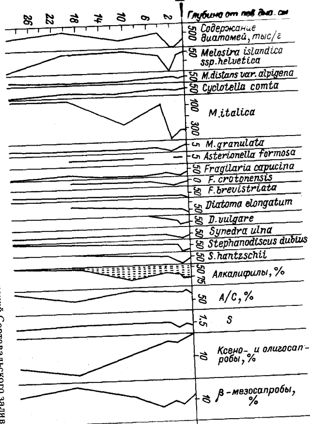
Рис. 17. Диатомовая диаграмма колонки донных отложений Соргавальского залива Ладожского озера.
