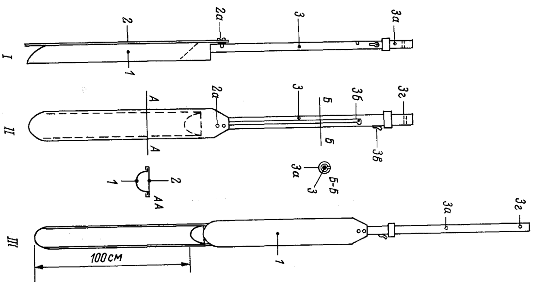
Рис. 7. Унифицированный бур Института горфа.
