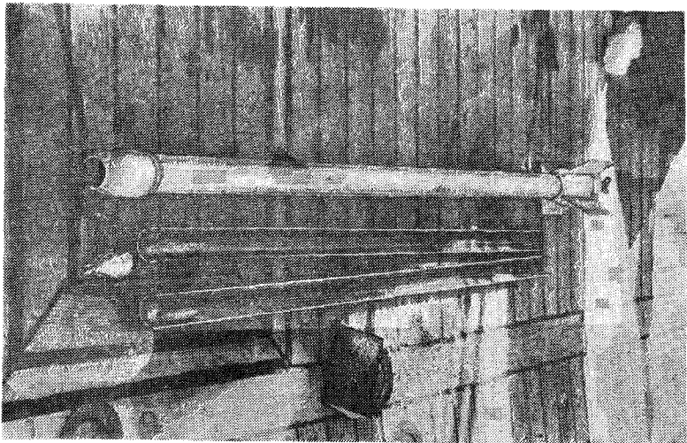
Рис. 8. Грунтовая трубка конструкции ГОИНА длиной 1,5 м (ГОИН-1.5), опускаемая на тросе.
