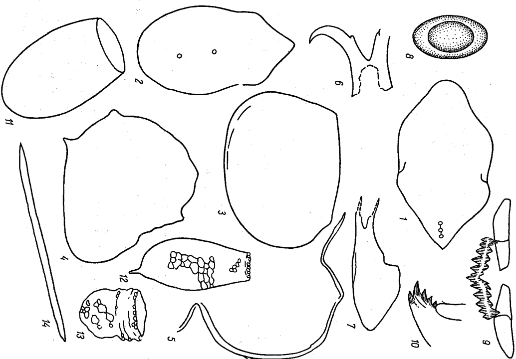
Рис. 18. Некоторые обычные остатки животных в грунте континентальных водоемов (увел. разное).
