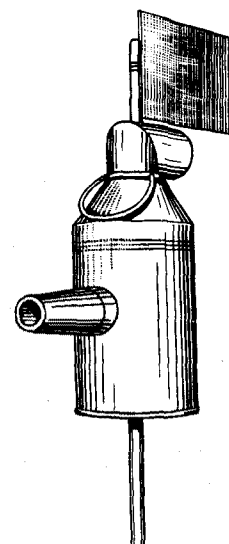
Рис. 11. Метелемер В. В. Кузнецова с коническим соплом.
