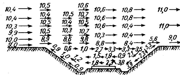
Рис. 7. Спектр скоростей воздушного потока в выемке в м/сек.
