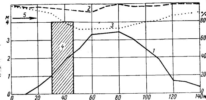
Рис. 19. Высота отложения снега (м) и скорость ветра (в процентах от полевой) на различных расстояниях от одиночной лесной полосы № 1 в 1950/51 г., по данным А. А. Комарова (19546).
