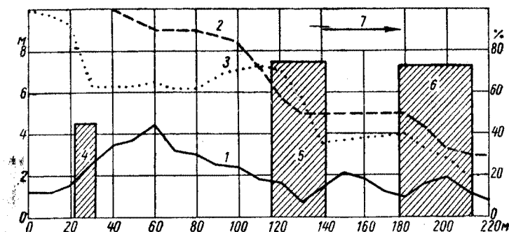
Рис. 20. Высота снега (м) и скорость ветра (в процентах от полевой) на опытном участке № 1 снегозащитных лесонасаждений Томской ж. д. в 1952/53 г., по данным А. А. Комарова (19546).
