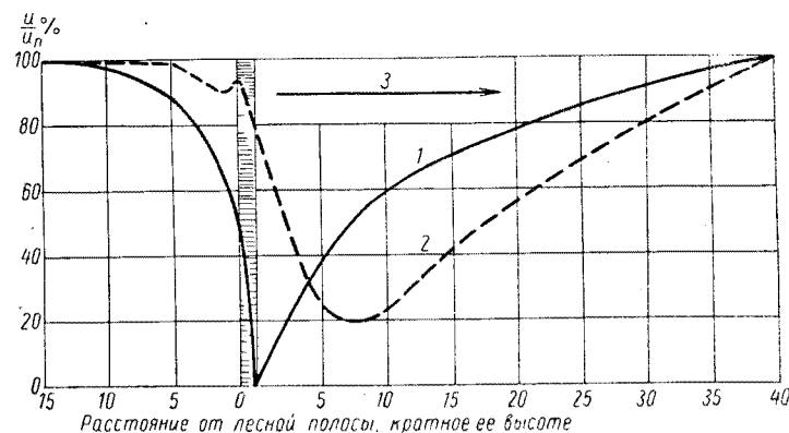
Рис. 17. Влияние узкой лесной полосы на снижение скорости ветра.
