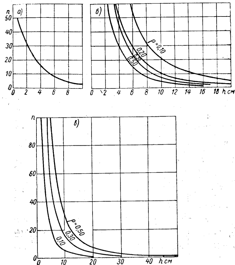
Рис. 27. Число промерных точек n , необходимых для того, чтобы на однородной площадке измерить высоту снега с точностью \pm 5\% (а), плотность снега с точностью \pm 5\% (б), плотность снега с ошибкой \pm 0,01 г/см 3 (в).
