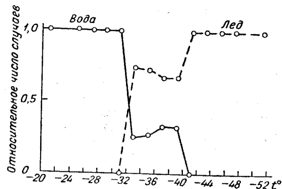
Рис. 1. Образование конденсированных частиц в пересыщенном водяном паре при быстром (близком к адиабатическому) разряжении влажного воздуха (по Л. Г. Качурину).
