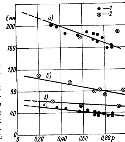
Рис. 22. Запас воды в снежном покрове к началу таяния ( E мм) в хвойном лесу в зависимости от полноты насаждения ( p ) по данным наблюдений на Валдае.
