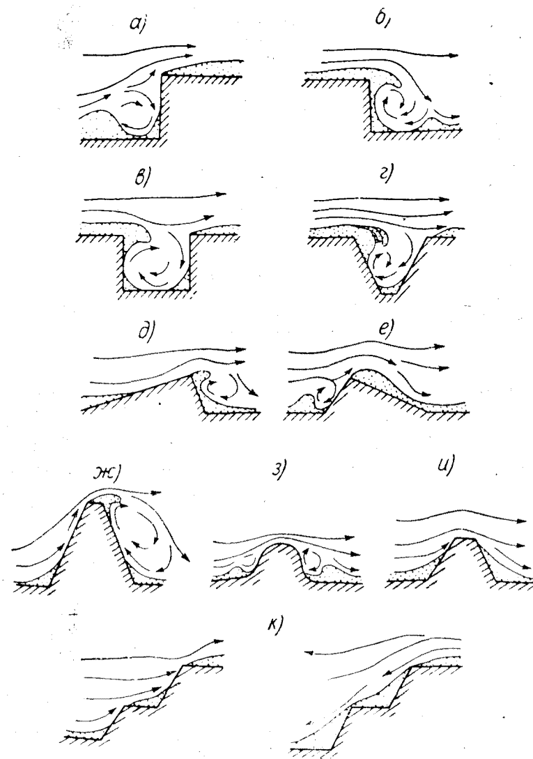
Рис. 15. Схема отложения снега на различных элементах рельефа (по Г. Д. Рихтеру).
