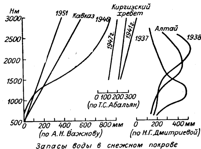
Рис. 25. Кривые изменения снегозапасов по высоте H , близкие к средним многолетним и за отдельные характерные годы для Кавказа, Киргизского хребта и Алтая.
