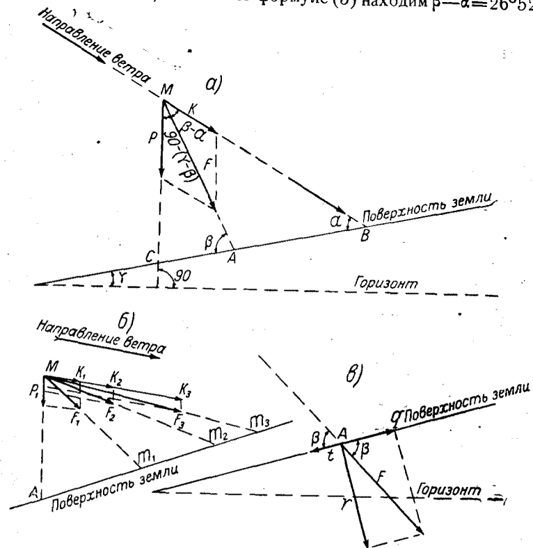
Рис. 8. Равнодействующая F двух сил P и K (веса снежинки и силы ветра), под влиянием которых происходит перемещение снежной частицы M .
