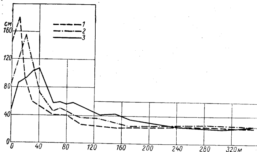
Рис. 18. Высота снега (см) на различных расстояниях от лесных полос (м) в зависимости от их конструкции (Никитин и Минин, 1949). Лесная полоса: 1 — плотная, 2 — ажурная, 3 — продуваемая.
