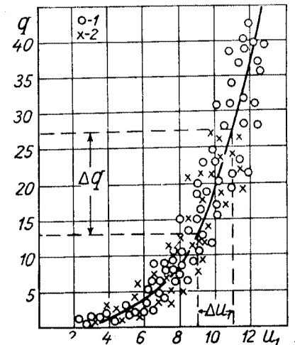
Рис. 13. Зависимость общей интенсивности переноса снега от скорости ветра по данным метелемерных наблюдений (Колмаров, 1954а). 1 — на открытой площадке, 2 — за преградами.
