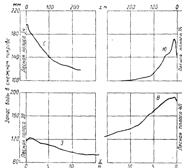
Рис. 24. Убыль среднего по маршруту запаса воды в снеге в зависимости от его длины (расстояния \frac{B}{2} + x от середины лесной полосы по направлению к середине поля Б-2) по данным снегомерной съемки по постоянным рейкам 13/III 1953 г. С — северный маршрут поля Б-2, Ю — южный, З — западный и В — восточный, Н — высота лесной полосы, x — расстояние от края полосы.
