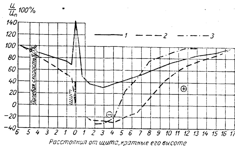
Рис. 16. Скорость ветра у плоских преград по данным анемометрических съемок и продувания моделей в аэродинамической трубе (Савиных и Дюнин, 1954).
