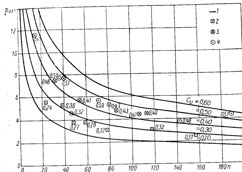
Рис. 29. Ошибка определения среднего запаса воды в снежном покрове, обеспеченная на 0,67 ( p ), в зависимости от коэффициента вариации запаса C_v и числа промерных точек n .
