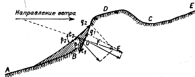
Рис. 14. Изменение угла \beta с увеличением толщины слоя отложения снега.
