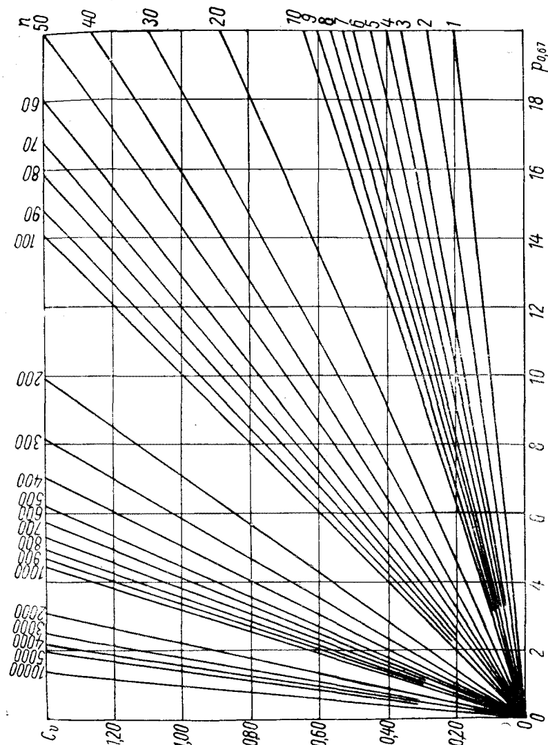
Рис. 28. Число промерных точек n , вычисленное по формуле (73), в зависимости от коэффициента вариации C_v и заданной точности результата измерения, обеспеченной на 0,67 ( p_{0,67} ).
