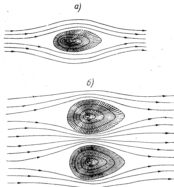
Рис. 4. Схема линий тока в случае движения воздушного потока.
