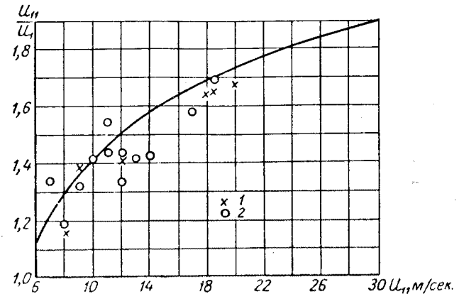
Рис. 12. Отношение скоростей ветра на уровнях 11 и 1 м \left(\frac{u_{11}}{u_1}\right) в зависимости от скорости ветра u_{11} .
