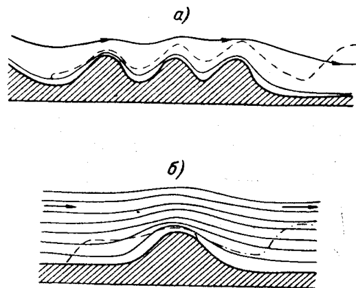
Рис. 2. Обтекание воздушным потоком возвышенностей, имеющих форму хребта. Пунктиром показана траектория движения воздушного шара, поднявшегося в низине (в левой части рисунков а и б).
