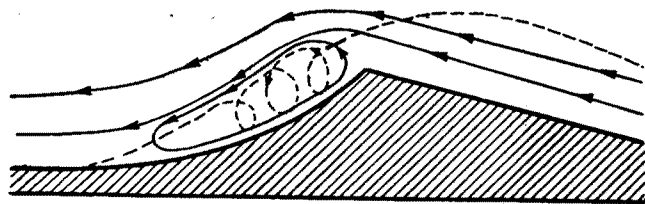
Рис. 3. Образование на подветренном склоне возвышенности кругового вихреобразного потока.
