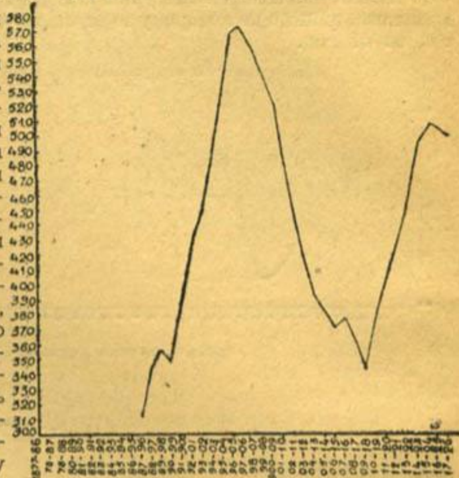
Саме. График десятилетних средних уровней Аму-Дарьи
