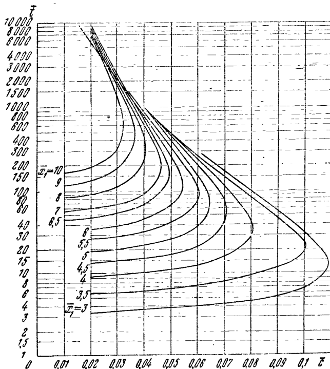
Рис. 28. График зависимости \bar{t} = f(\bar{C}, \bar{x}) для одиночного водозабора у реки при подтягивании соленых вод со стороны берега
