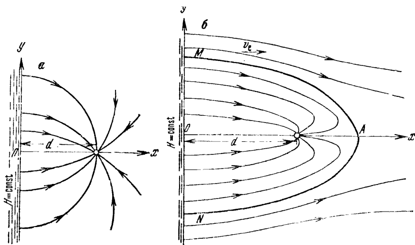
Рис. 6. Схема линий тока в полуограниченном пласте: контуром постоянного напора в условиях бассейна и естественного потока подземных вод, направленного от контура
