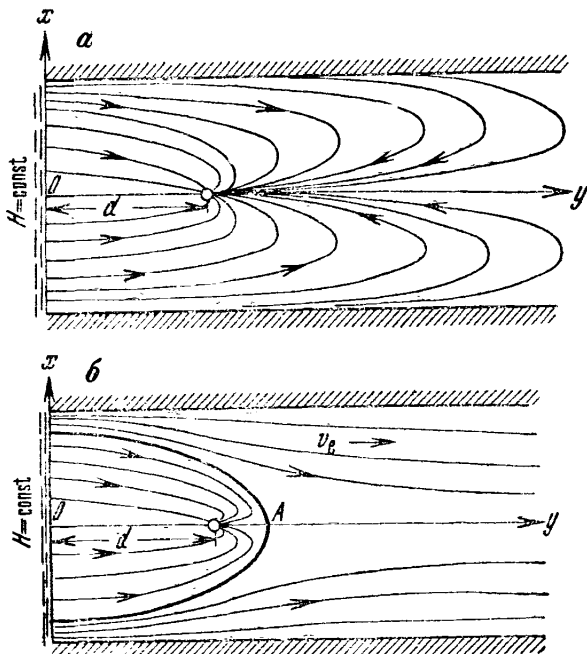
Рис. 12. Схема линий тока в пласте-полосе с внутренним контуром постоянного напора в условиях бассейна a и потока b
