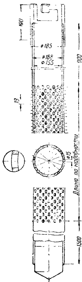
рис. 25. Дырчатый металлический фильтр с круглыми отверстиями
