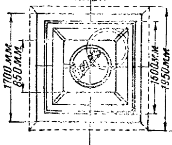
Рис. 53. Донный ящик
