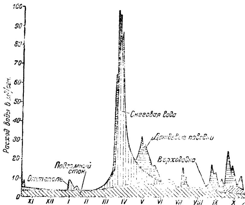
Рис. 7. Годограф р. Ижоры (по В. С. Советову)
