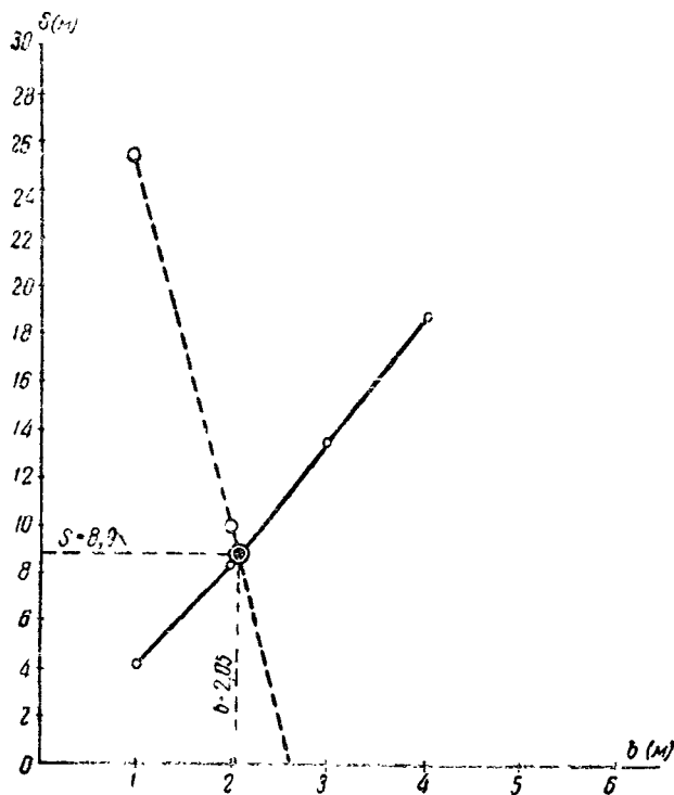
Рис. 67. Схема определения допустимого понижения уровня воды при откачке из бесфильтровой скважины и глубины водоприемной каверны [— по формуле (87), ... по формуле (92)]
