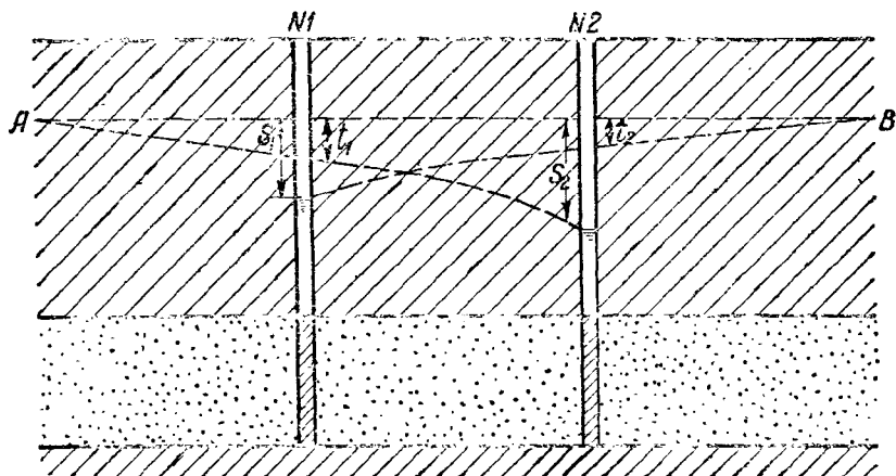
Рис. 41. Схема влияния откачки из сызжиг. АВ — пьезометрический уровень воды до откачки
